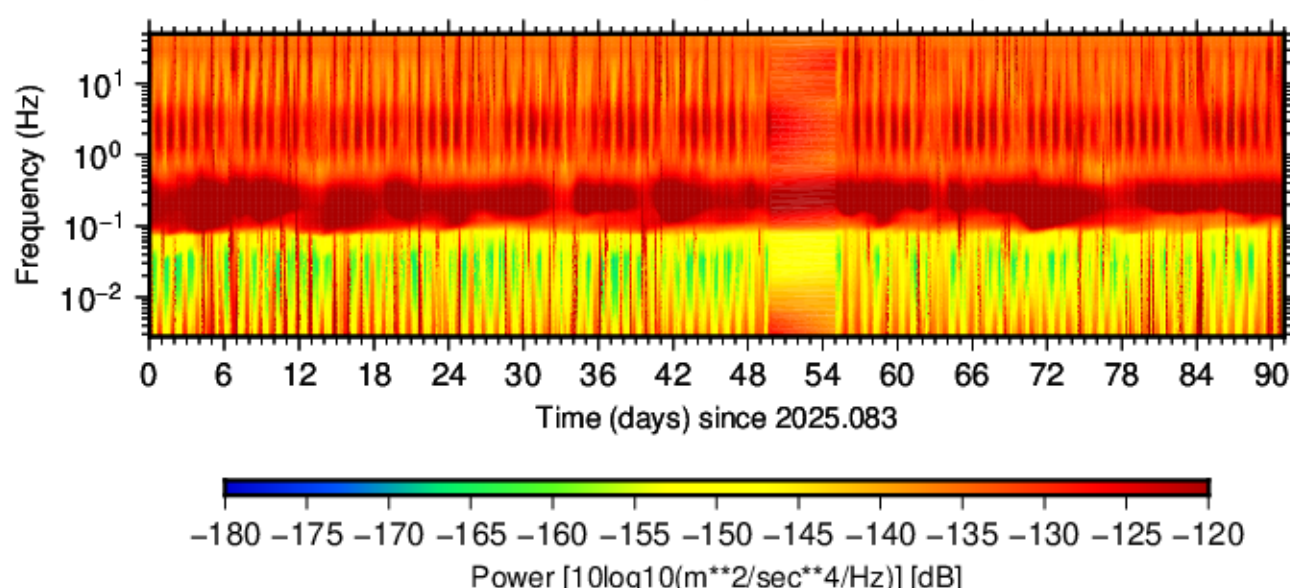
BK.MERC.HHN.00 (2025.083 - 2025.173)
