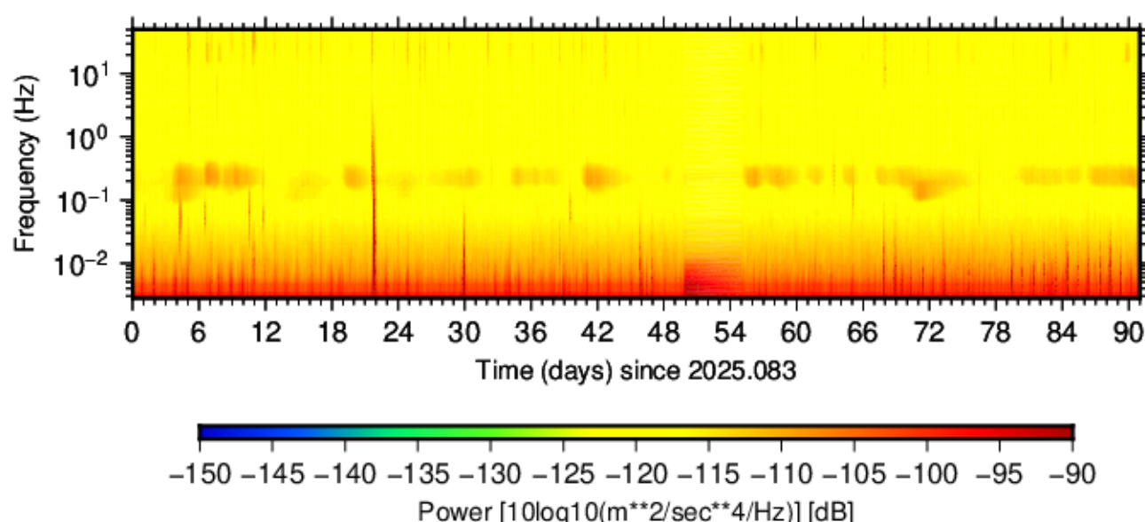
BK.MERC.HNE.00 (2025.083 - 2025.173)
