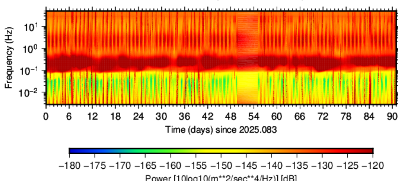
BK.MERC.HHE.00 (2025.083 - 2025.173)
