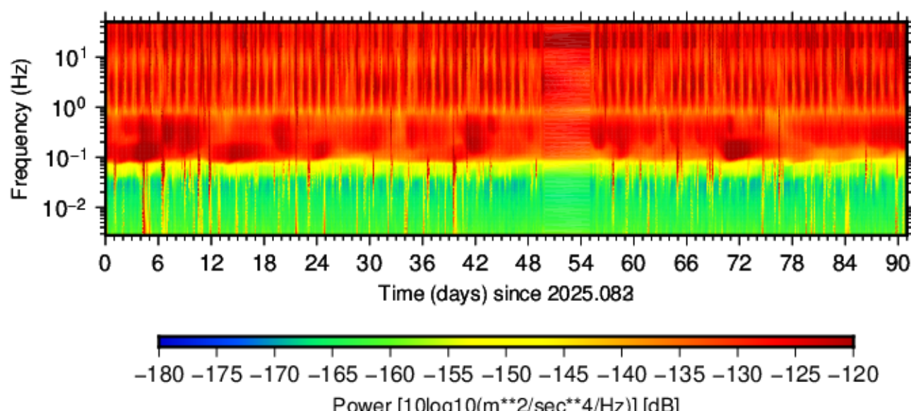
BK.MERC.HHZ.00 (2025.083 - 2025.173)
