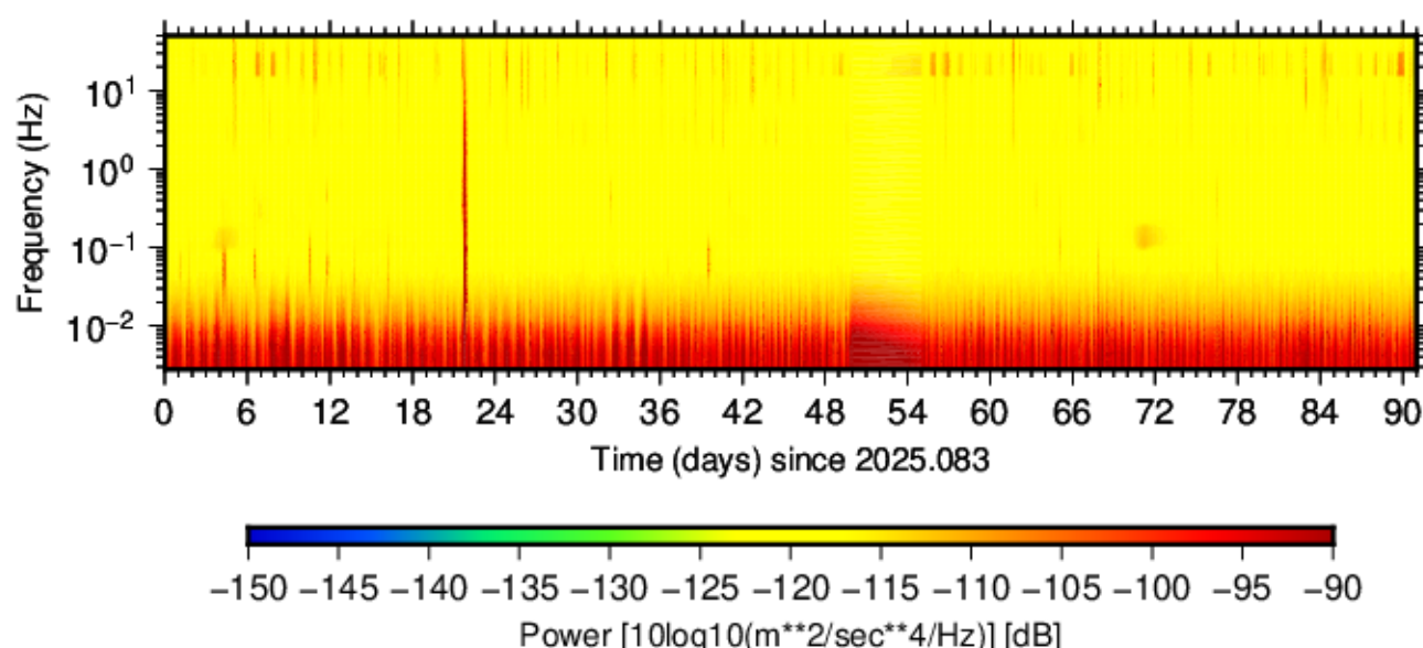
BK.MERC.HNZ.00 (2025.083 - 2025.173)
