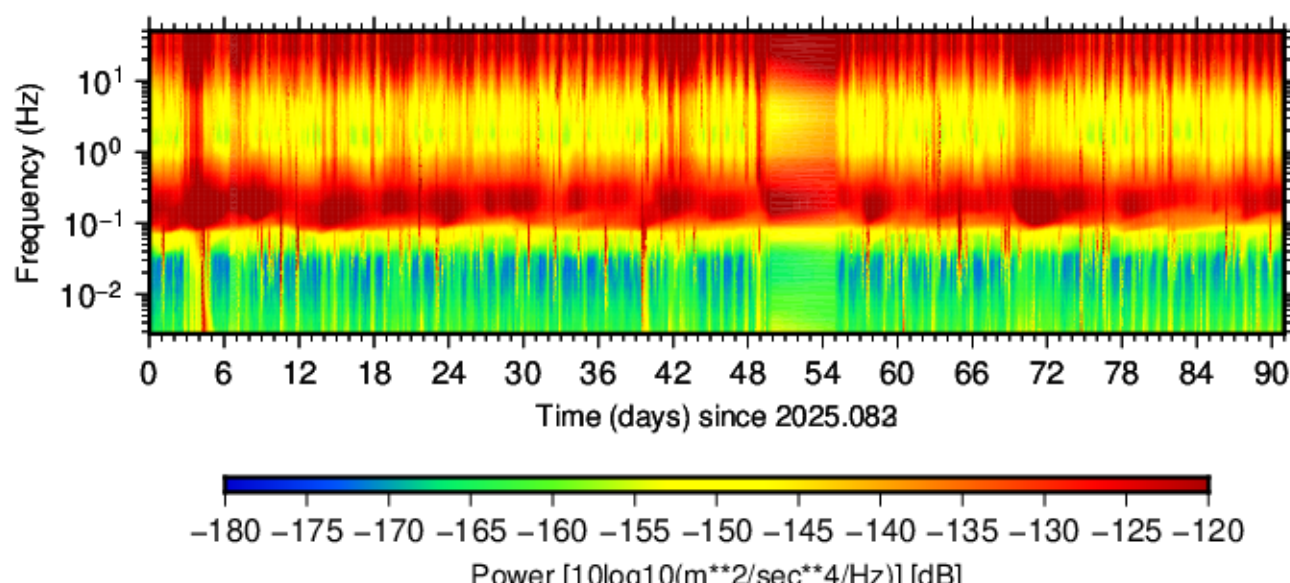
BK.LTIB.HHZ.00 (2025.083 - 2025.173)
