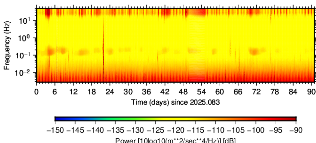
BK.LTIB.HNN.00 (2025.083 - 2025.173)
