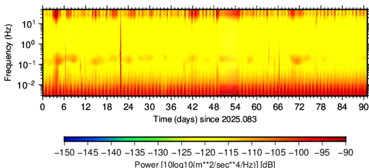
BK.LTIB.HNE.00 (2025.083 - 2025.173)
