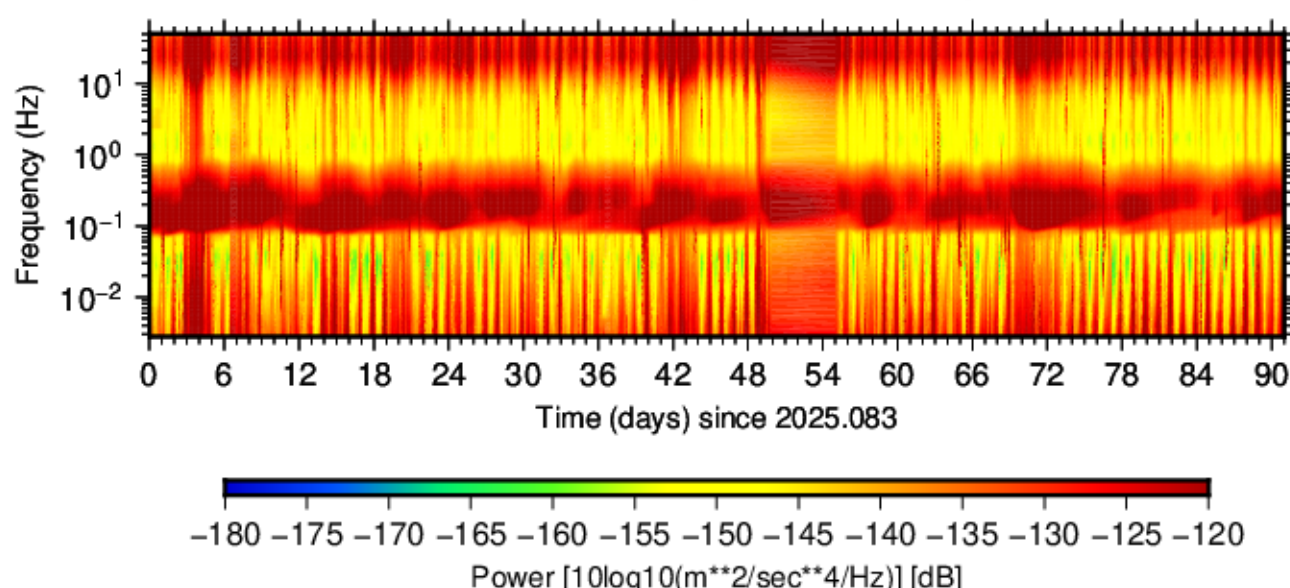
BK.LTIB.HHN.00 (2025.083 - 2025.173)
