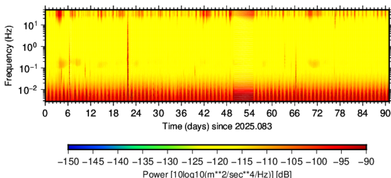
BK.LTIB.HNZ.00 (2025.083 - 2025.173)
