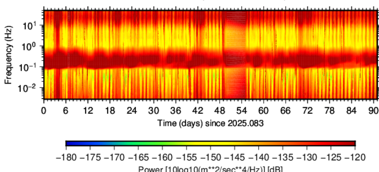
BK.LTIB.HHE.00 (2025.083 - 2025.173)
