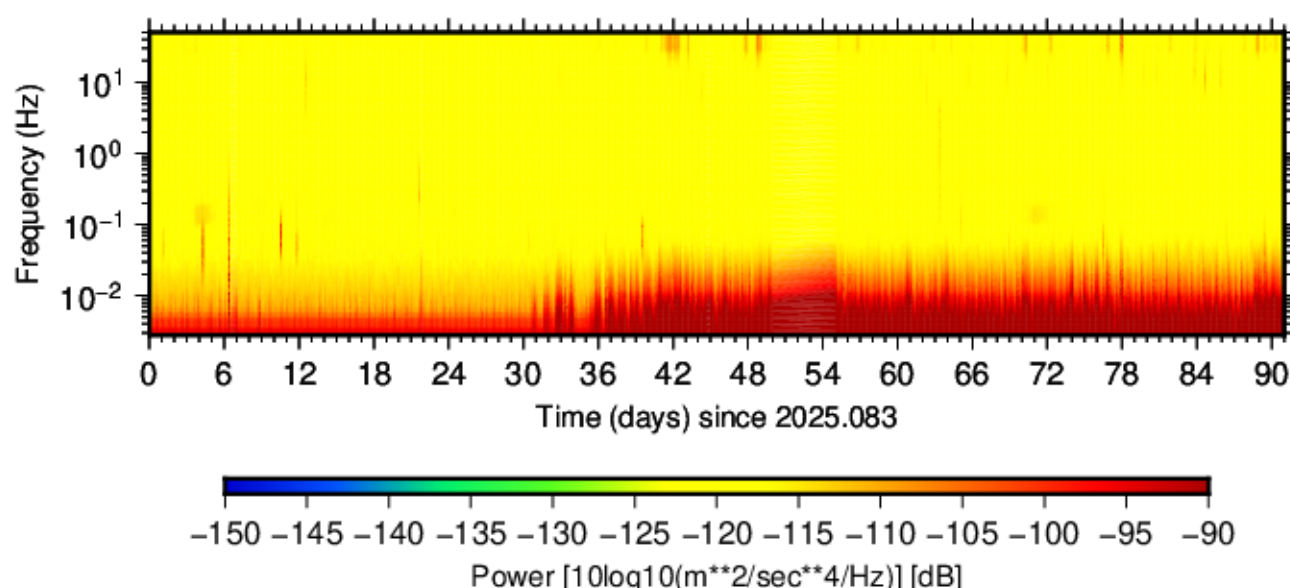
BK.LSIB.HNZ.00 (2025.083 - 2025.173)
