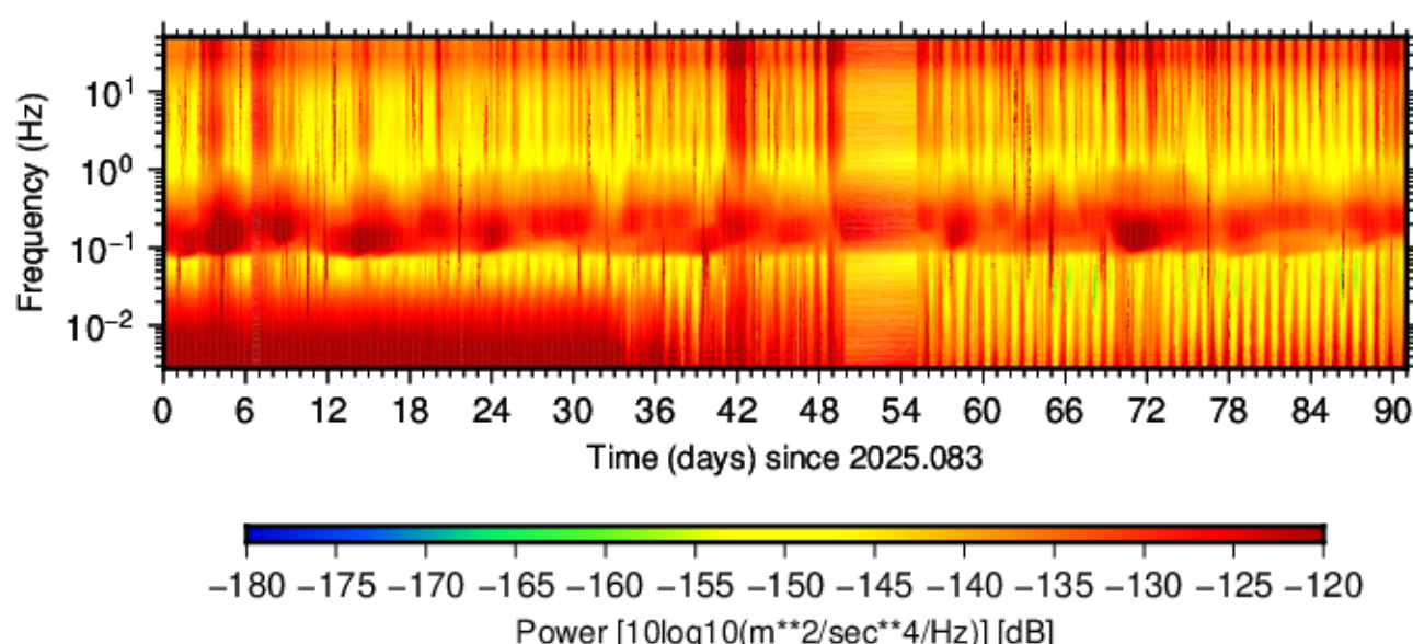
BK.LSIB.HHN.00 (2025.083 - 2025.173)
