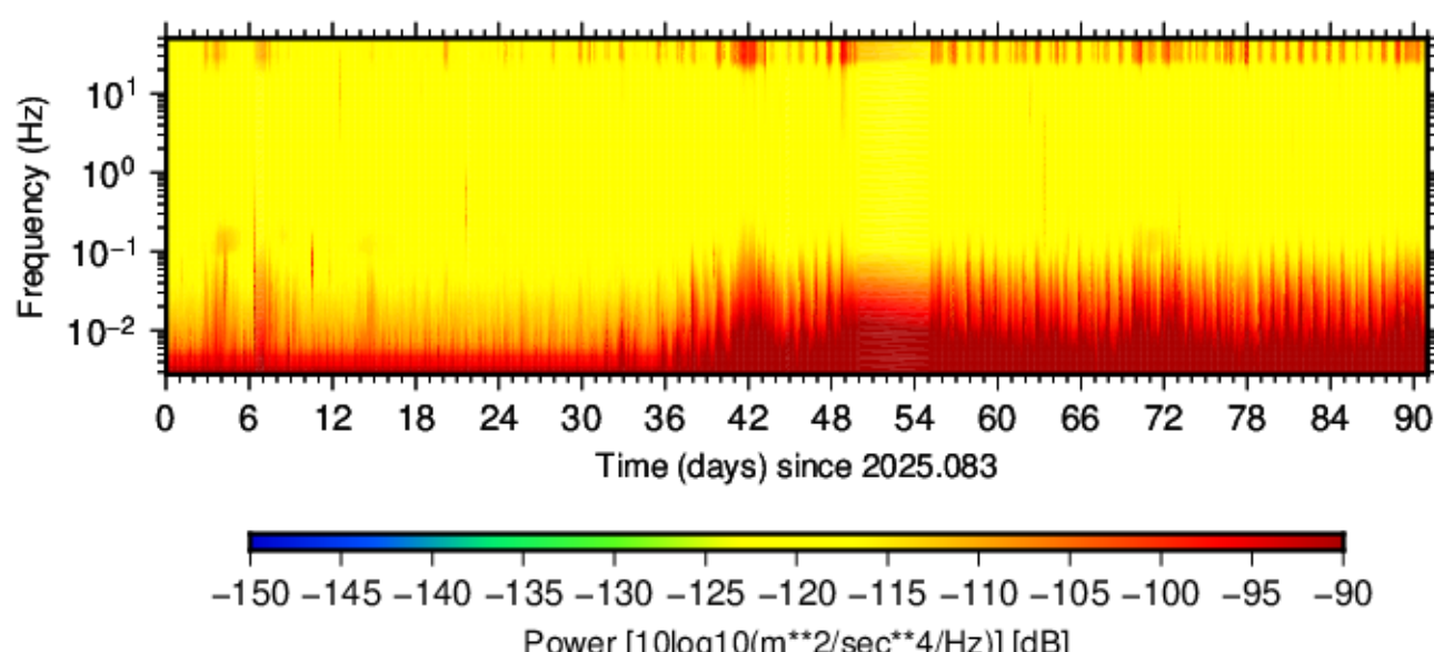
BK.LSIB.HNN.00 (2025.083 - 2025.173)
