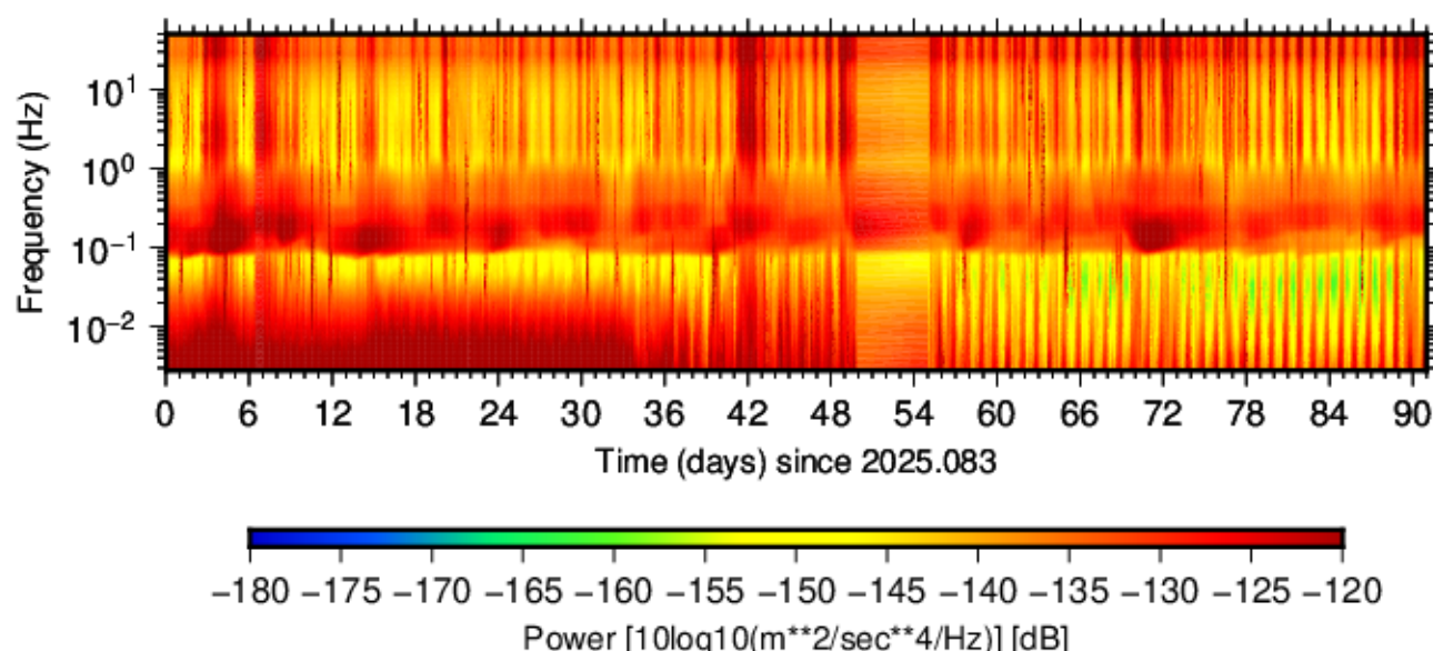
BK.LSIB.HHE.00 (2025.083 - 2025.173)
