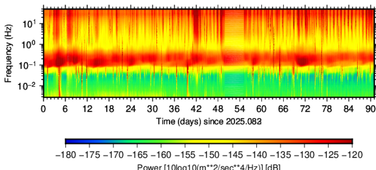
BK.LSIB.HHZ.00 (2025.083 - 2025.173)
