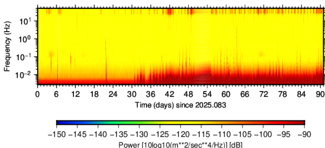
BK.LSIB.HNE.00 (2025.083 - 2025.173)
