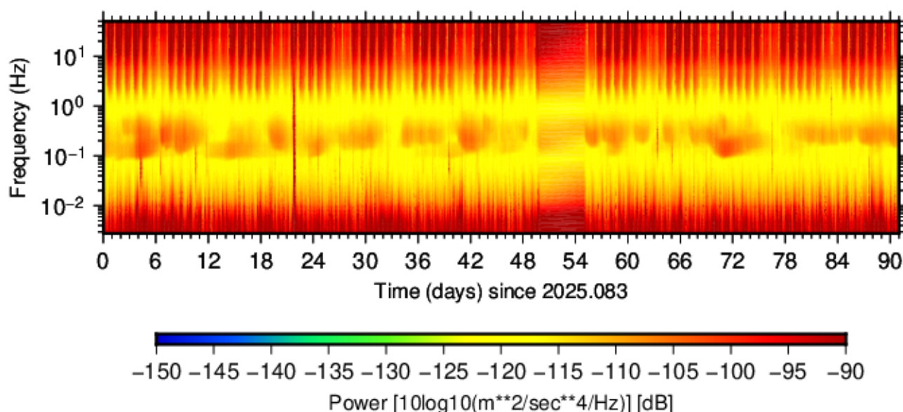
BK.LLNL.HNN.00 (2025.083 - 2025.173)
