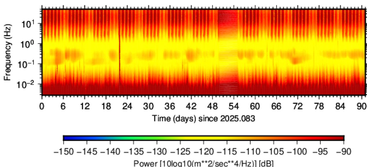
BK.LLNL.HNZ.00 (2025.083 - 2025.173)
