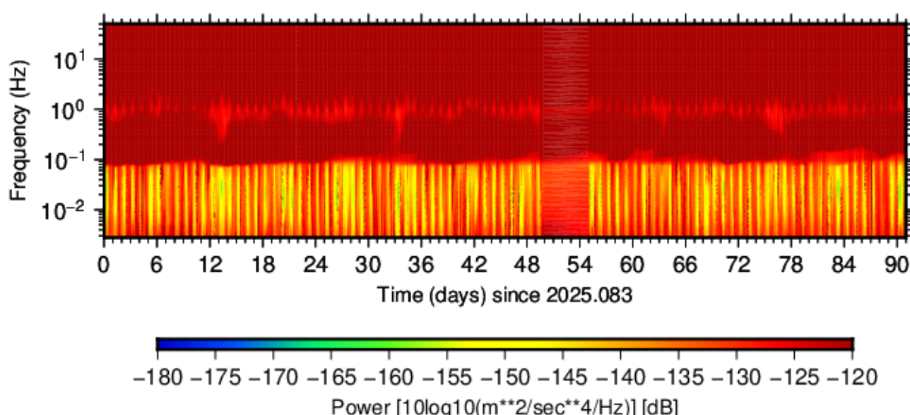
BK.LLNL.HHN.00 (2025.083 - 2025.173)
