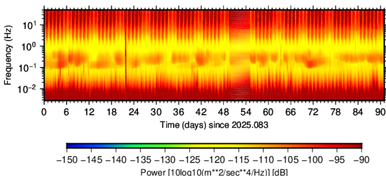
BK.LLNL.HNE.00 (2025.083 - 2025.173)
