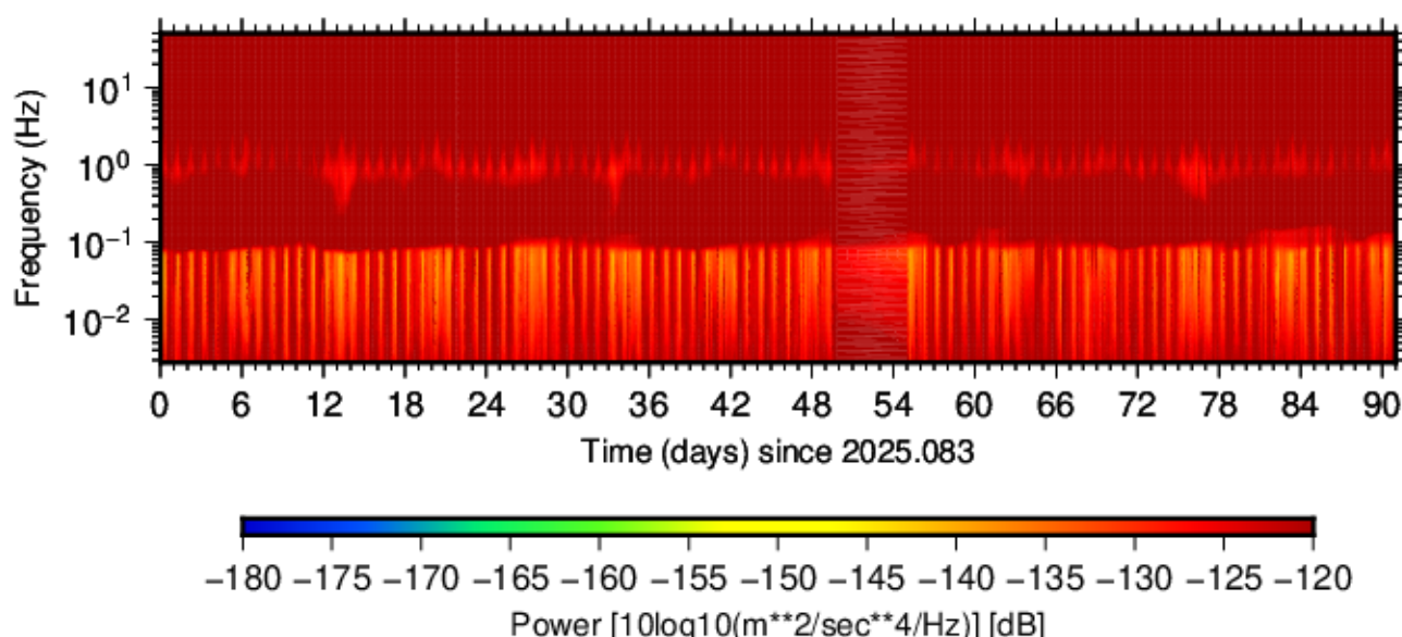
BK.LLNL.HHE.00 (2025.083 - 2025.173)
