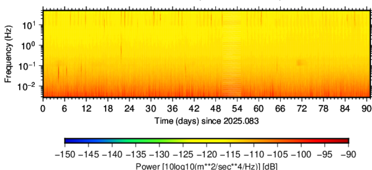
BK.LIND.HNZ.00 (2025.083 - 2025.173)
