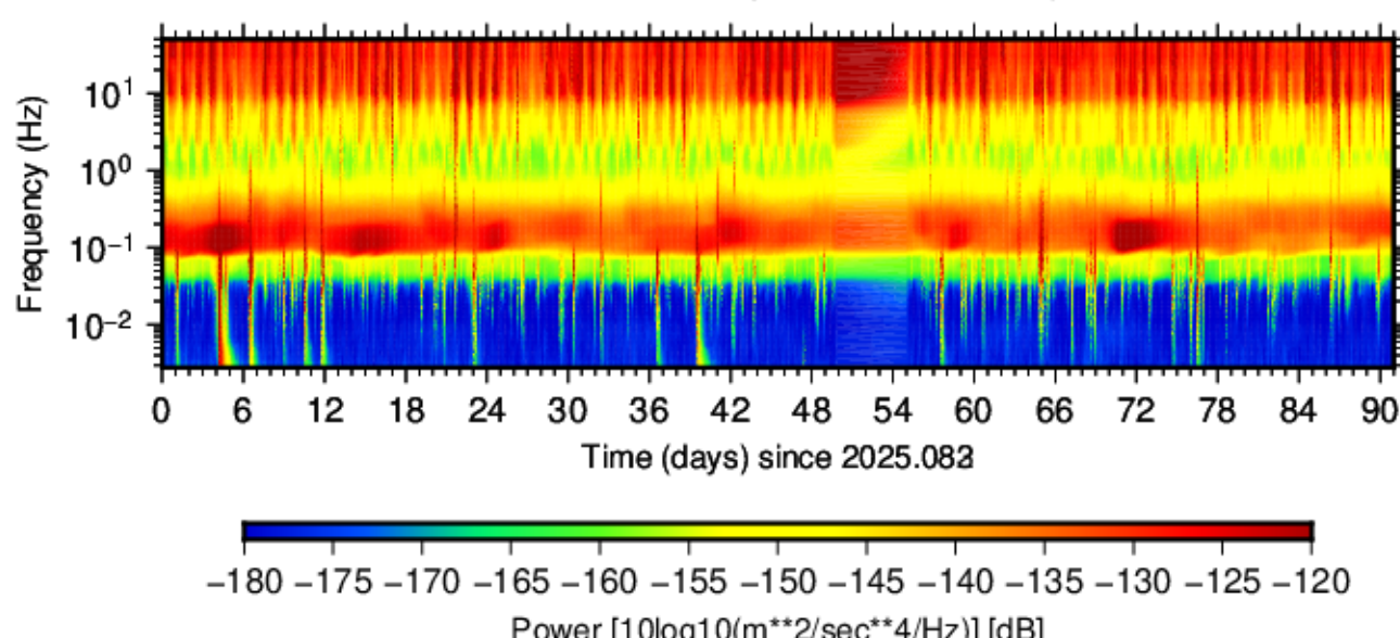
BK.LIND.HHZ.00 (2025.083 - 2025.173)
