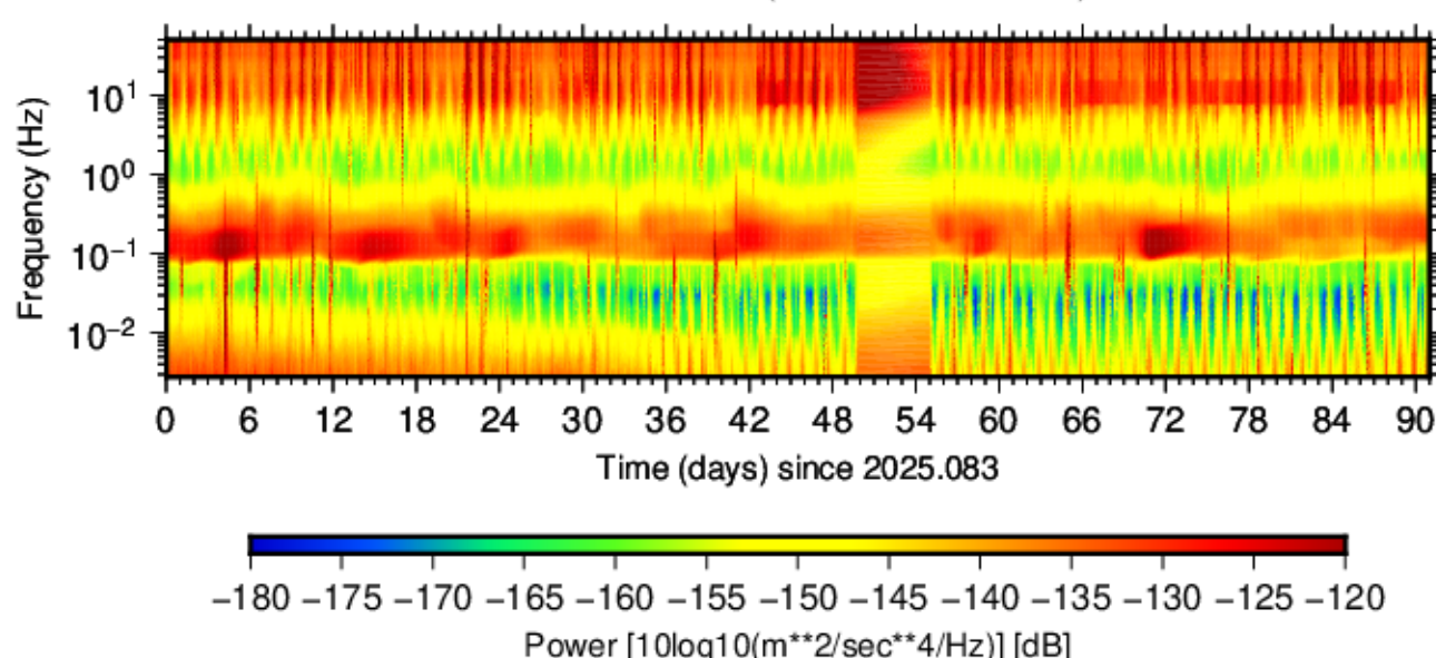
BK.LIND.HHE.00 (2025.083 - 2025.173)
