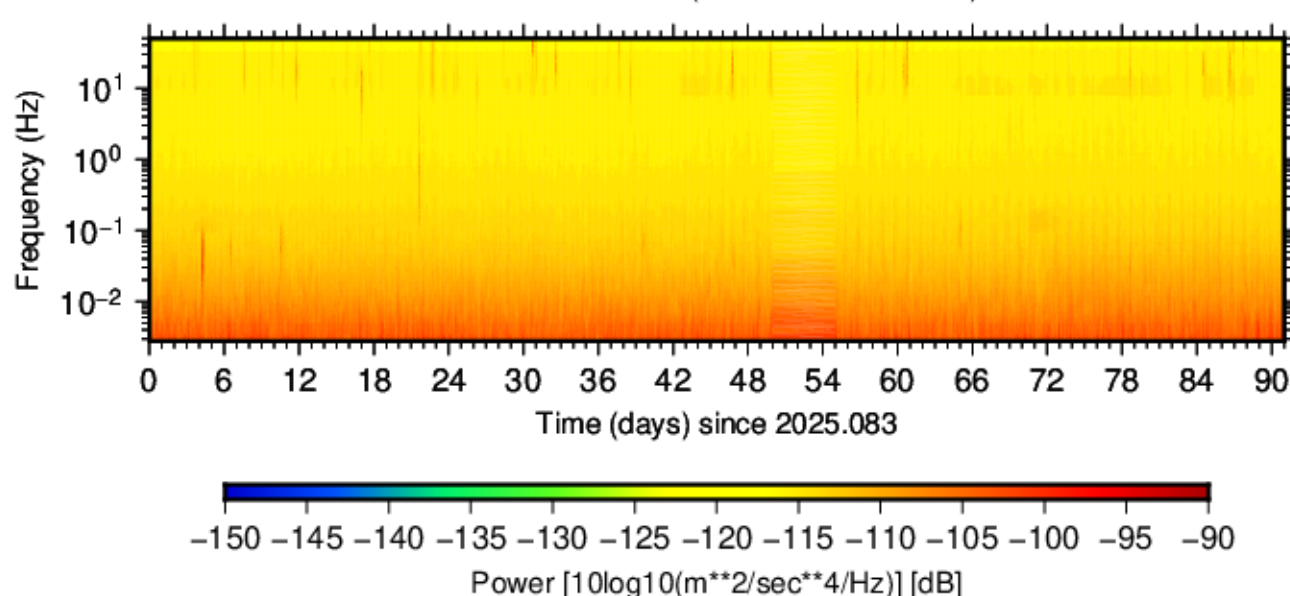
BK.LIND.HNN.00 (2025.083 - 2025.173)
