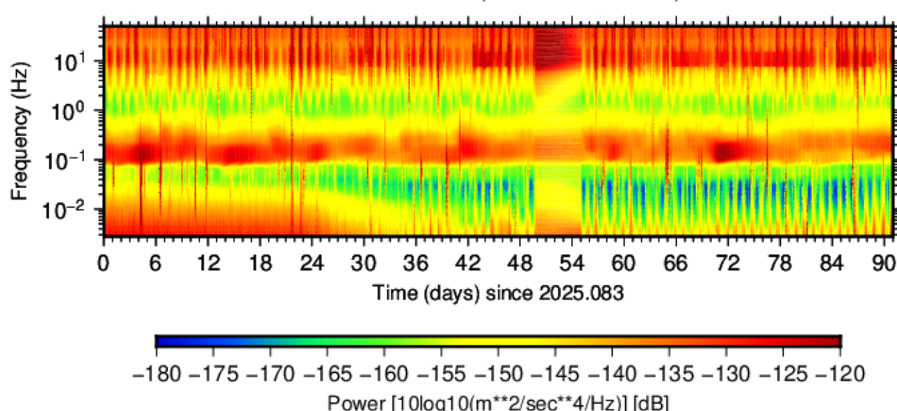
BK.LIND.HHN.00 (2025.083 - 2025.173)
