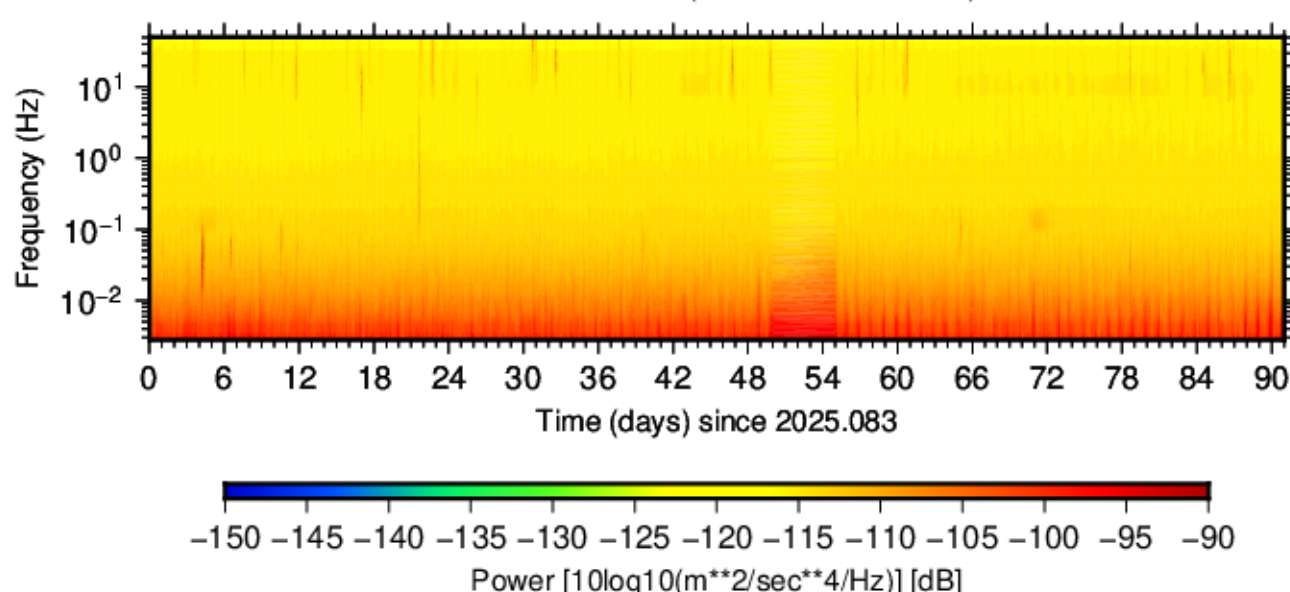
BK.LIND.HNE.00 (2025.083 - 2025.173)
