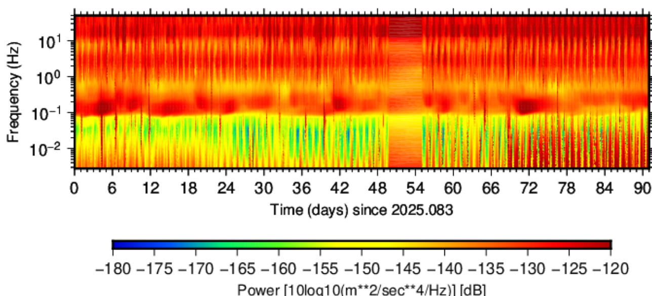
BK.LEGD.HHE.00 (2025.083 - 2025.173)
