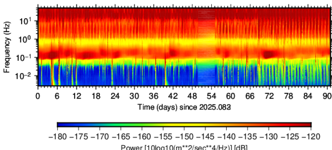
BK.LEGD.HHZ.00 (2025.083 - 2025.173)
