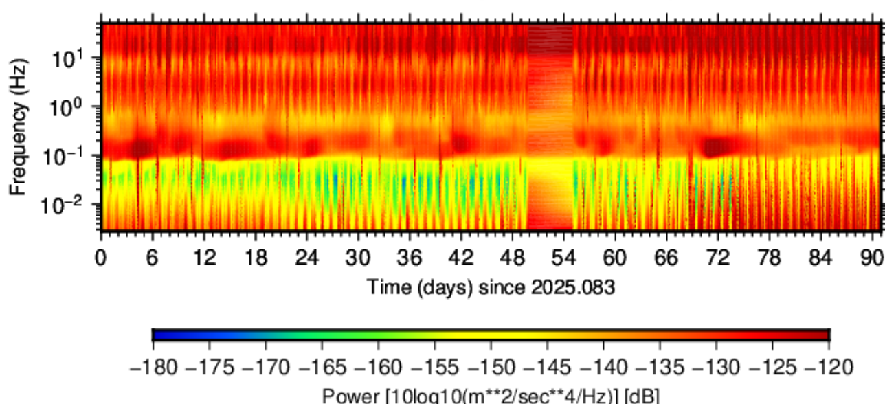
BK.LEGD.HHN.00 (2025.083 - 2025.173)
