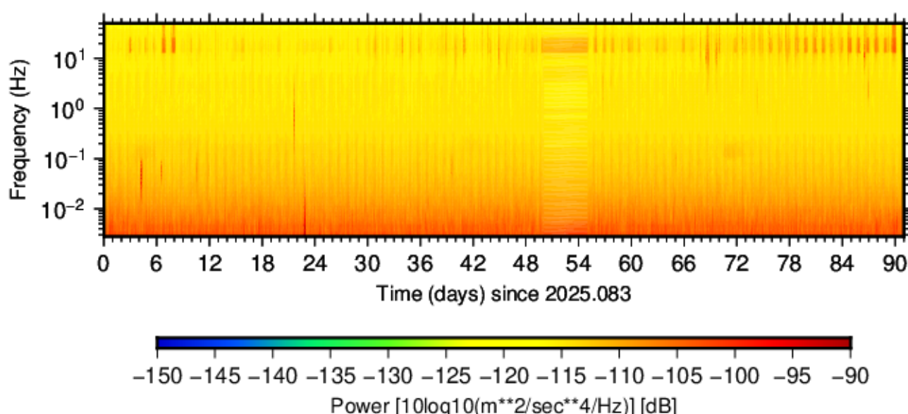
BK.LEGD.HNE.00 (2025.083 - 2025.173)
