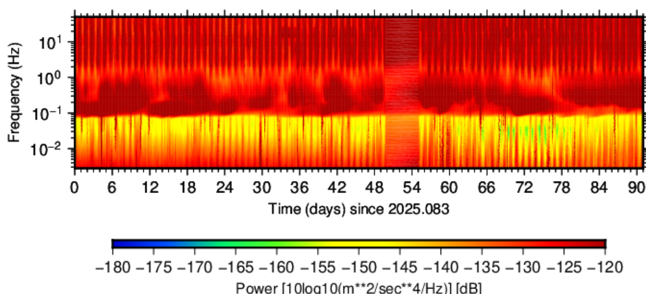
BK.LCUV.HHN.00 (2025.083 - 2025.173)
