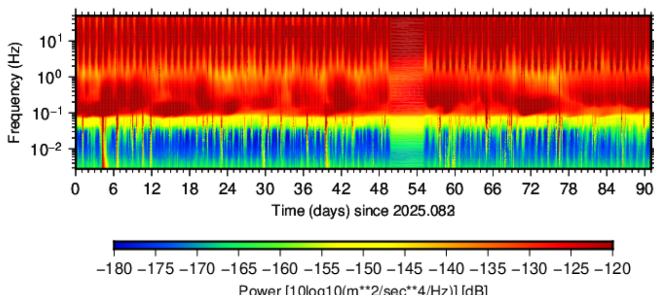
BK.LCUV.HHZ.00 (2025.083 - 2025.173)
