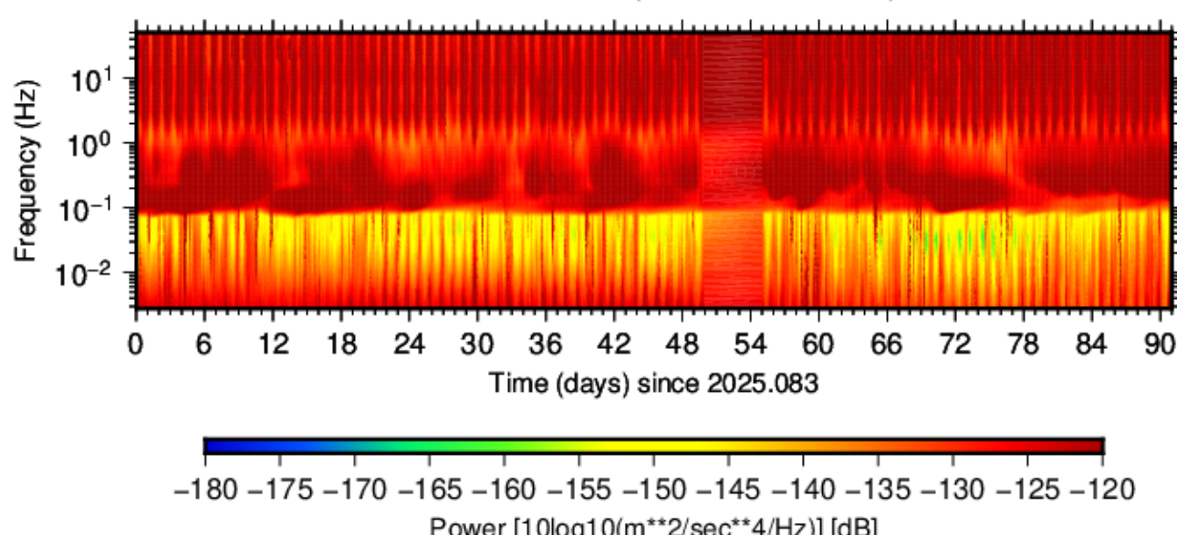
BK.LCUV.HHE.00 (2025.083 - 2025.173)
