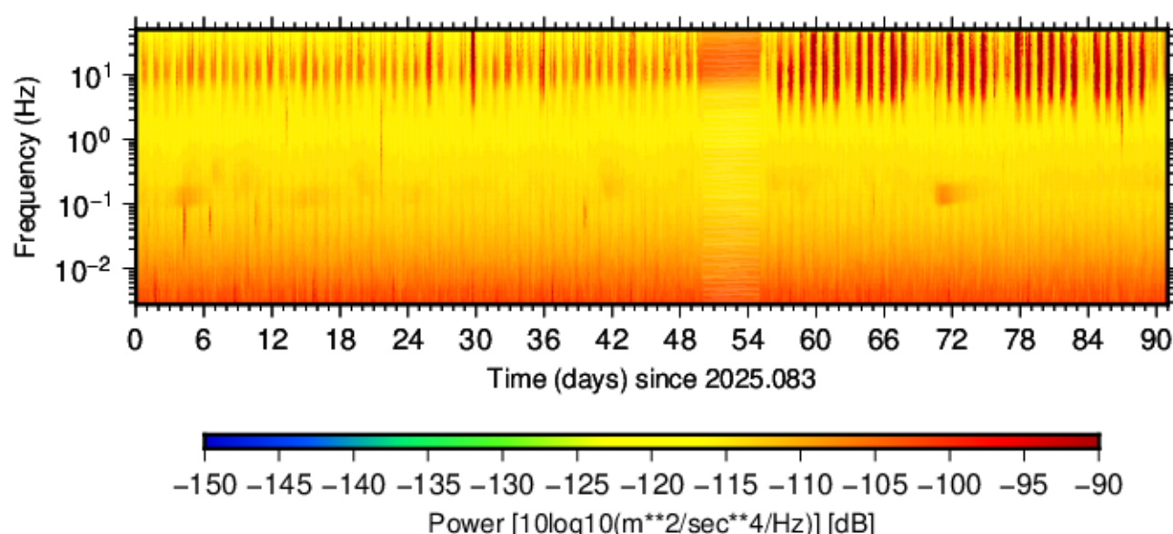
BK.LCUV.HNZ.00 (2025.083 - 2025.173)
