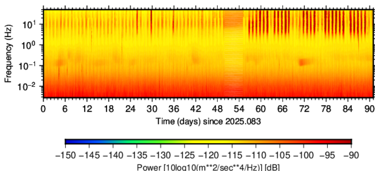
BK.LCUV.HNE.00 (2025.083 - 2025.173)
