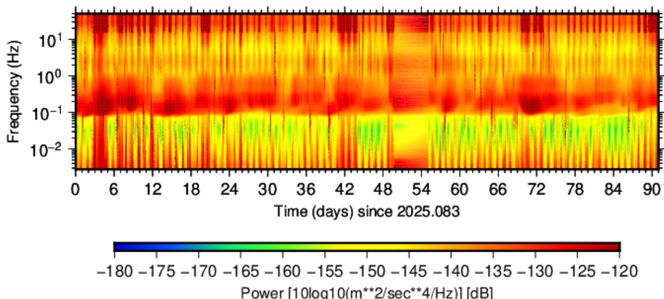
BK.LCOW.HHE.00 (2025.083 - 2025.173)
