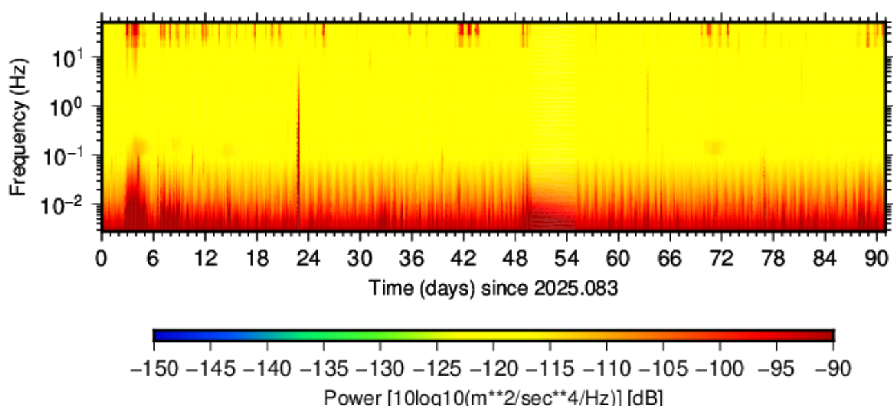
BK.LCOW.HNZ.00 (2025.083 - 2025.173)
