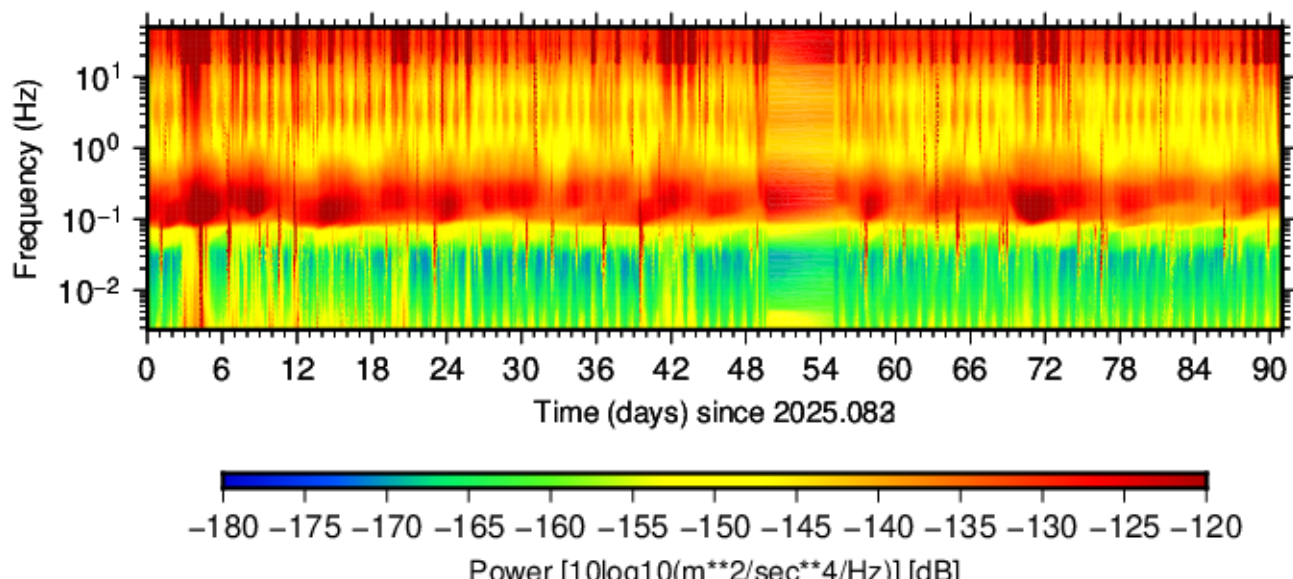
BK.LCOW.HHZ.00 (2025.083 - 2025.173)
