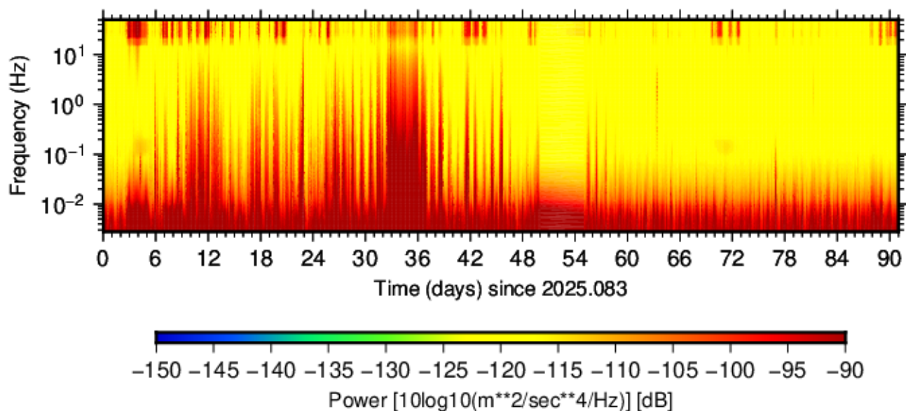
BK.LCOW.HNE.00 (2025.083 - 2025.173)
