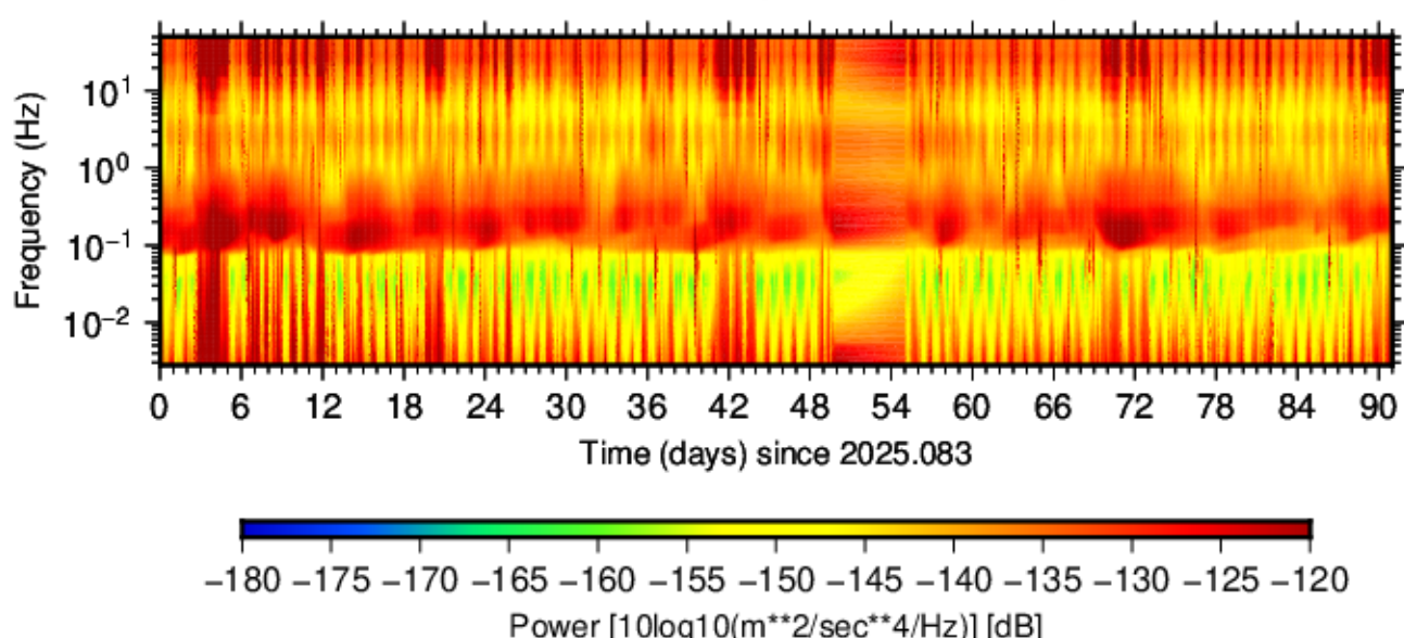
BK.LCOW.HHN.00 (2025.083 - 2025.173)
