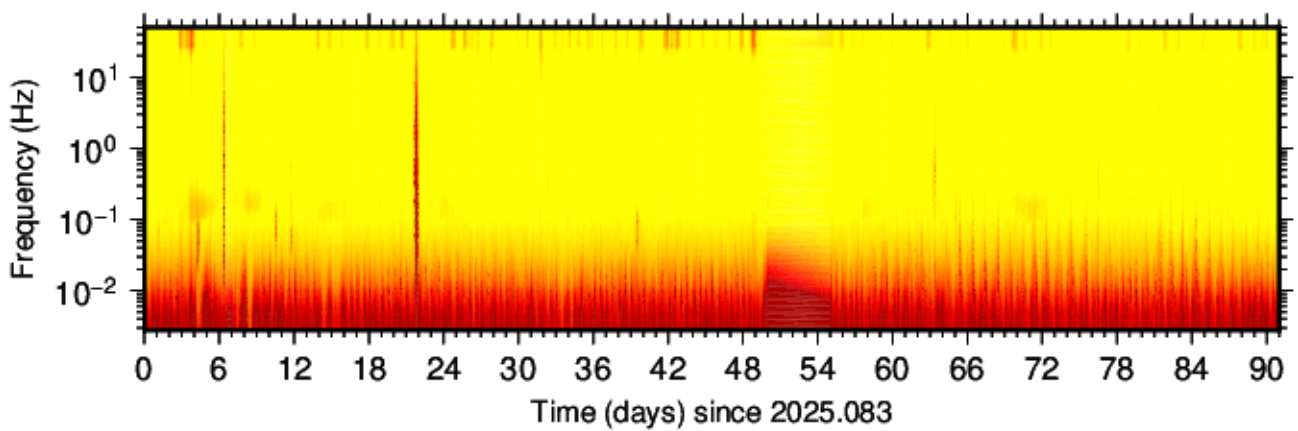
BK.LAKN.HNZ.00 (2025.083 - 2025.173)
