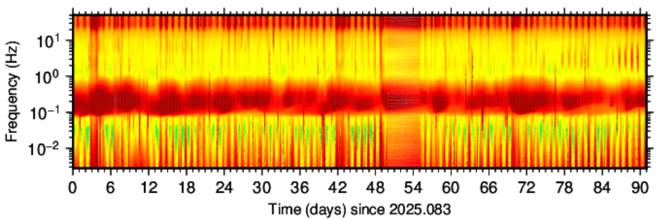
BK.LAKN.HHN.00 (2025.083 - 2025.173)
