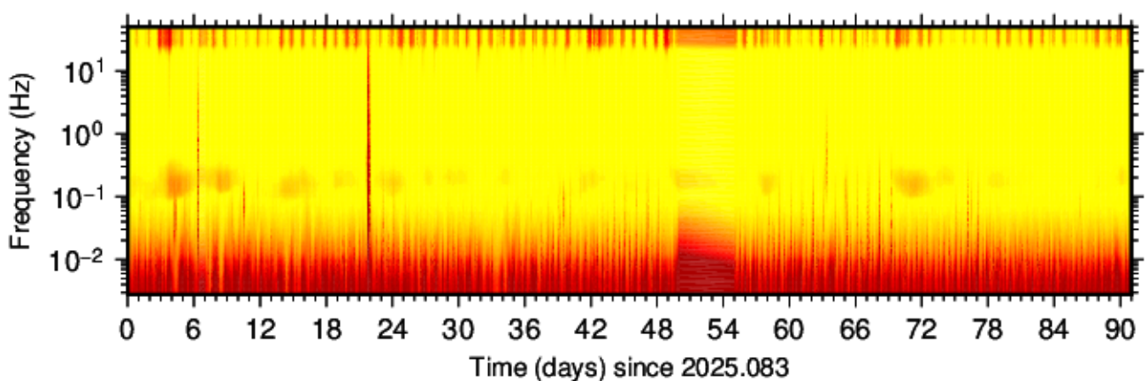
BK.LAKN.HNN.00 (2025.083 - 2025.173)
