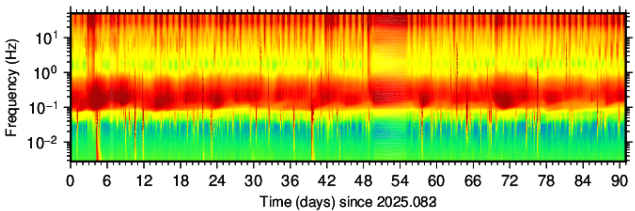
BK.LAKN.HHZ.00 (2025.083 - 2025.173)
