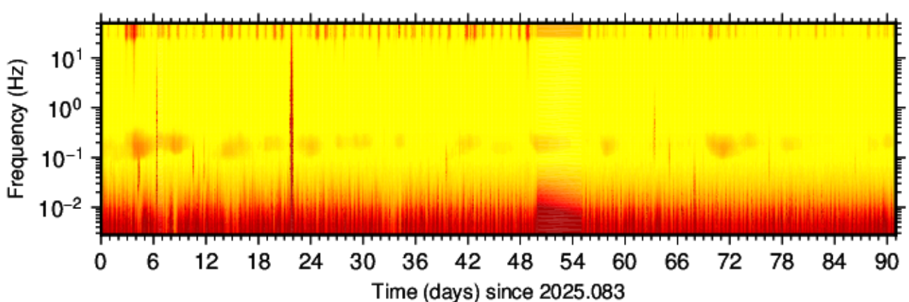
BK.LAKN.HNE.00 (2025.083 - 2025.173)
