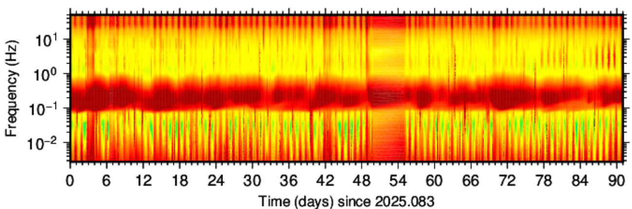
BK.LAKN.HHE.00 (2025.083 - 2025.173)
