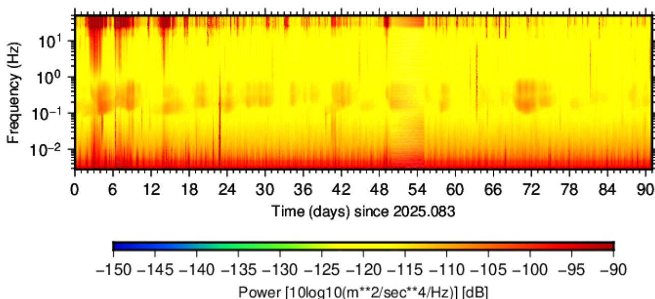
BK.KNEE.HNN.00 (2025.083 - 2025.173)
