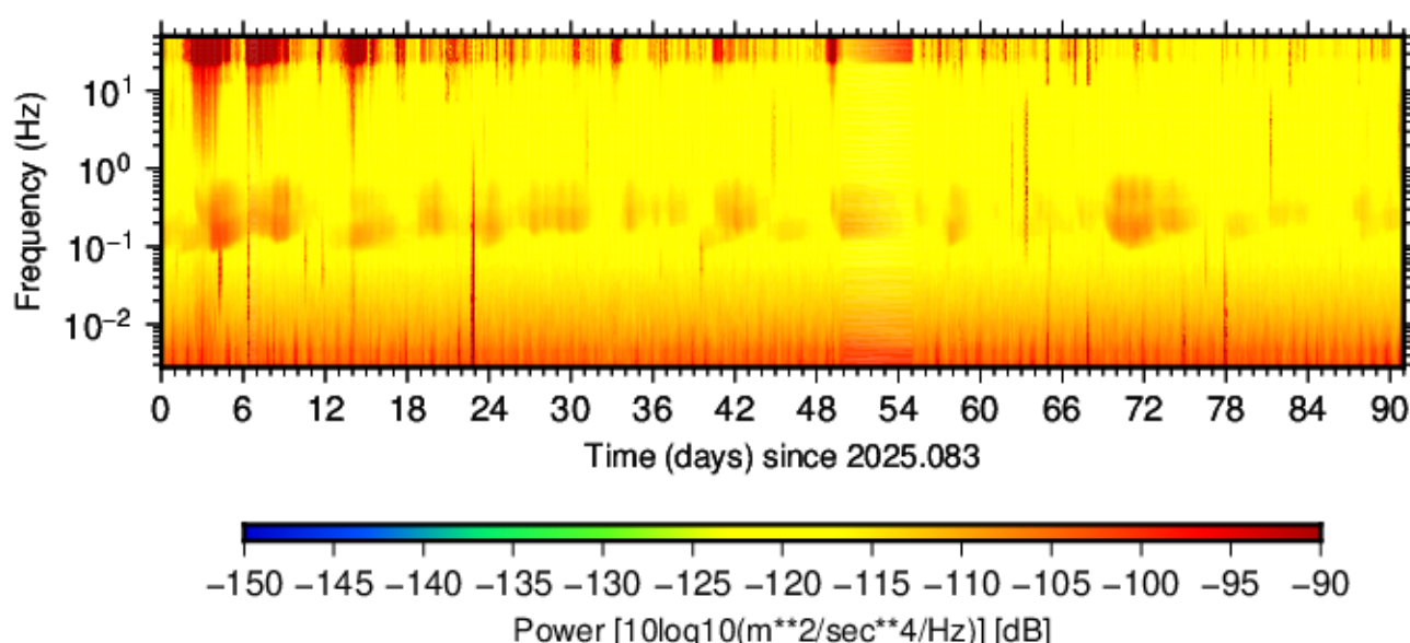
BK.KNEE.HNE.00 (2025.083 - 2025.173)
