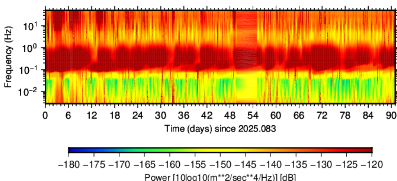
BK.KNEE.HHN.00 (2025.083 - 2025.173)
