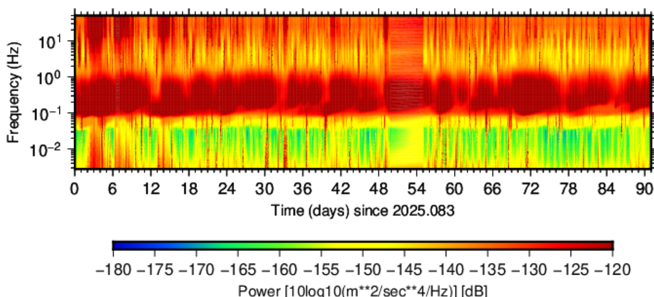
BK.KNEE.HHE.00 (2025.083 - 2025.173)
