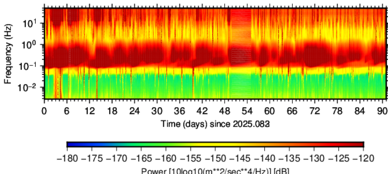
BK.KNEE.HHZ.00 (2025.083 - 2025.173)
