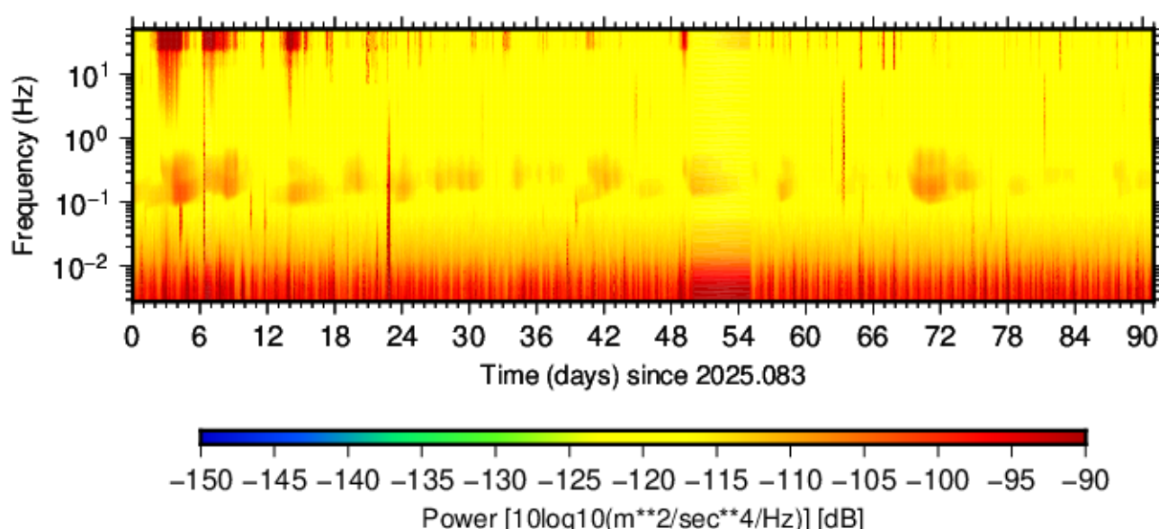
BK.KNEE.HNZ.00 (2025.083 - 2025.173)
