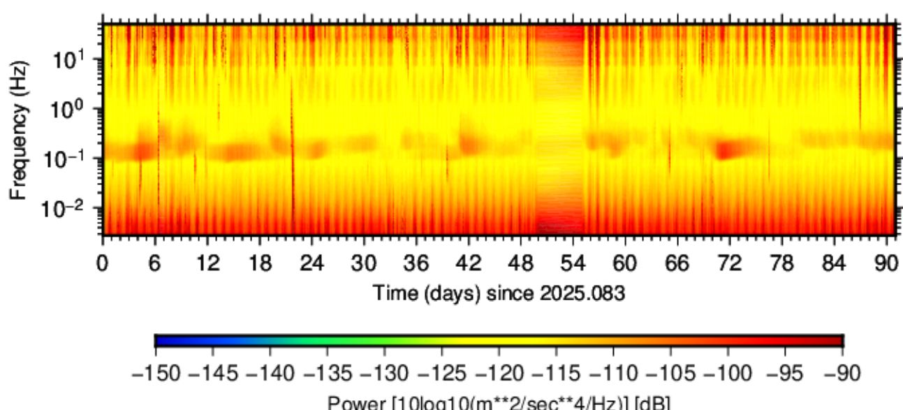
BK.KETL.HNN.00 (2025.083 - 2025.173)
