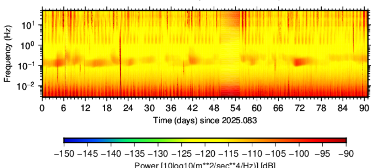
BK.KETL.HNE.00 (2025.083 - 2025.173)
