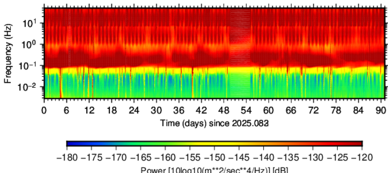
BK.KETL.HHZ.00 (2025.083 - 2025.173)
