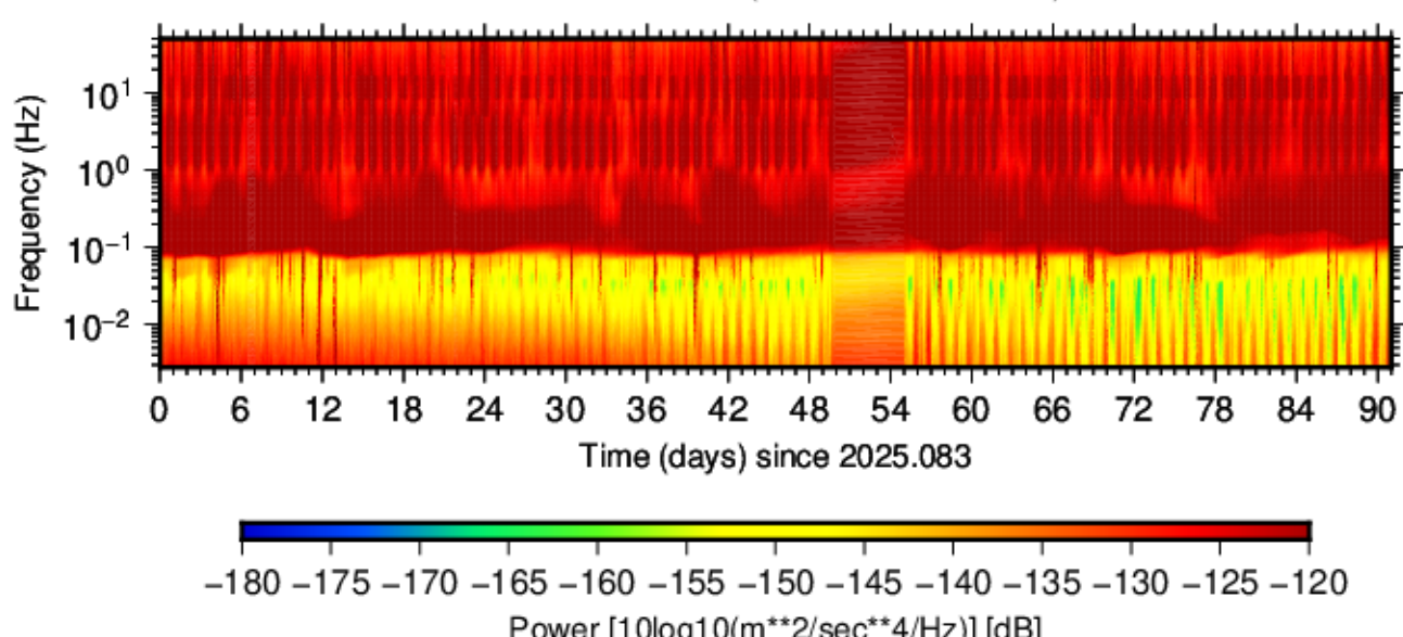
BK.KETL.HHE.00 (2025.083 - 2025.173)
