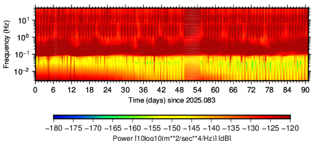
BK.KETL.HHN.00 (2025.083 - 2025.173)
