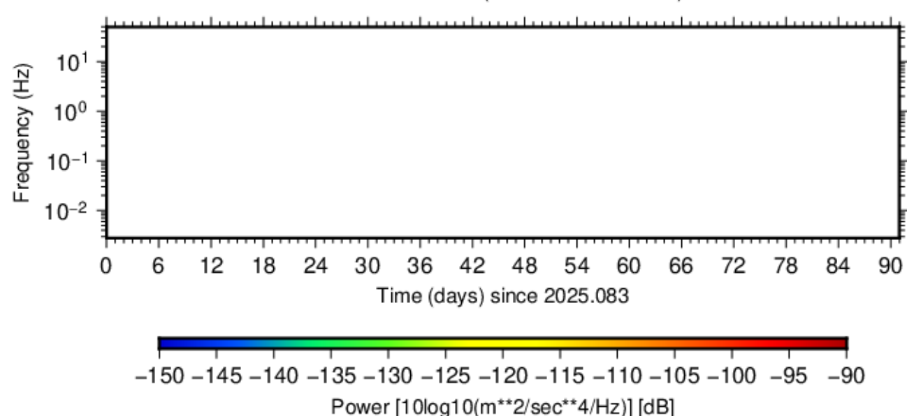
BK.KCC.HNN.00 (2025.083 - 2025.173)
