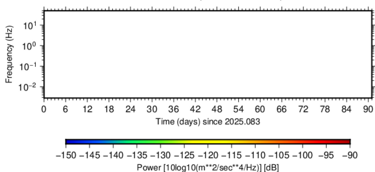
BK.KCC.HNE.00 (2025.083 - 2025.173)
