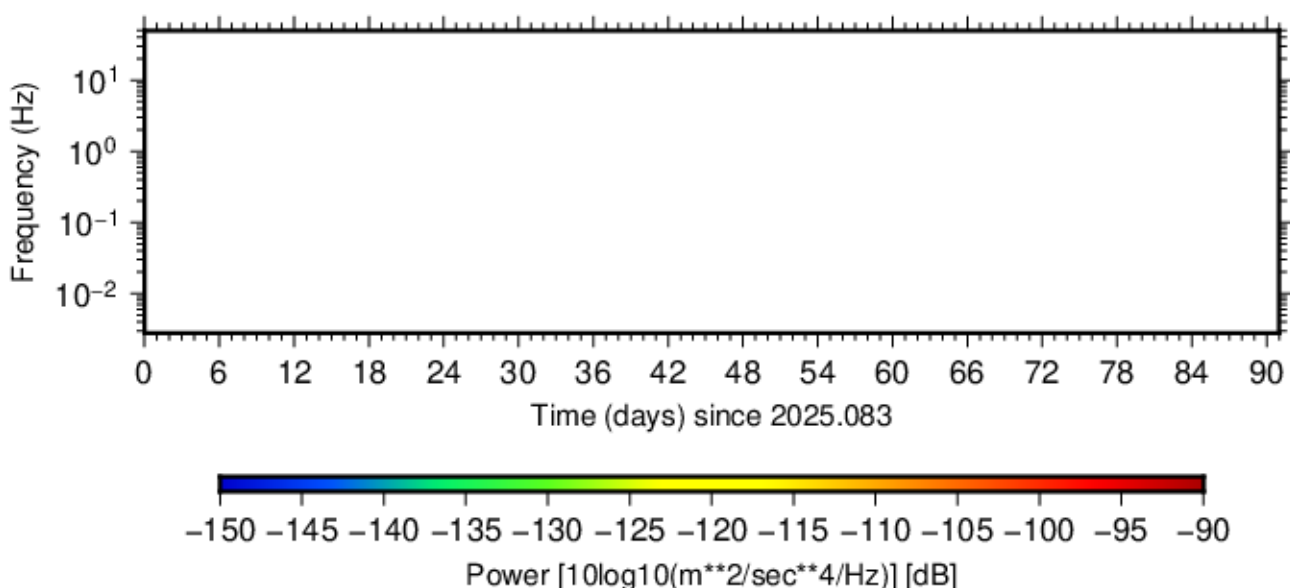
BK.JRSC.HNN.00 (2025.083 - 2025.173)
