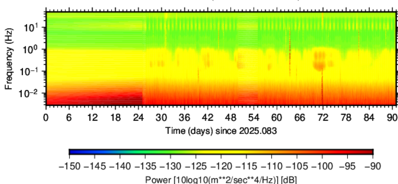
BK.JCC.HNN.00 (2025.083 - 2025.173)
