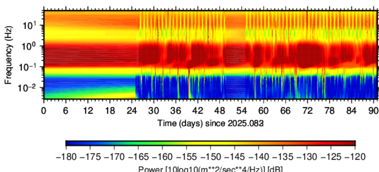
BK.JCC.HHZ.00 (2025.083 - 2025.173)
