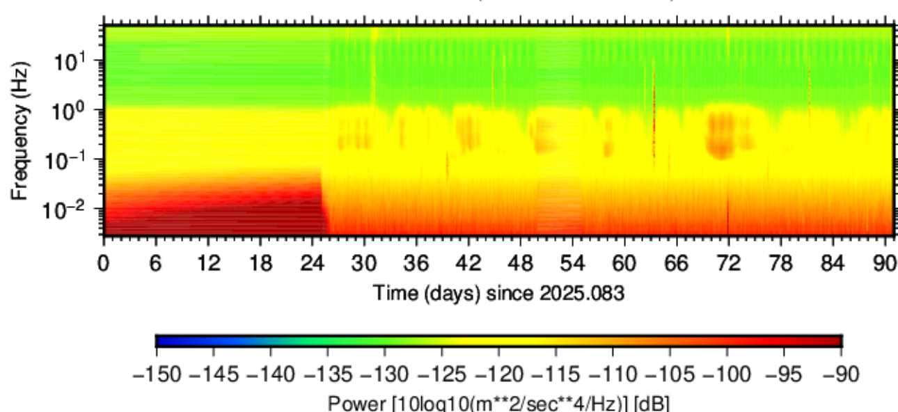
BK.JCC.HNZ.00 (2025.083 - 2025.173)
