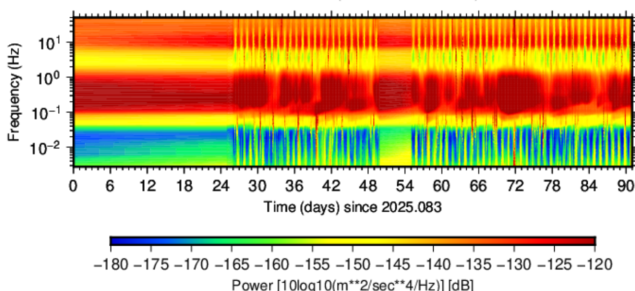
BK.JCC.HHE.00 (2025.083 - 2025.173)
