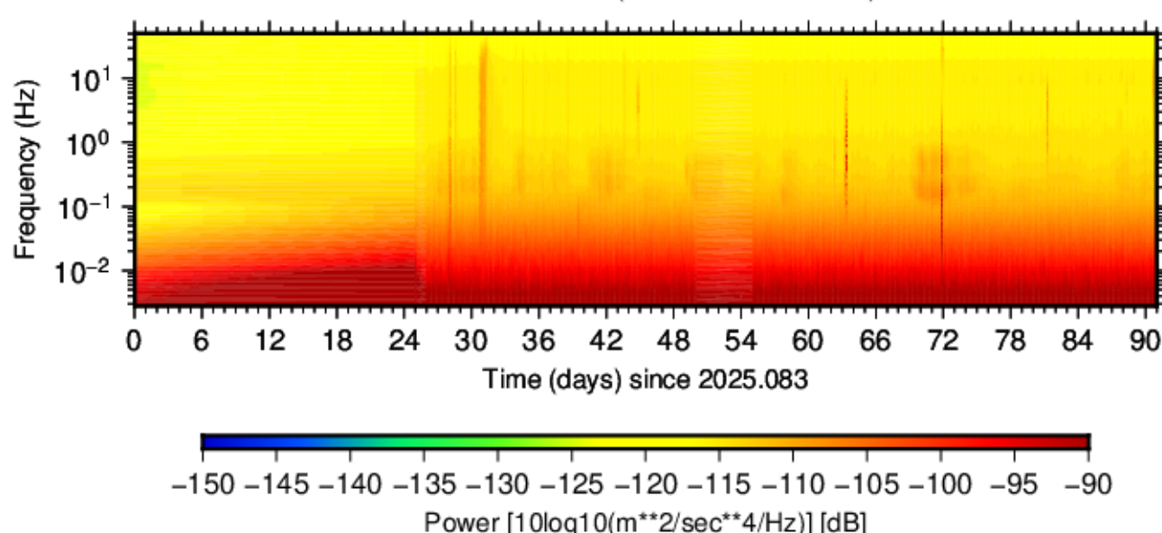
BK.JCC.HNE.00 (2025.083 - 2025.173)
