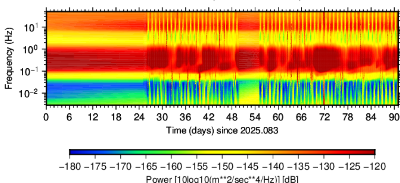
BK.JCC.HHN.00 (2025.083 - 2025.173)
