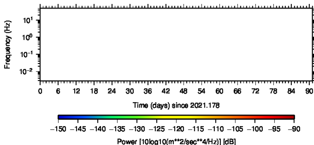
BK.HUMO.HHE.00 (2021.178 – 2021.268)
