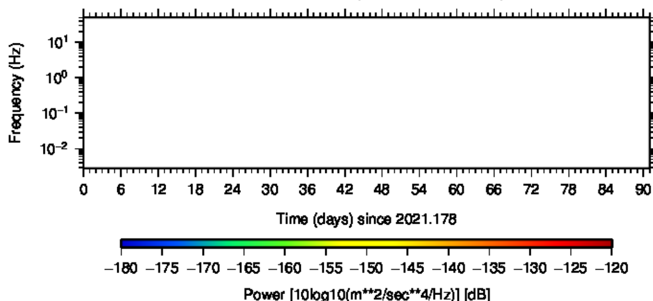
BK.HUMO.HNZ.00 (2021.178 – 2021.268)
