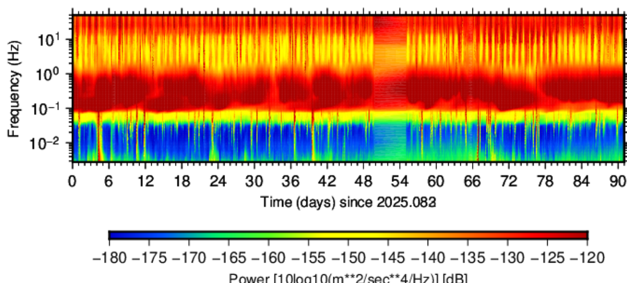
BK.HULI.HHZ.00 (2025.083 - 2025.173)
