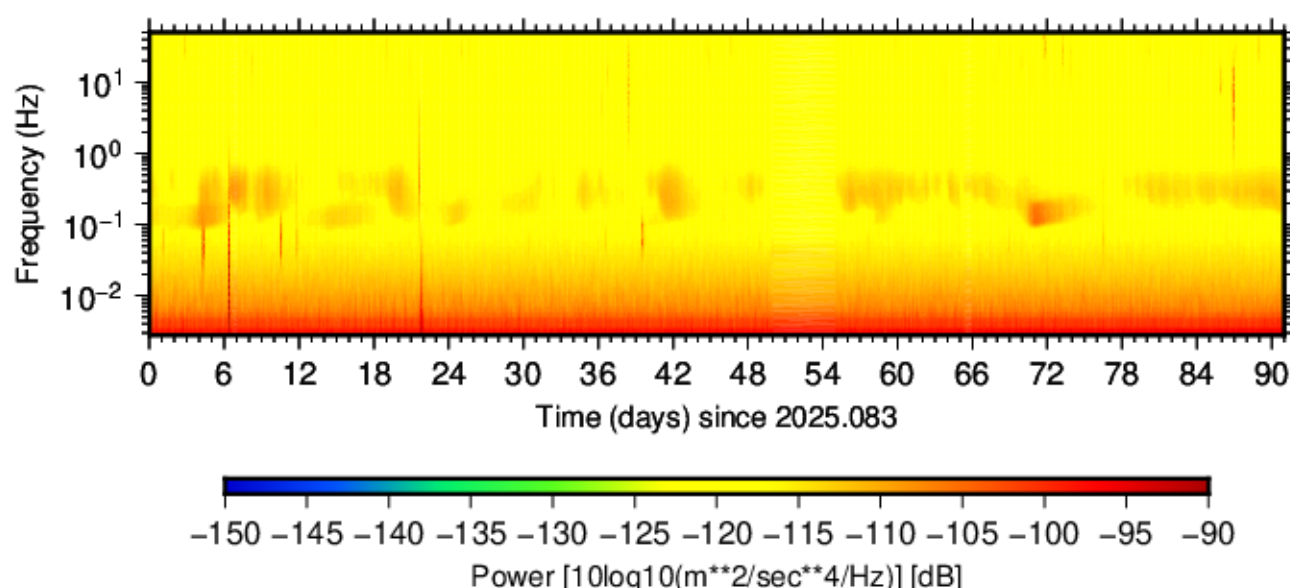
BK.HULI.HNZ.00 (2025.083 - 2025.173)
