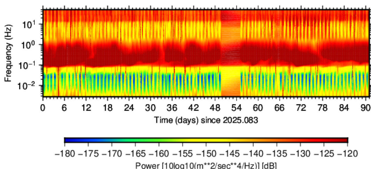
BK.HULI.HHN.00 (2025.083 - 2025.173)
