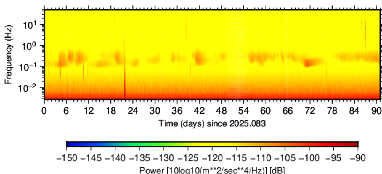
BK.HULI.HNE.00 (2025.083 - 2025.173)
