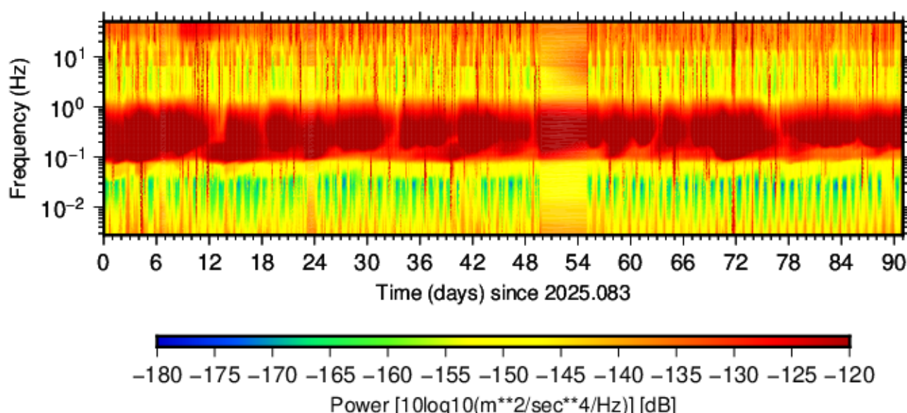
BK.HOPS.HHE.00 (2025.083 - 2025.173)
