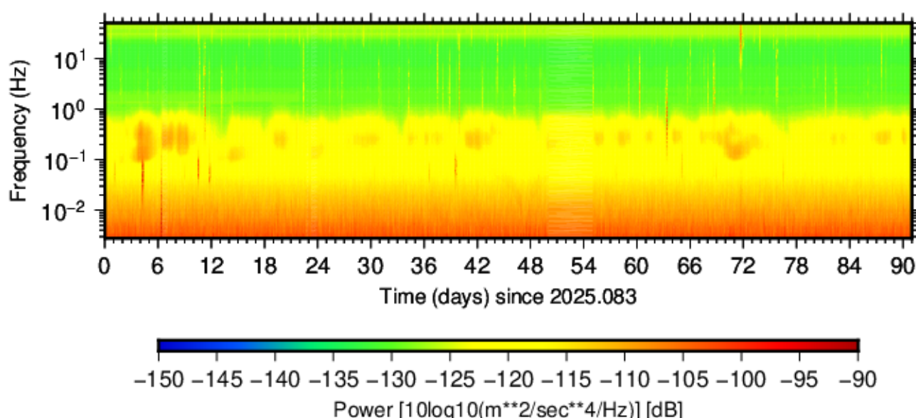
BK.HOPS.HNZ.00 (2025.083 - 2025.173)
