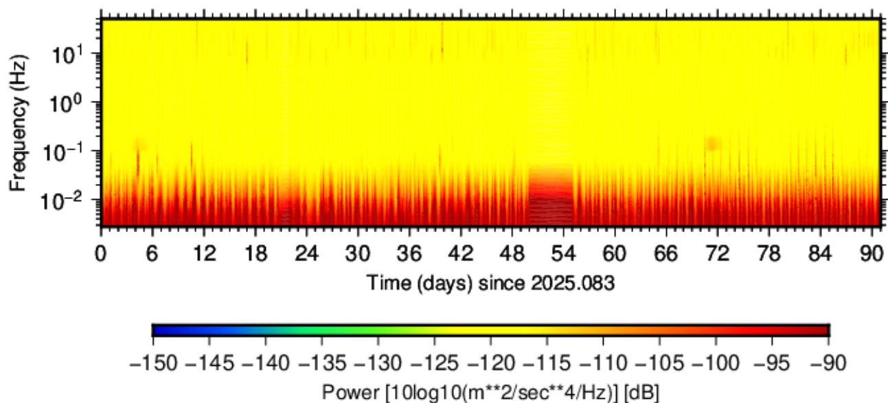
BK.HELL.HNZ.00 (2025.083 - 2025.173)
