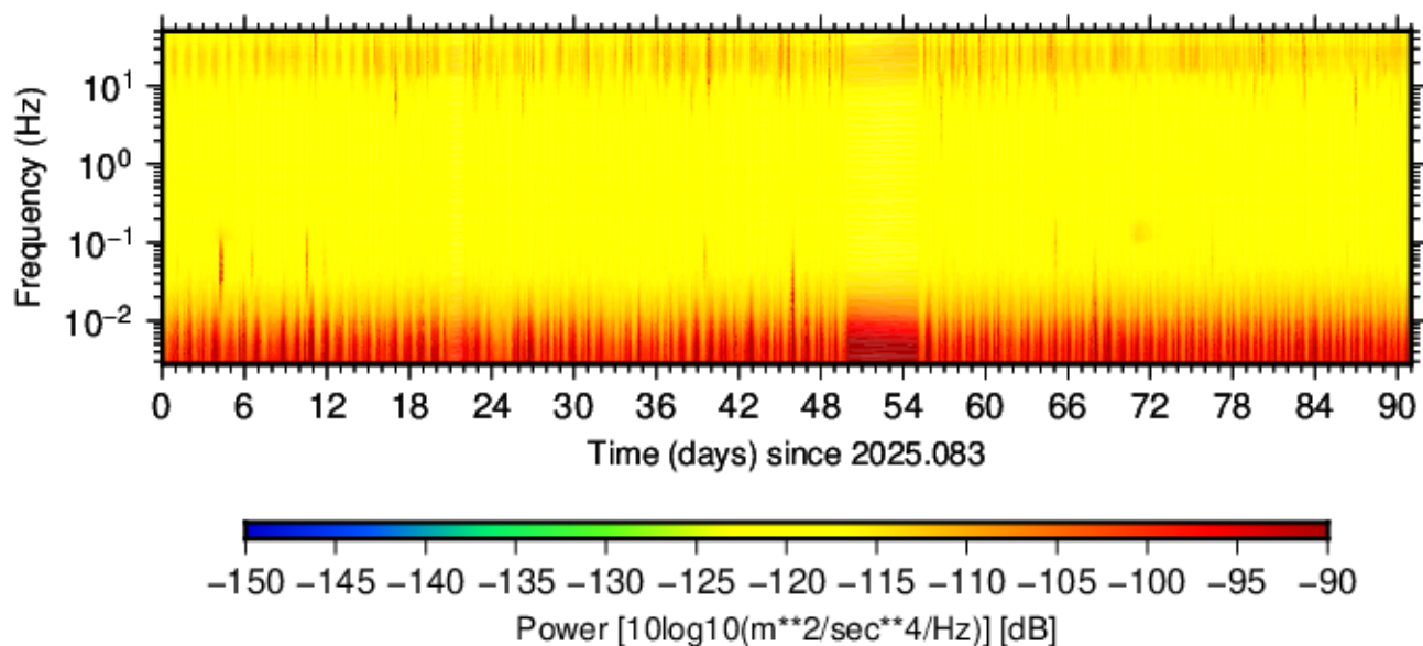
BK.HELL.HNE.00 (2025.083 - 2025.173)
