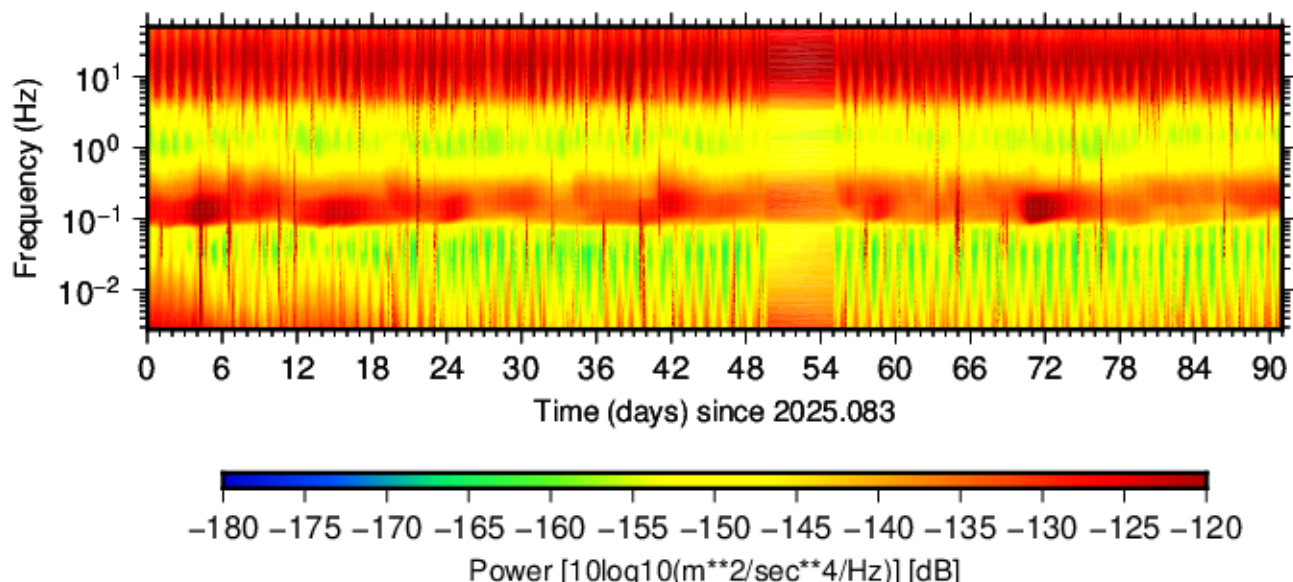
BK.HELL.HHE.00 (2025.083 - 2025.173)
