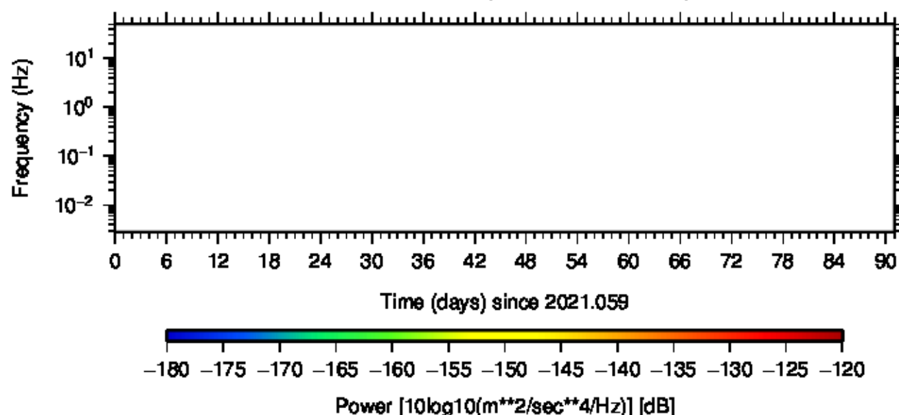
BK.HAST.HNZ.00 (2021.059 – 2021.149)
