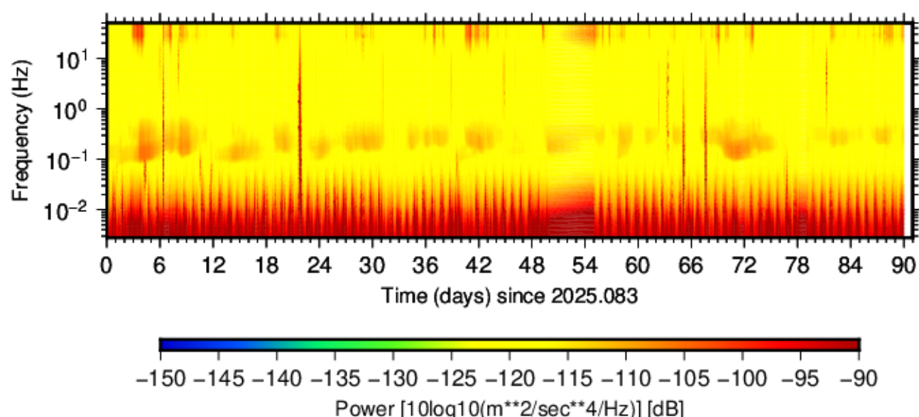
BK.HALS.HNZ.00 (2025.083 - 2025.173)
