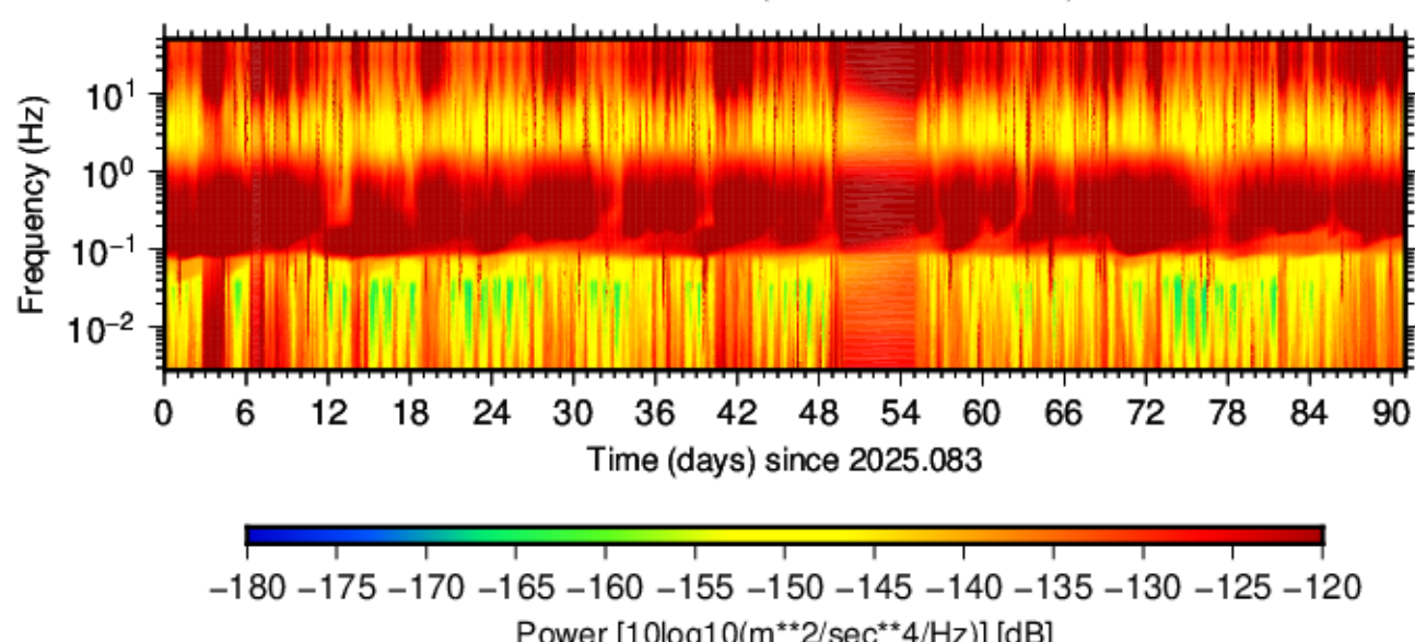
BK.HALS.HHE.00 (2025.083 - 2025.173)
