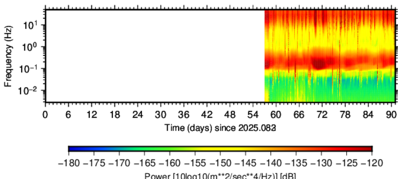
BK.GRPK.HHZ.00 (2025.083 - 2025.173)
