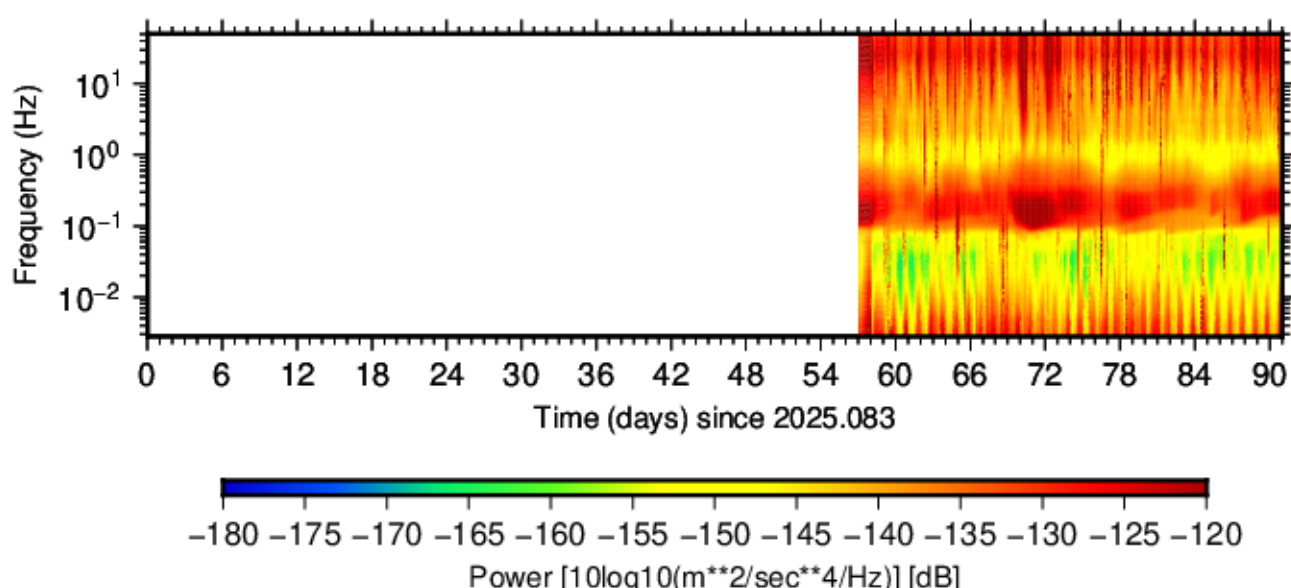
BK.GRPK.HHN.00 (2025.083 - 2025.173)
