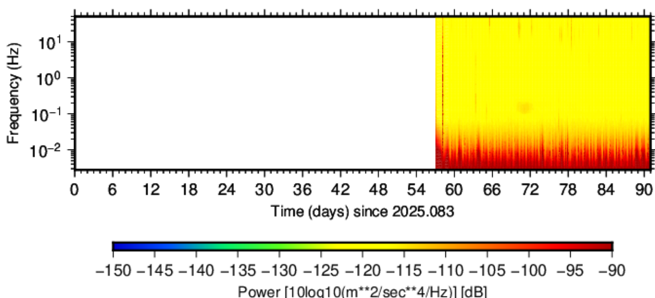
BK.GRPK.HNZ.00 (2025.083 - 2025.173)
