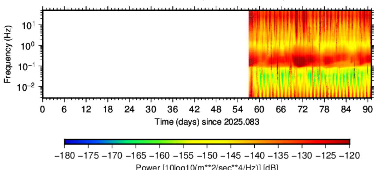
BK.GRPK.HHE.00 (2025.083 - 2025.173)
