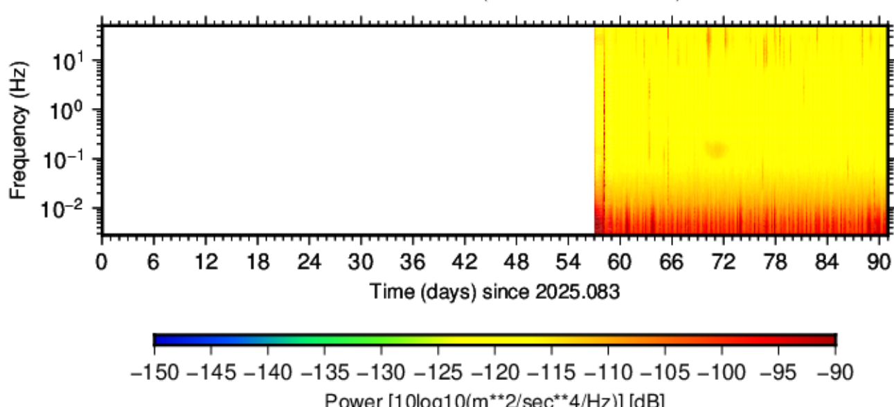
BK.GRPK.HNE.00 (2025.083 - 2025.173)
