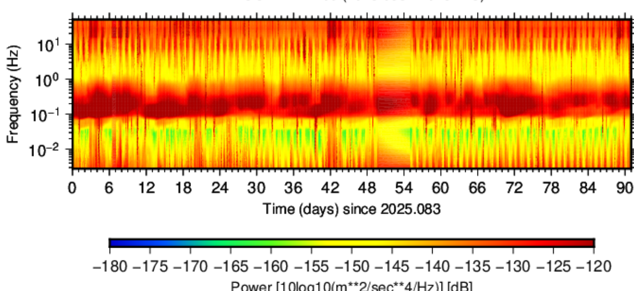
BK.GCKB.HHE.00 (2025.083 - 2025.173)
