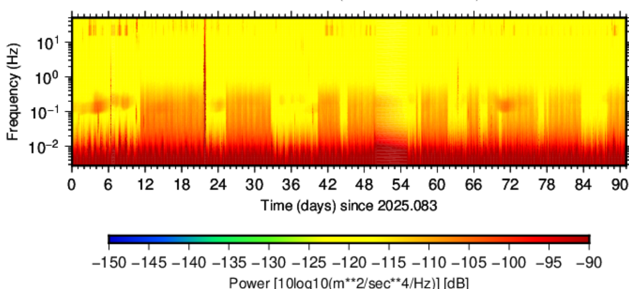
BK.GCKB.HNZ.00 (2025.083 - 2025.173)
