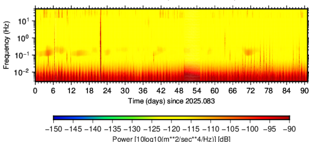
BK.GCKB.HNE.00 (2025.083 - 2025.173)
