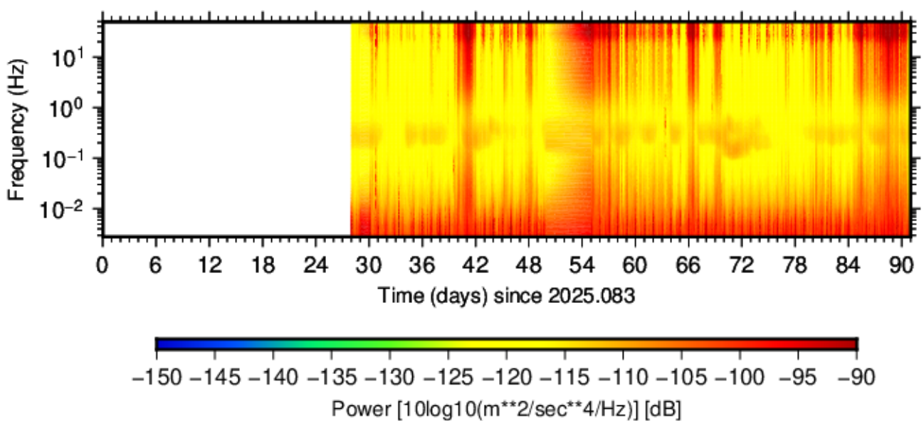
BK.GALB.HNN.00 (2025.083 - 2025.173)
