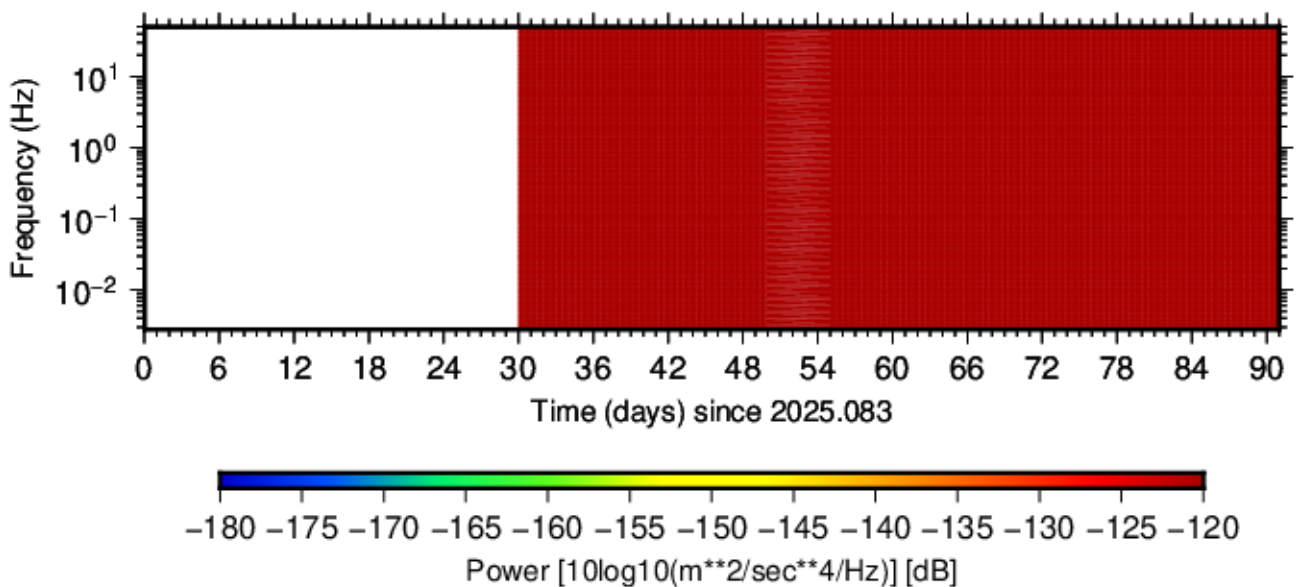
BK.GALB.HHE.00 (2025.083 - 2025.173)
