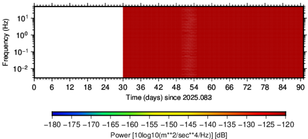
BK.GALB.HHZ.00 (2025.083 - 2025.173)
