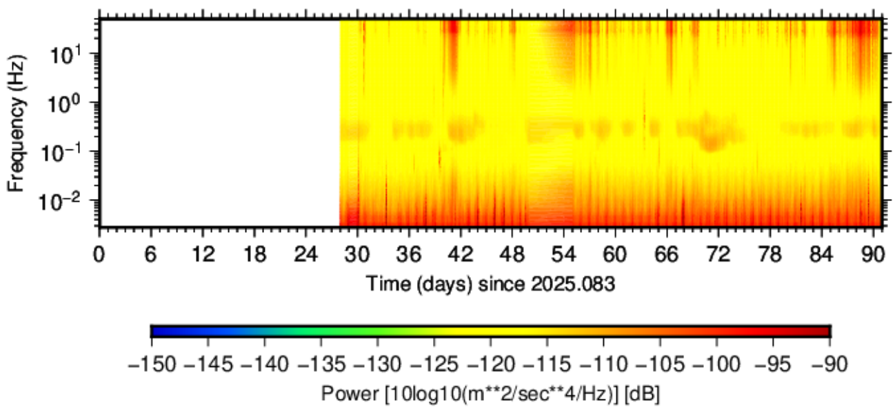
BK.GALB.HNZ.00 (2025.083 - 2025.173)
