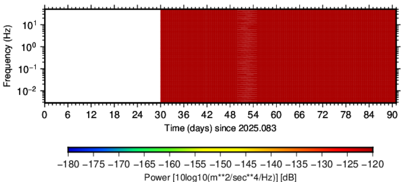
BK.GALB.HHN.00 (2025.083 - 2025.173)
