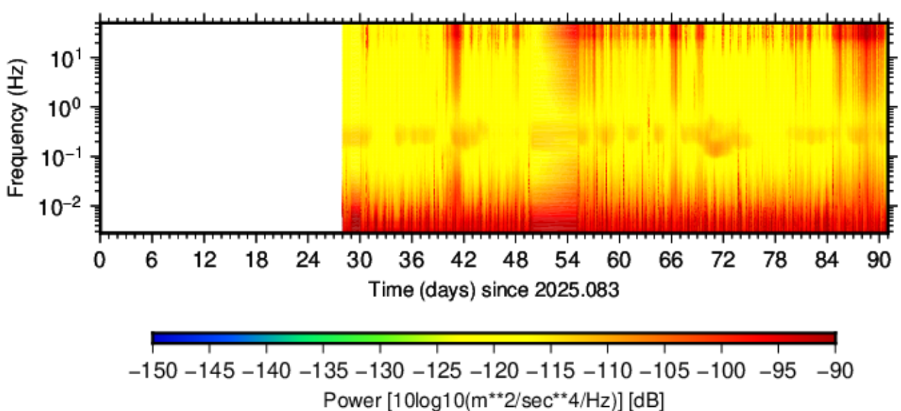
BK.GALB.HNE.00 (2025.083 - 2025.173)
