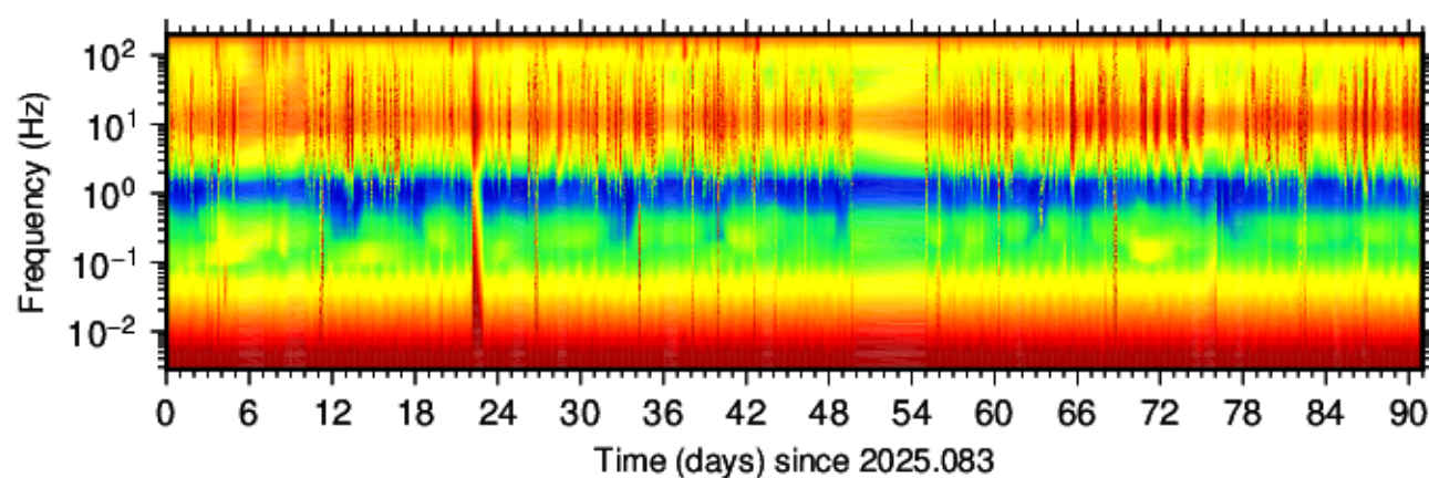
BG.FUM.DPE. (2025.083 - 2025.173)
