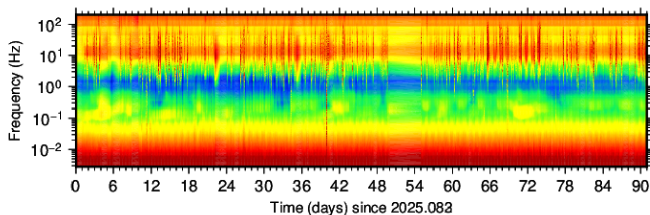
BG.FUM.DPZ. (2025.083 - 2025.173)
