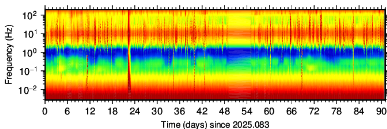
BG.FUM.DPN. (2025.083 - 2025.173)
