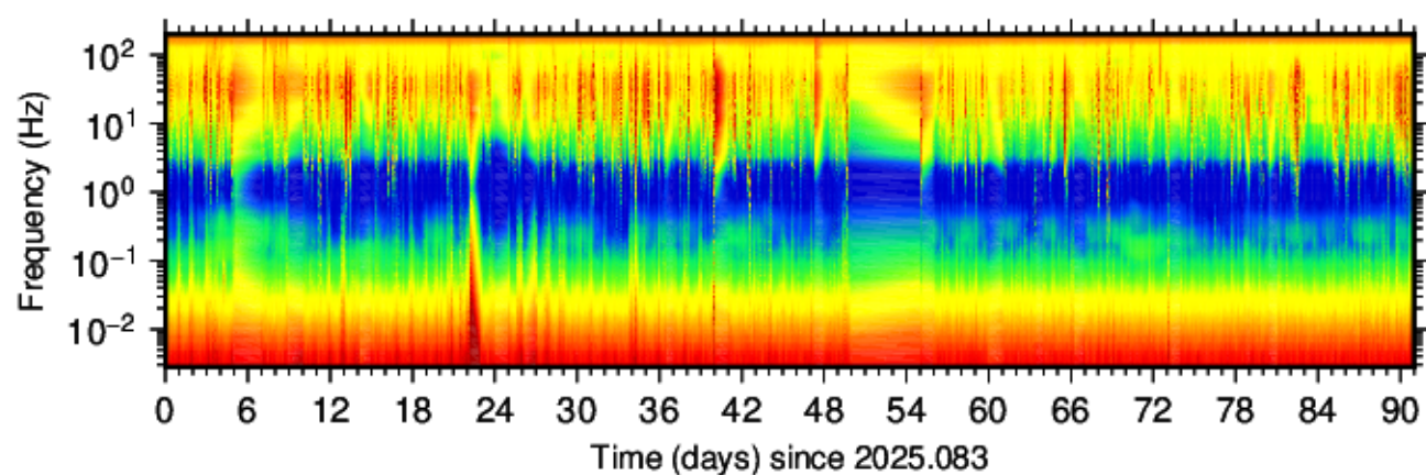
BG.FNF.DPE. (2025.083 - 2025.173)
