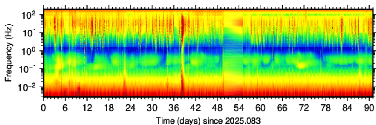
BG.FNF.DPN. (2025.083 - 2025.173)
