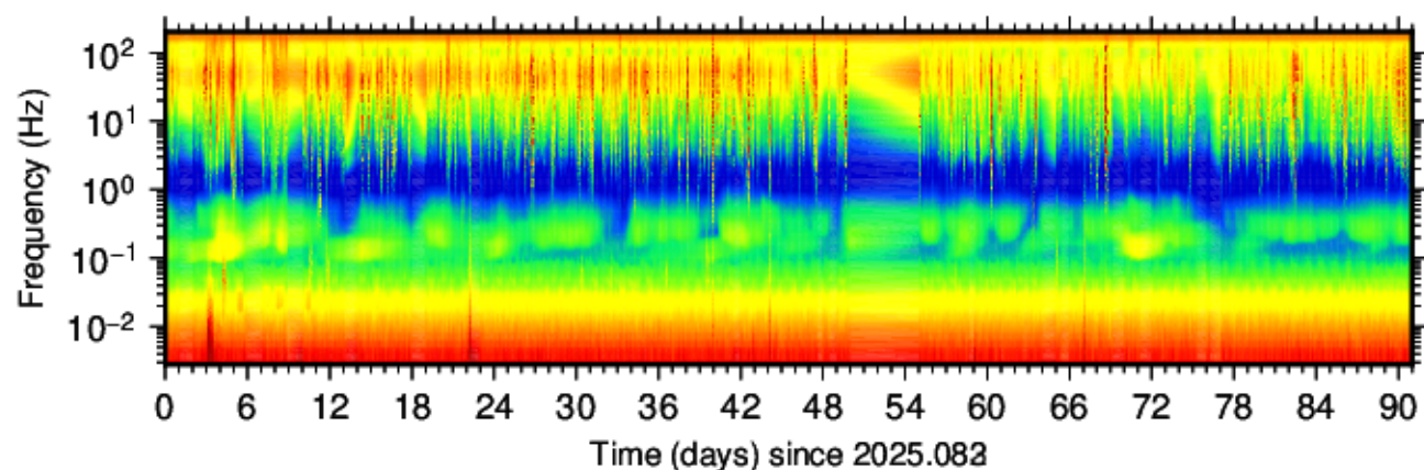
BG.FNF.DPZ. (2025.083 - 2025.173)
