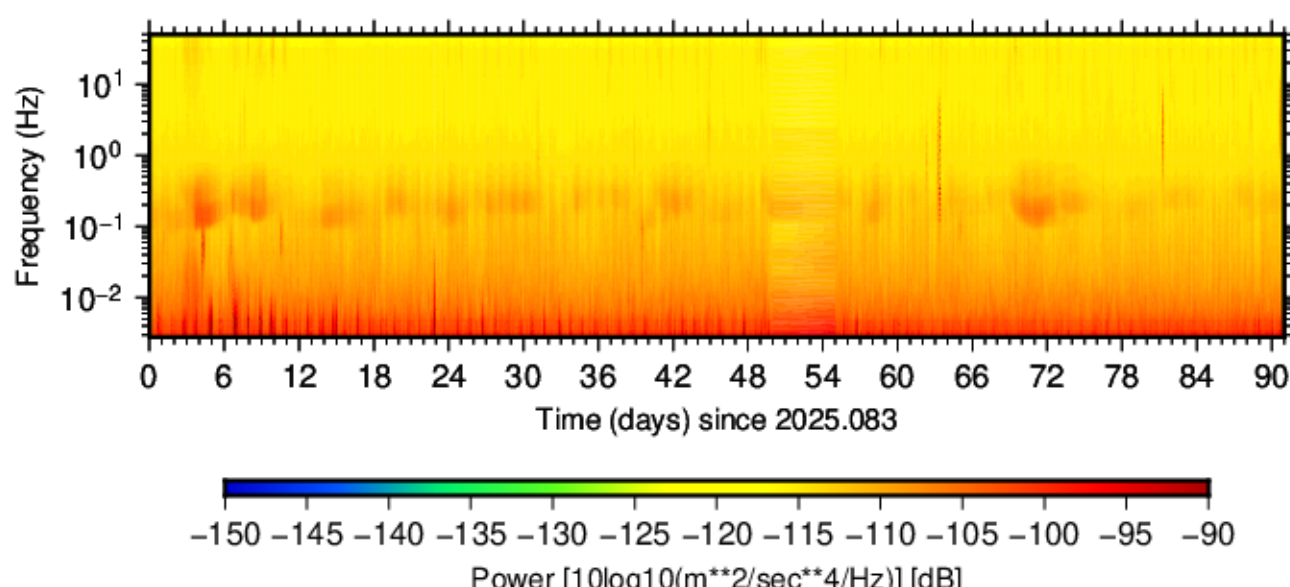
BK.DMOR.HNN.00 (2025.083 - 2025.173)
