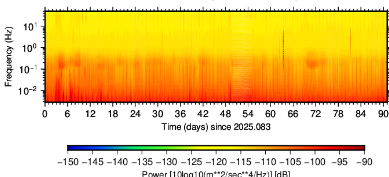
BK.DMOR.HNE.00 (2025.083 - 2025.173)
