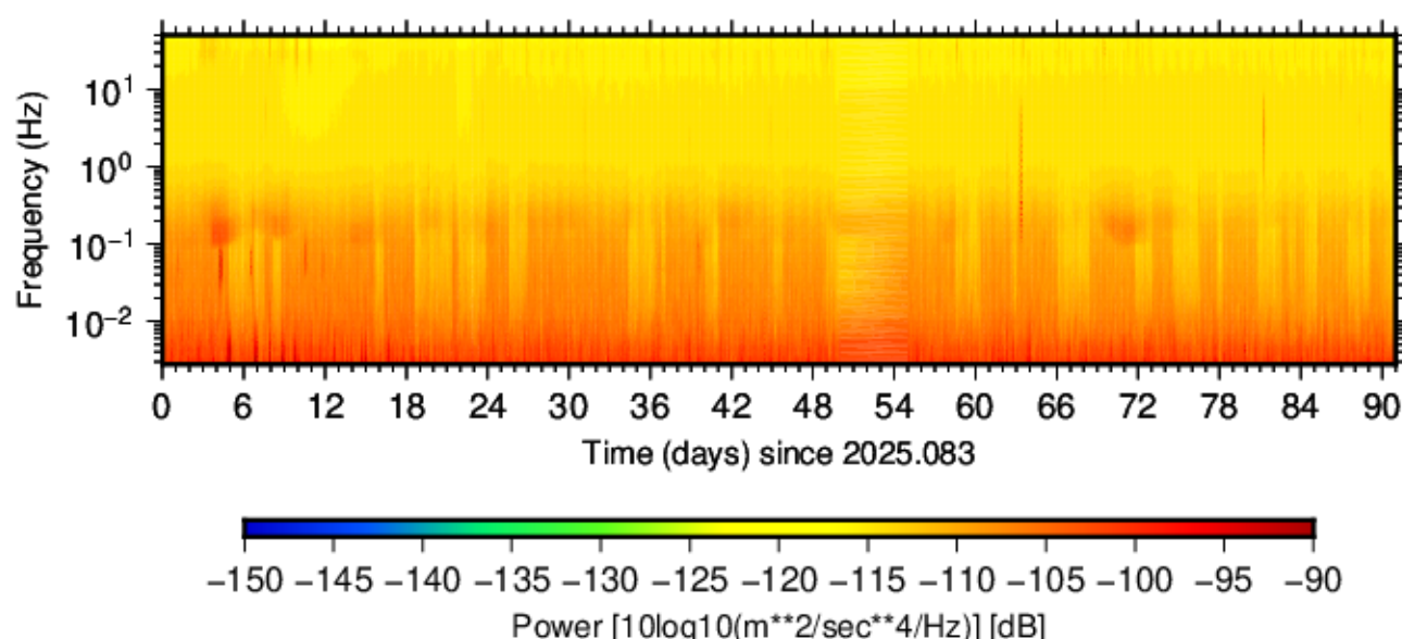
BK.DMOR.HNZ.00 (2025.083 - 2025.173)
