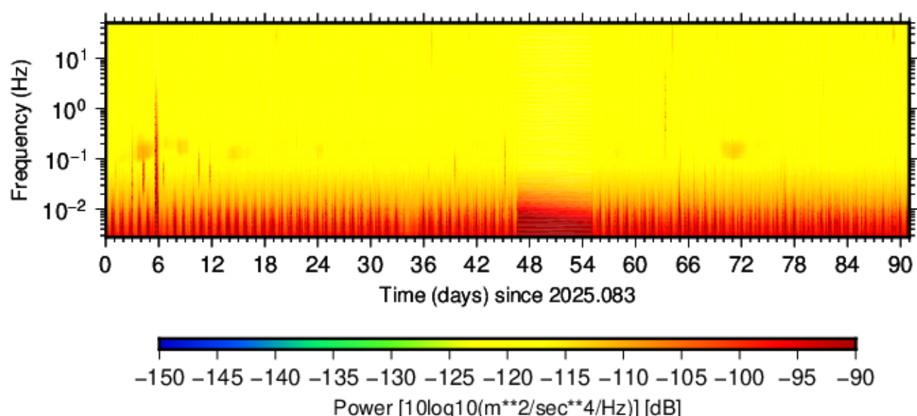
BK.DLIK.HNZ.00 (2025.083 - 2025.173)
