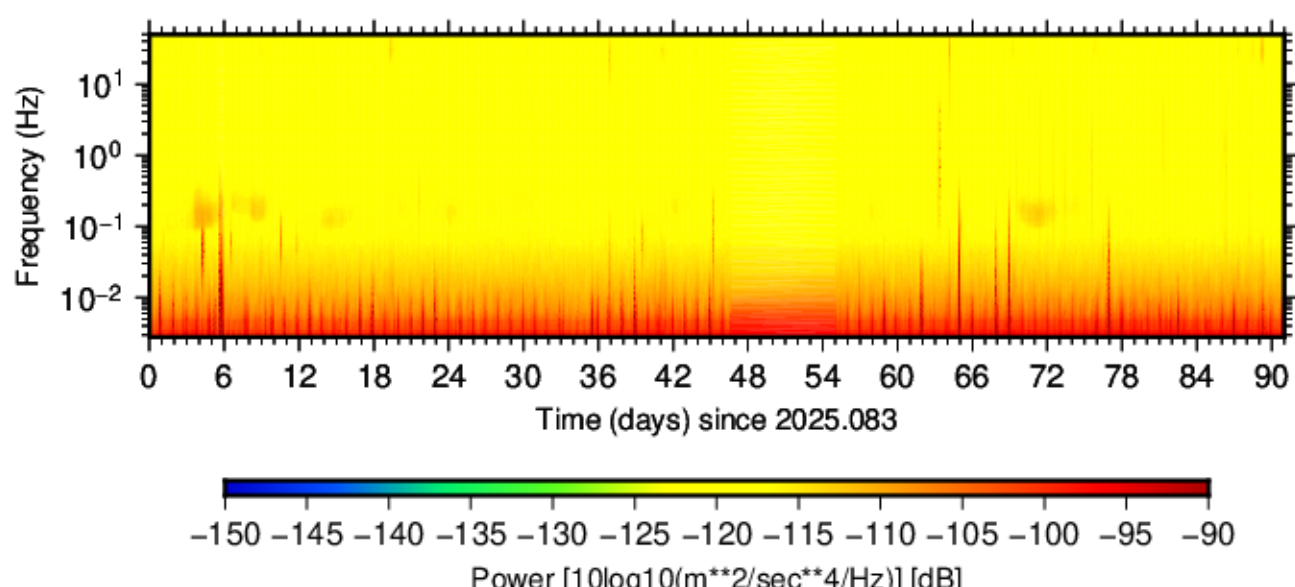
BK.DLIK.HNN.00 (2025.083 - 2025.173)
