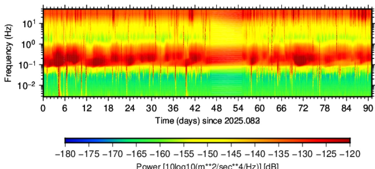
BK.DLIK.HHZ.00 (2025.083 - 2025.173)
