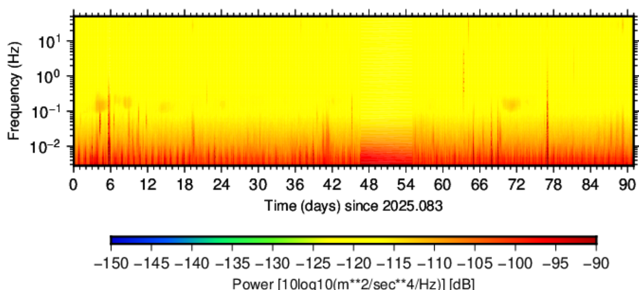
BK.DLIK.HNE.00 (2025.083 - 2025.173)
