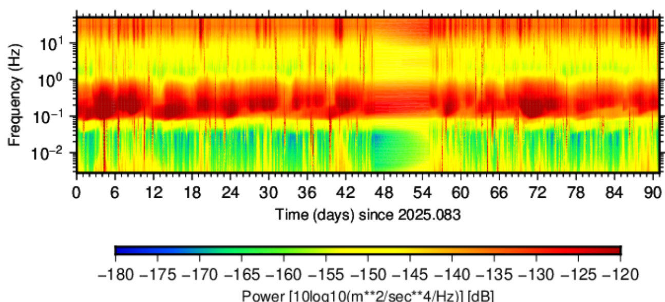
BK.DLIK.HHN.00 (2025.083 - 2025.173)
