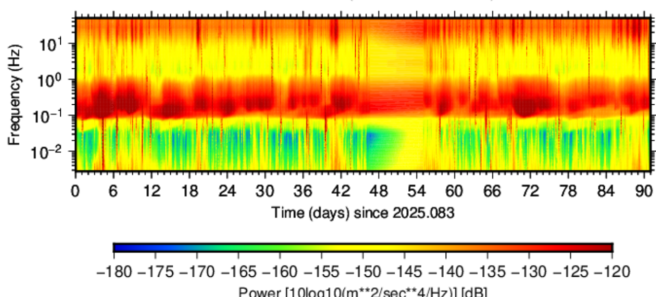
BK.DLIK.HHE.00 (2025.083 - 2025.173)
