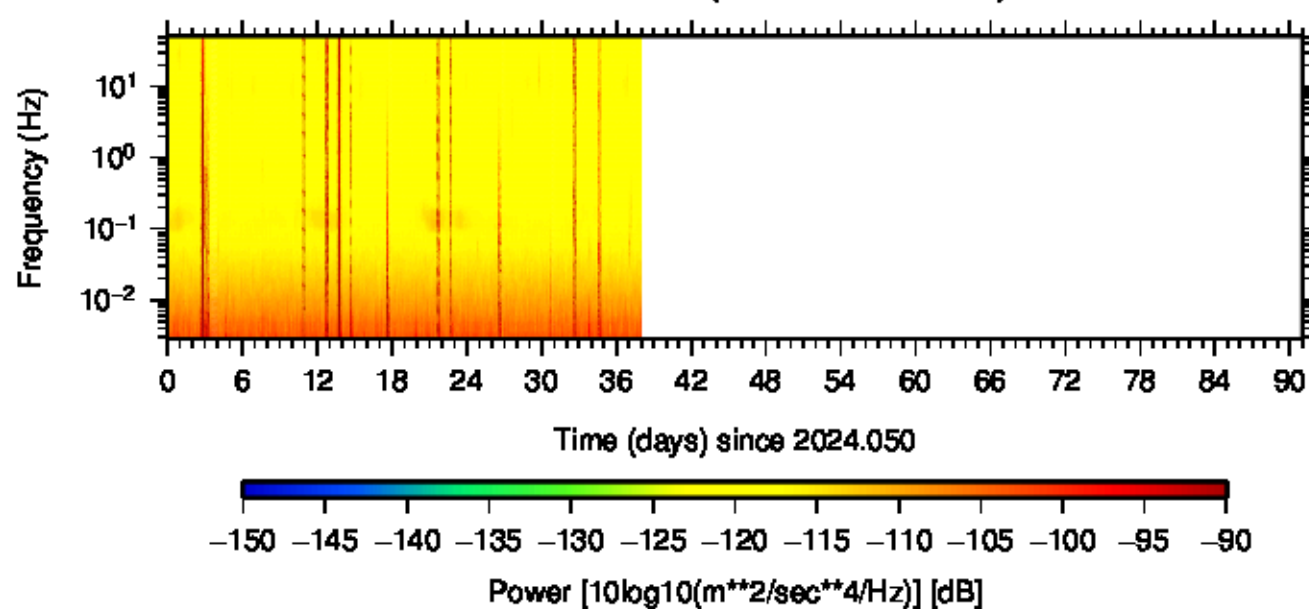
BK.DANT.HHN.00 (2024.050 – 2024.140)
