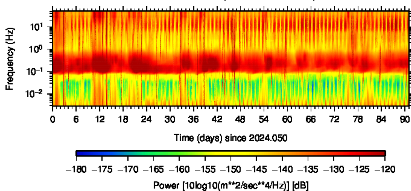
BK.DANT.HNE.00 (2024.050 – 2024.140)
