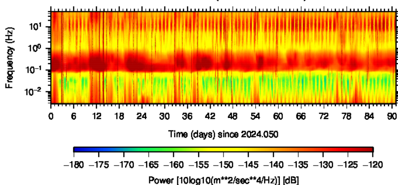
BK.DANT.HNN.00 (2024.050 – 2024.140)
