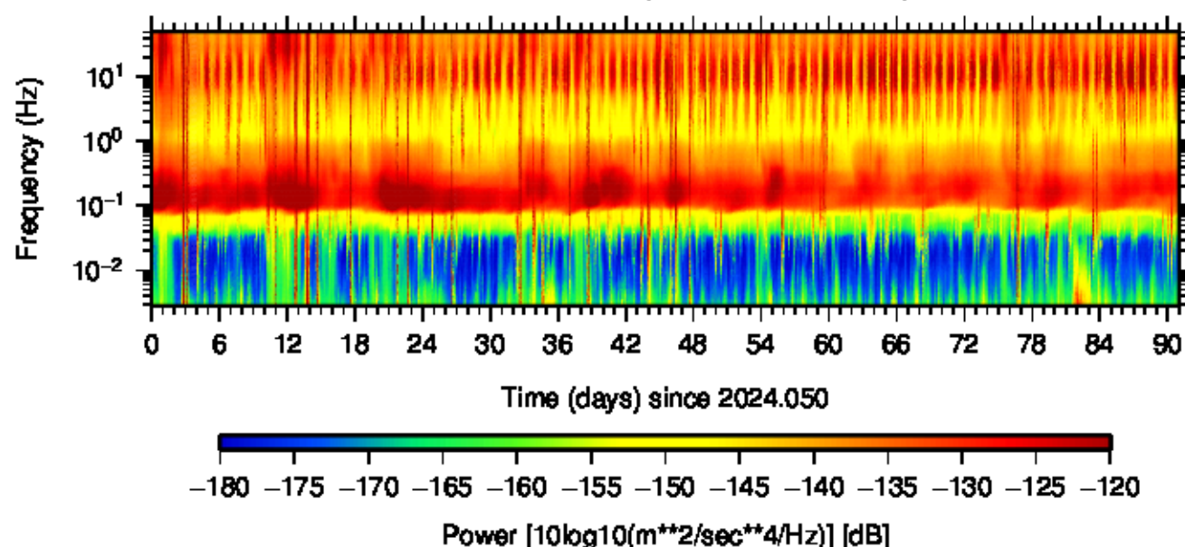
BK.DANT.HNZ.00 (2024.050 – 2024.140)
