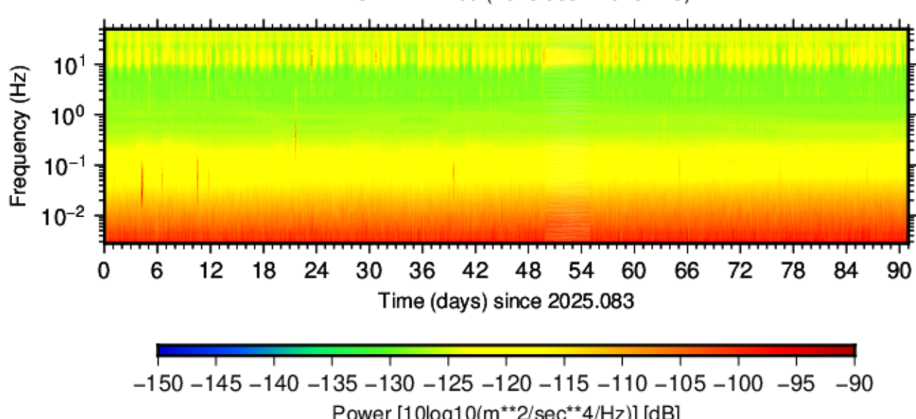
BK.CMB.HNE.00 (2025.083 - 2025.173)
