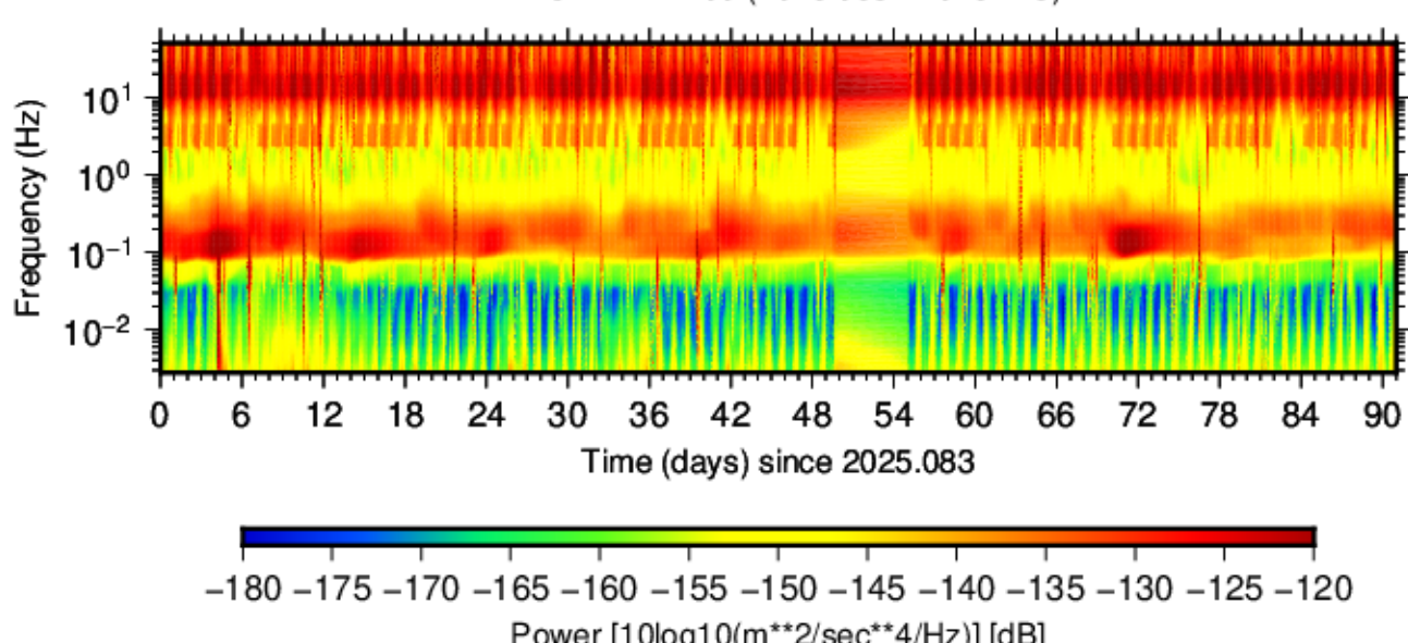
BK.CMB.HHE.00 (2025.083 - 2025.173)
