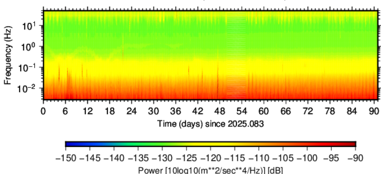
BK.CMB.HNZ.00 (2025.083 - 2025.173)
