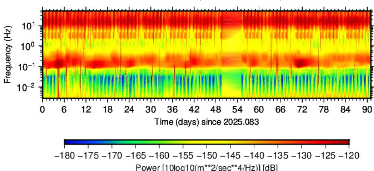
BK.CMB.HHN.00 (2025.083 - 2025.173)
