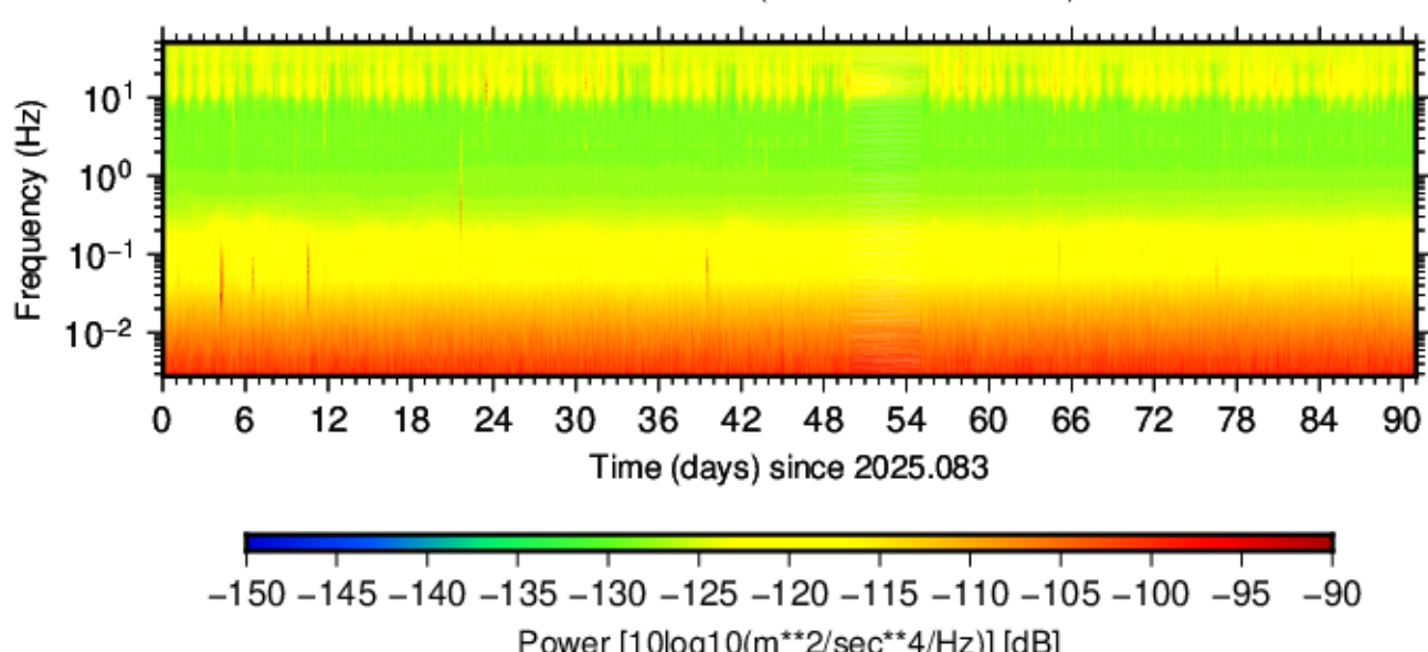
BK.CMB.HNN.00 (2025.083 - 2025.173)
