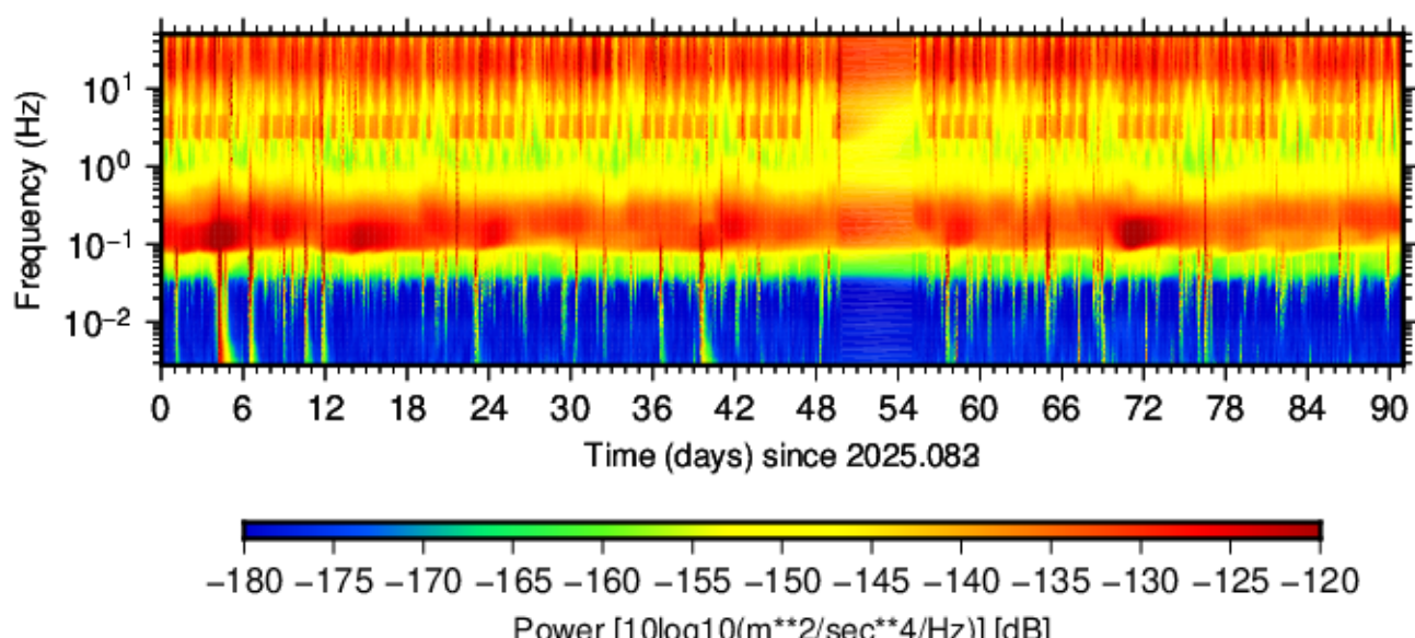
BK.CMB.HHZ.00 (2025.083 - 2025.173)
