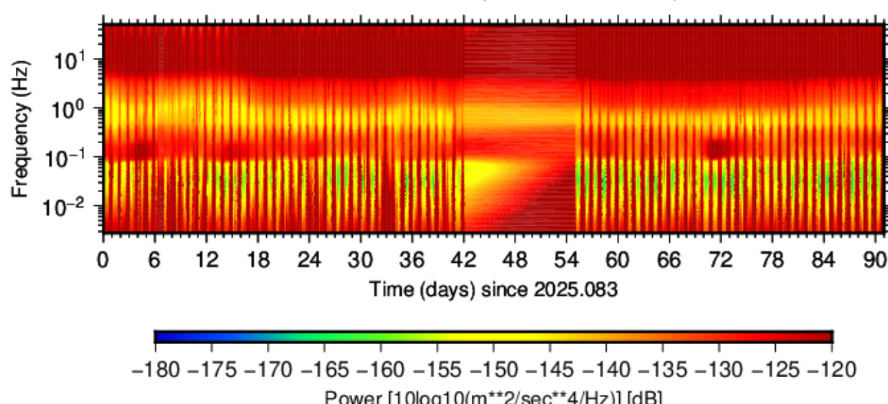
BK.CGRV.HHE.00 (2025.083 - 2025.173)
