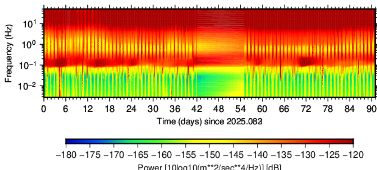
BK.CGRV.HHZ.00 (2025.083 - 2025.173)
