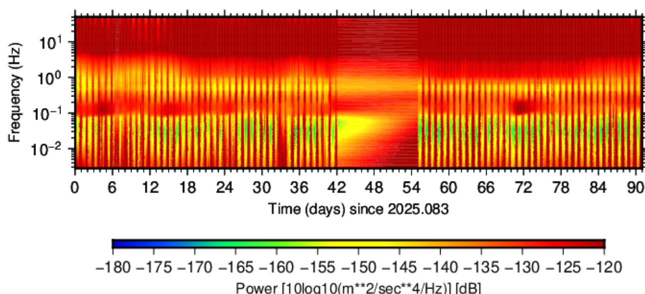
BK.CGRV.HHN.00 (2025.083 - 2025.173)
