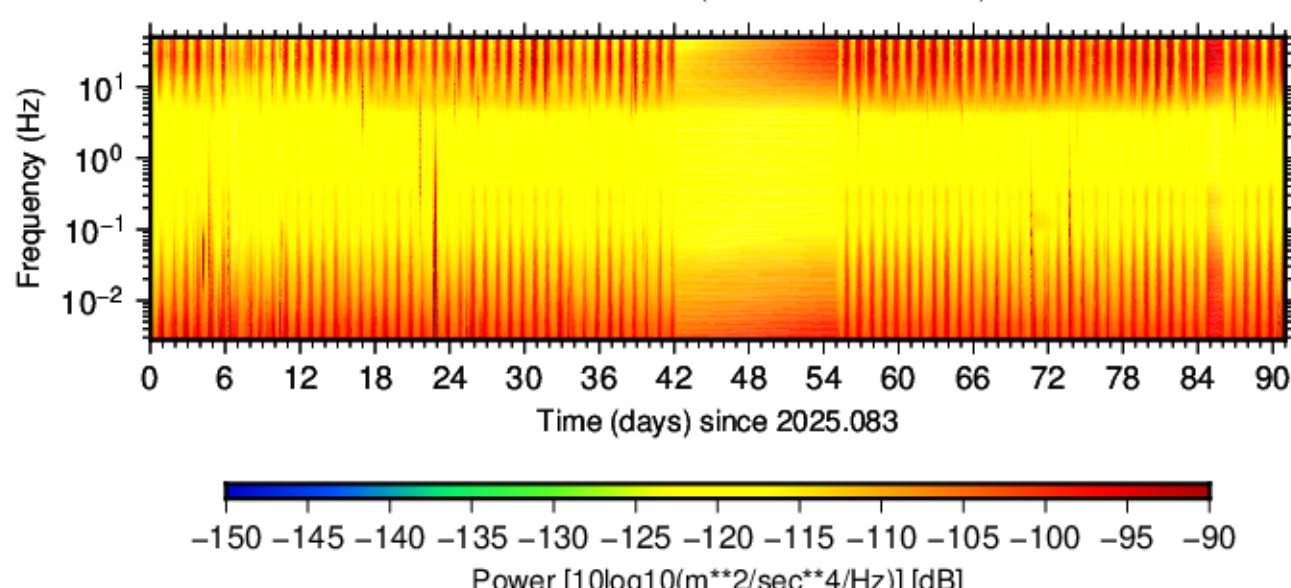
BK.CGRV.HNE.00 (2025.083 - 2025.173)
