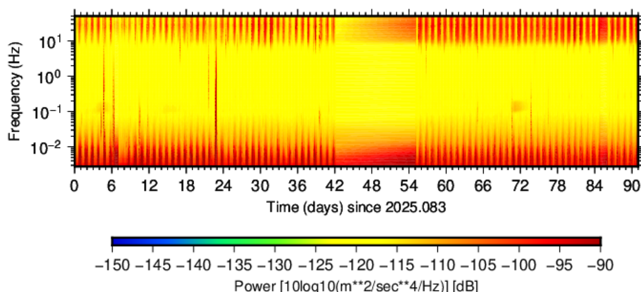
BK.CGRV.HNZ.00 (2025.083 - 2025.173)
