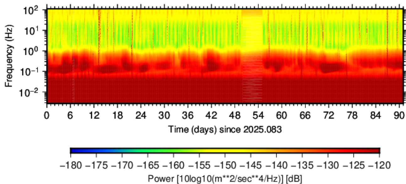
BP.CCRB.DP2.40 (2025.083 - 2025.173)
