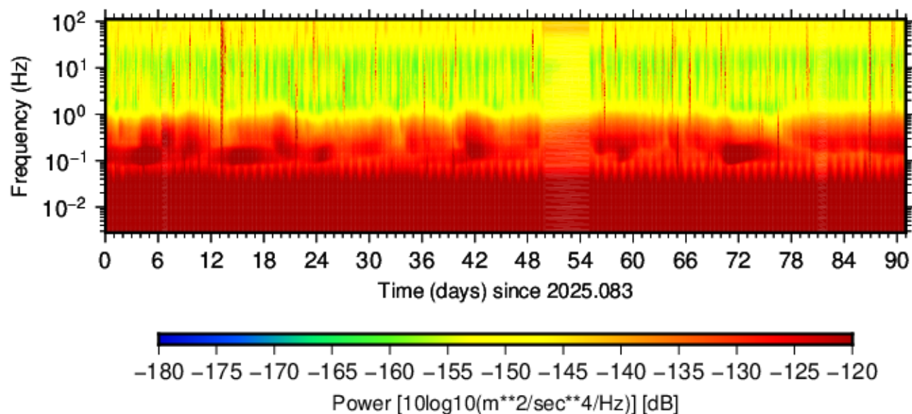
BP.CCRB.DP3.40 (2025.083 - 2025.173)
