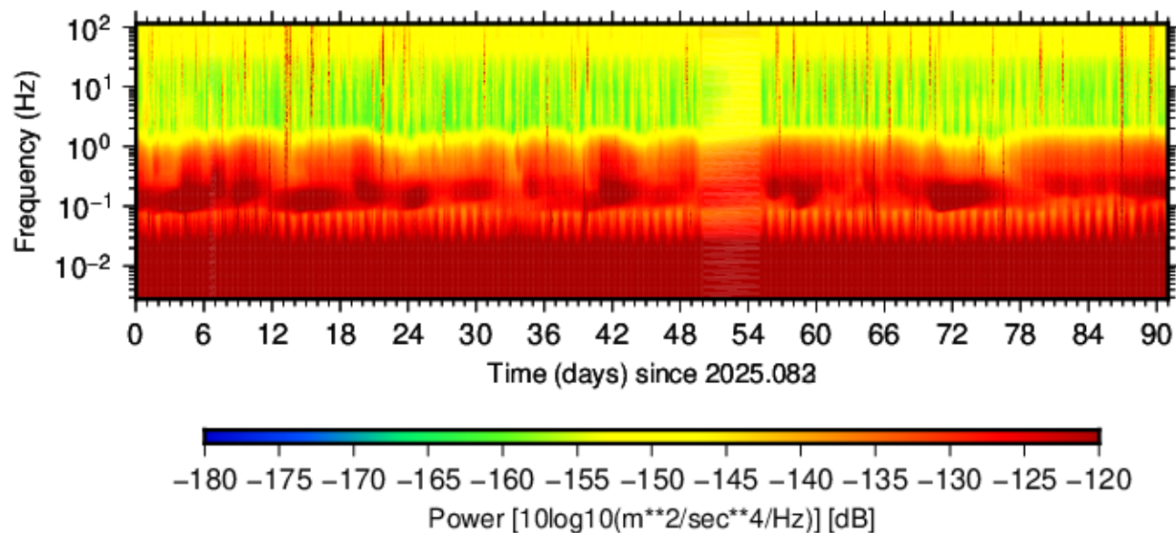
BP.CCRB.DP1.40 (2025.083 - 2025.173)
