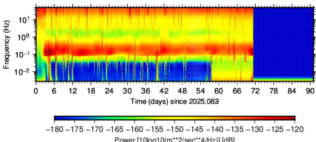
BK.BUCR.HHZ.00 (2025.083 - 2025.173)
