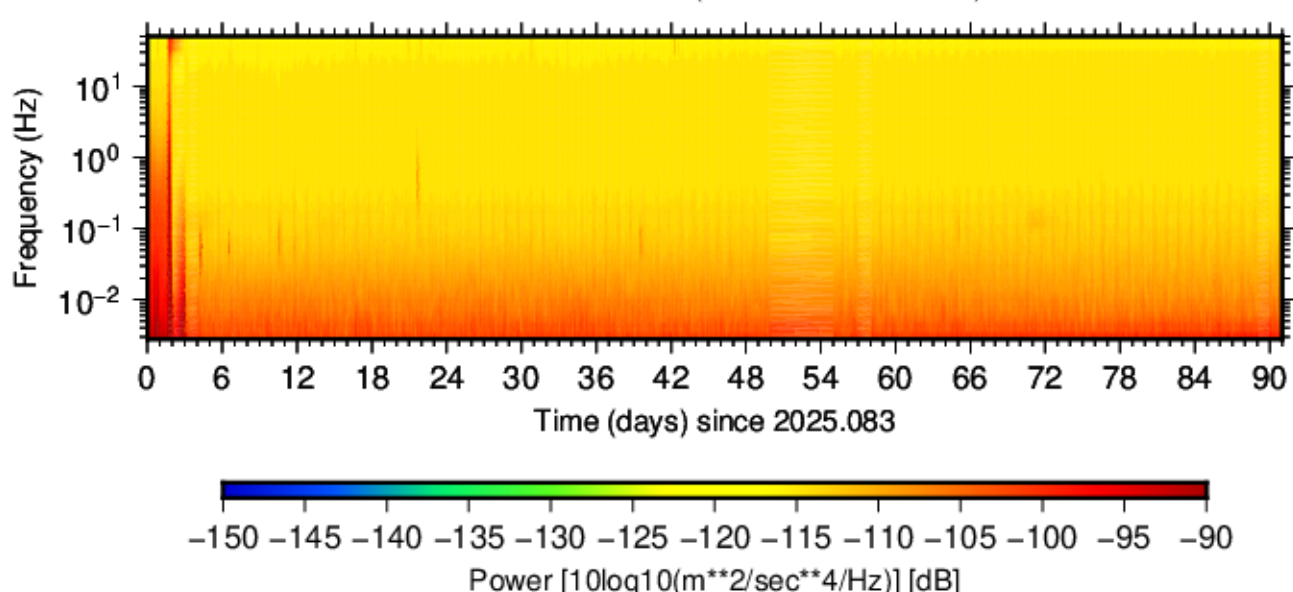
BK.BUCR.HNZ.00 (2025.083 - 2025.173)
