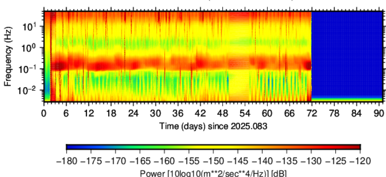
BK.BUCR.HHN.00 (2025.083 - 2025.173)
