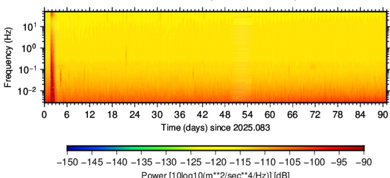
BK.BUCR.HNN.00 (2025.083 - 2025.173)
