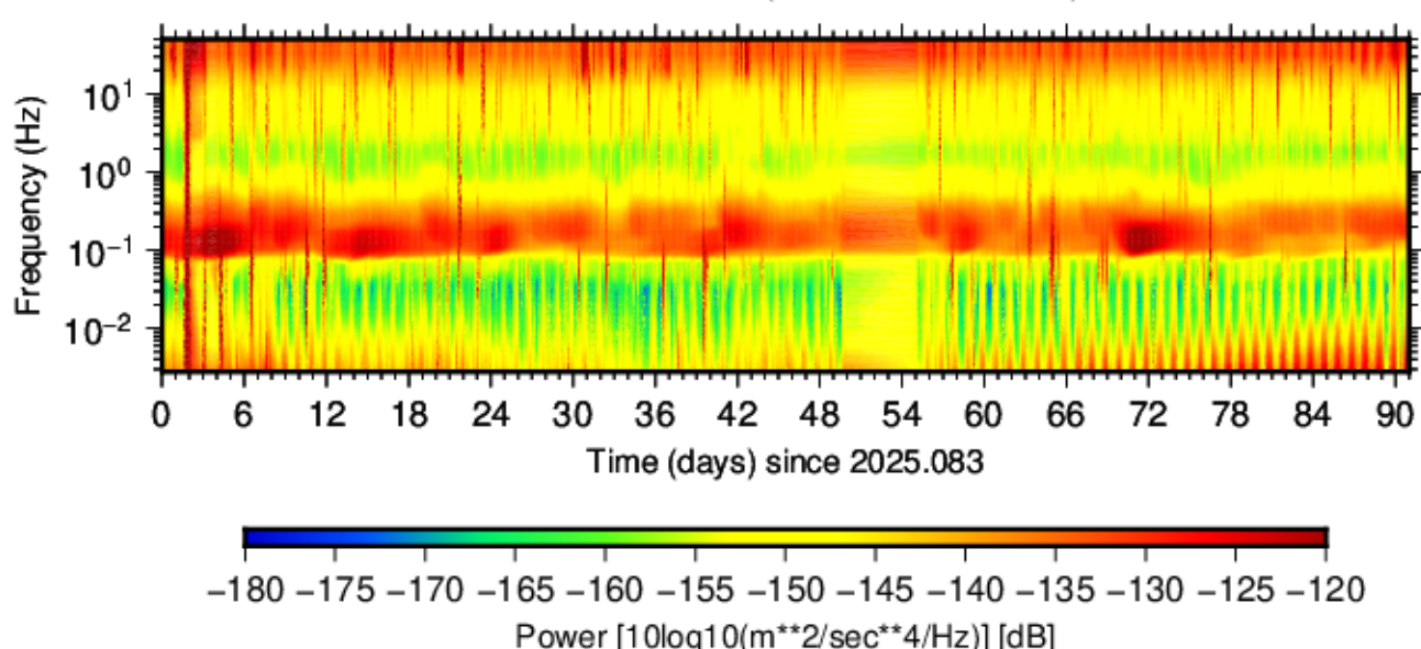
BK.BUCR.HHE.00 (2025.083 - 2025.173)
