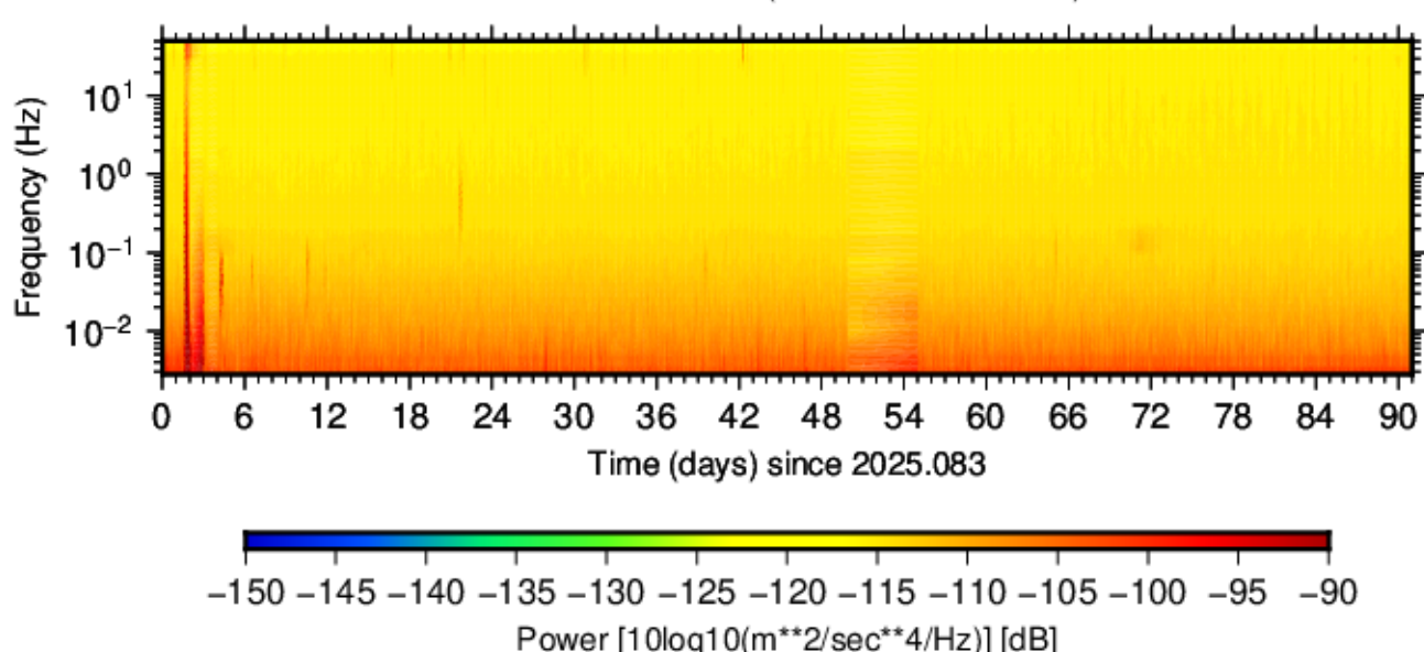
BK.BUCR.HNE.00 (2025.083 - 2025.173)
