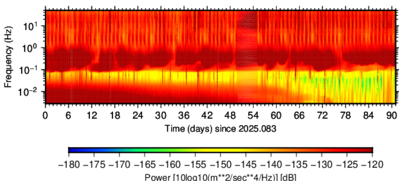
BK.BUCI.HHN.00 (2025.083 - 2025.173)
