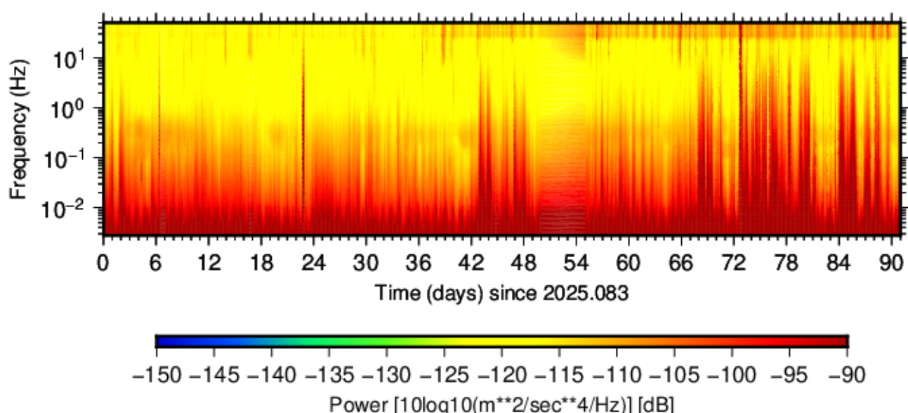
BK.BUCI.HNZ.00 (2025.083 - 2025.173)
