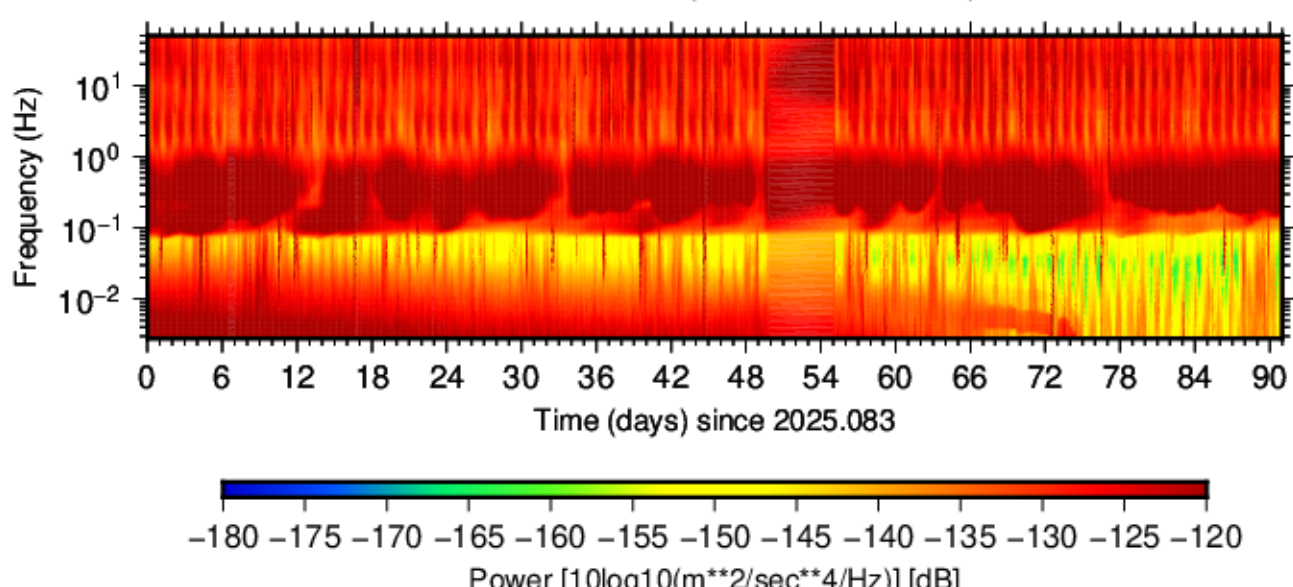
BK.BUCI.HHE.00 (2025.083 - 2025.173)
