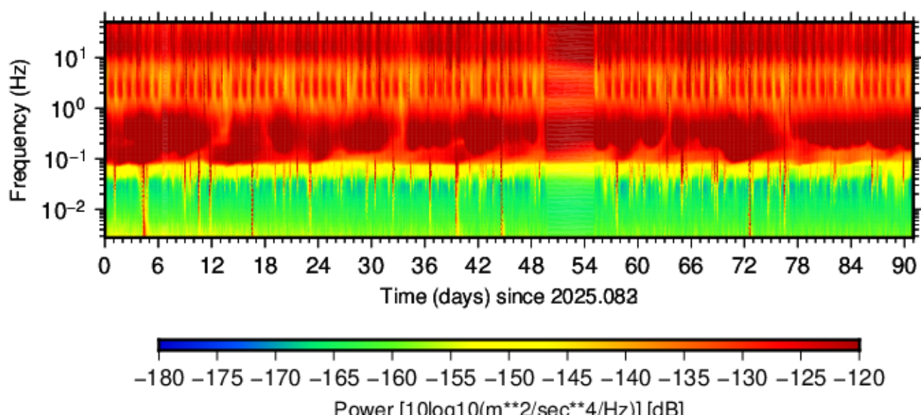
BK.BUCI.HHZ.00 (2025.083 - 2025.173)
