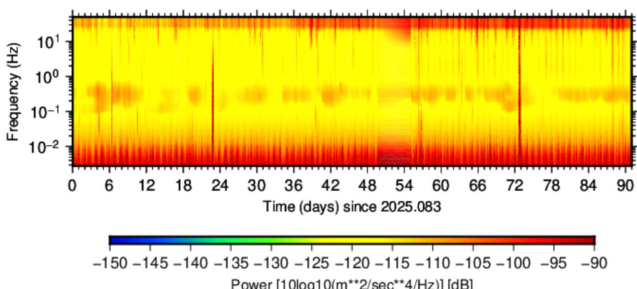
BK.BUCI.HNN.00 (2025.083 - 2025.173)
