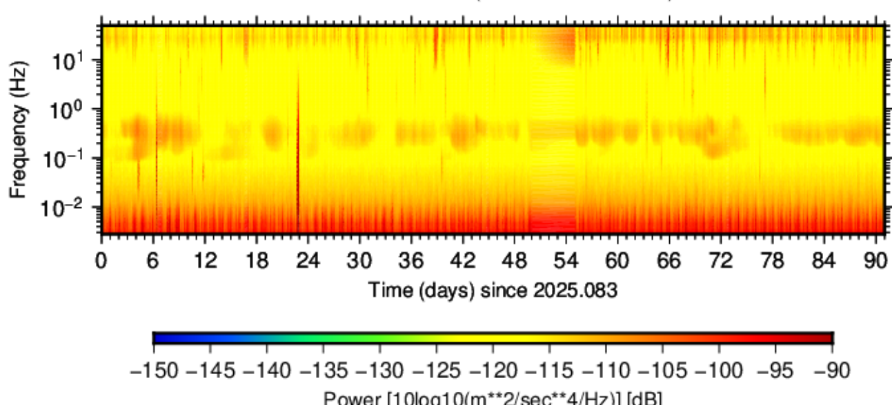
BK.BUCI.HNE.00 (2025.083 - 2025.173)
