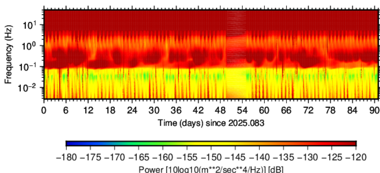
BK.BRK.HHN.00 (2025.083 - 2025.173)
