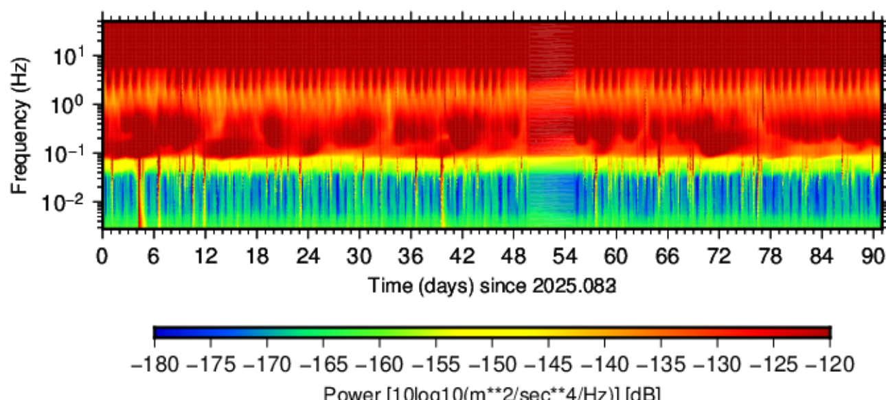
BK.BRK.HHZ.00 (2025.083 - 2025.173)
