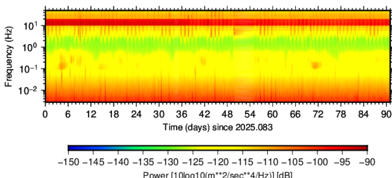
BK.BRK.HNN.00 (2025.083 - 2025.173)
