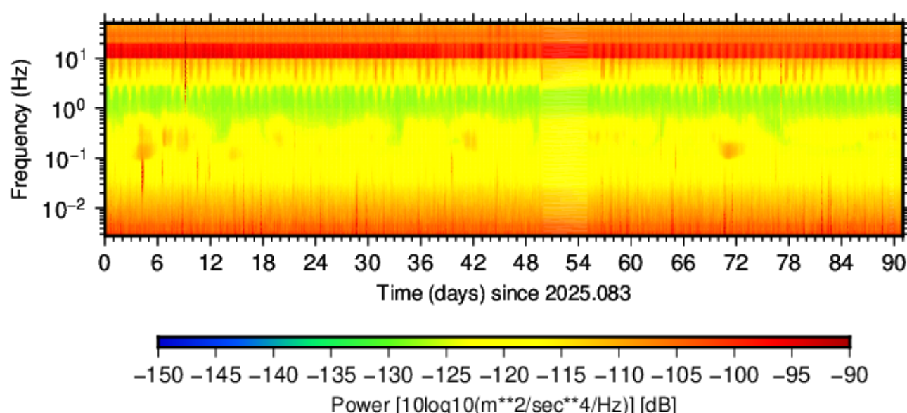
BK.BRK.HNE.00 (2025.083 - 2025.173)
