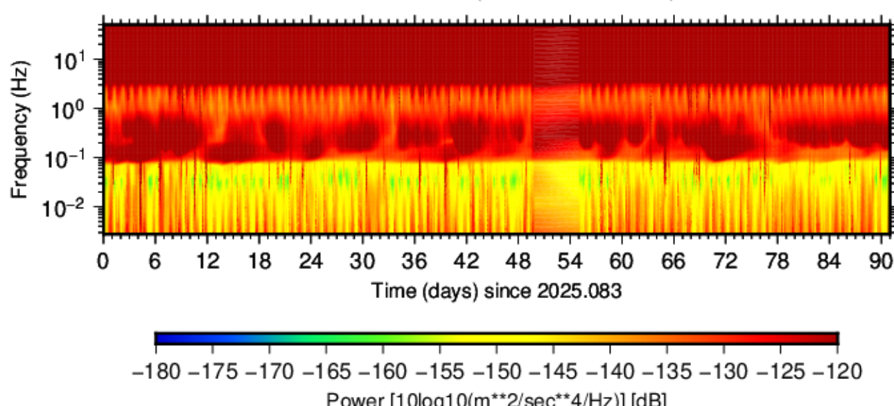
BK.BRK.HHE.00 (2025.083 - 2025.173)
