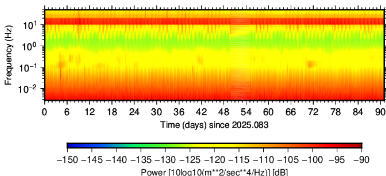
BK.BRK.HNZ.00 (2025.083 - 2025.173)
