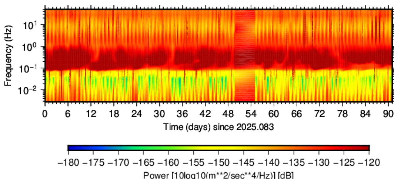
BK.BRIB.HHE.01 (2025.083 - 2025.173)
