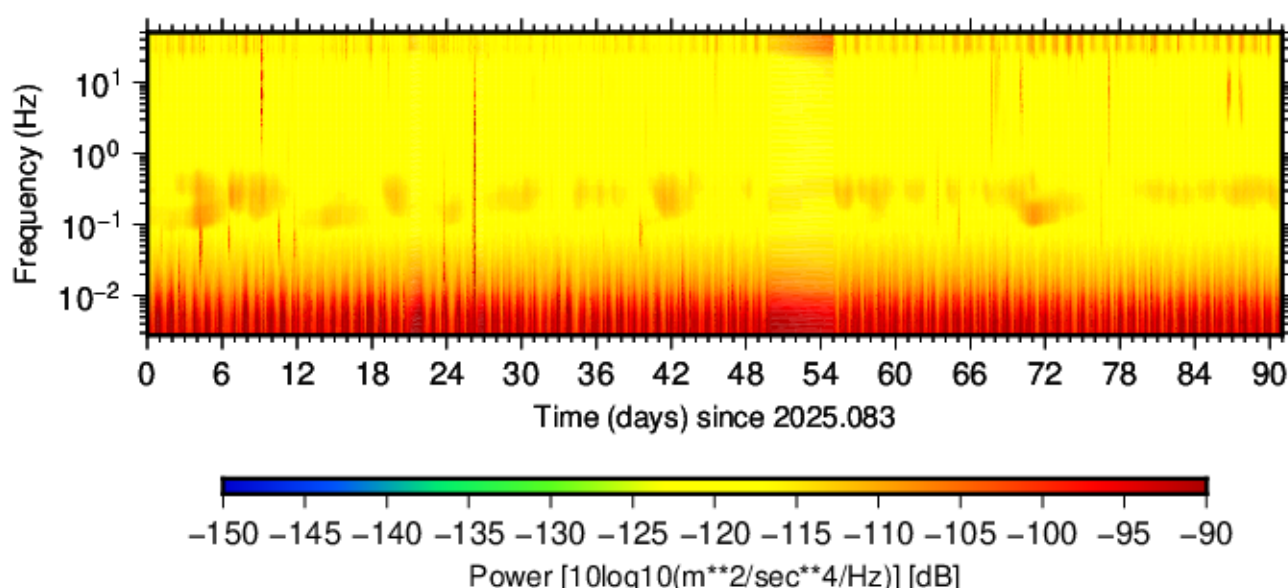
BK.BRIB.HNZ.01 (2025.083 - 2025.173)
