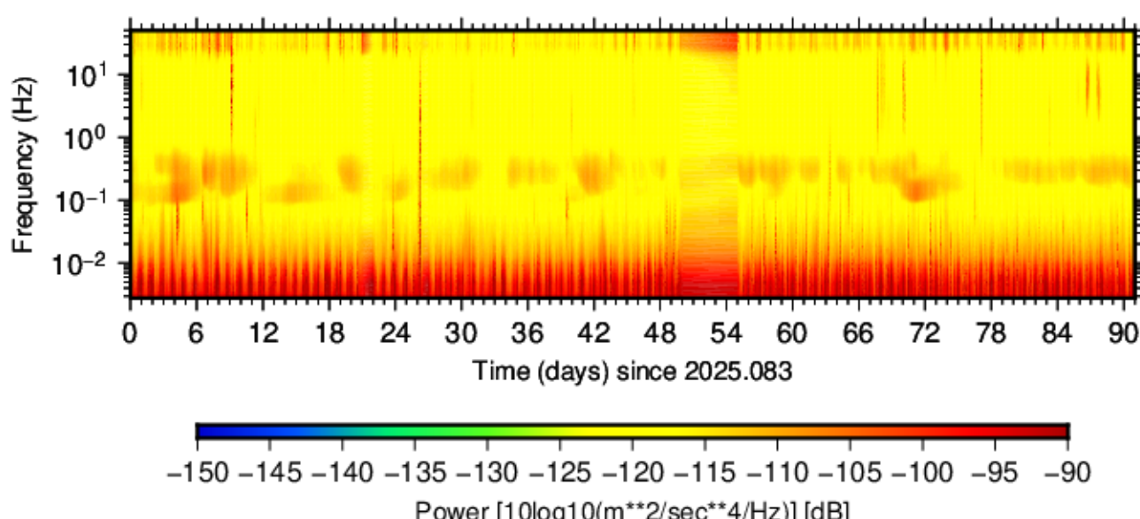
BK.BRIB.HNN.01 (2025.083 - 2025.173)
