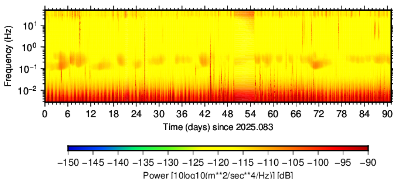
BK.BRIB.HNE.01 (2025.083 - 2025.173)
