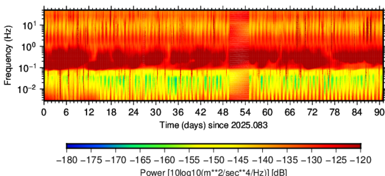
BK.BRIB.HHN.01 (2025.083 - 2025.173)
