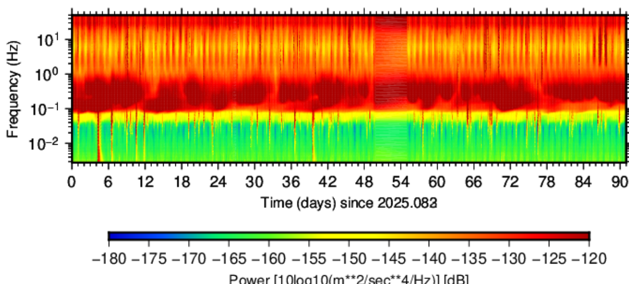
BK.BRIB.HHZ.01 (2025.083 - 2025.173)
