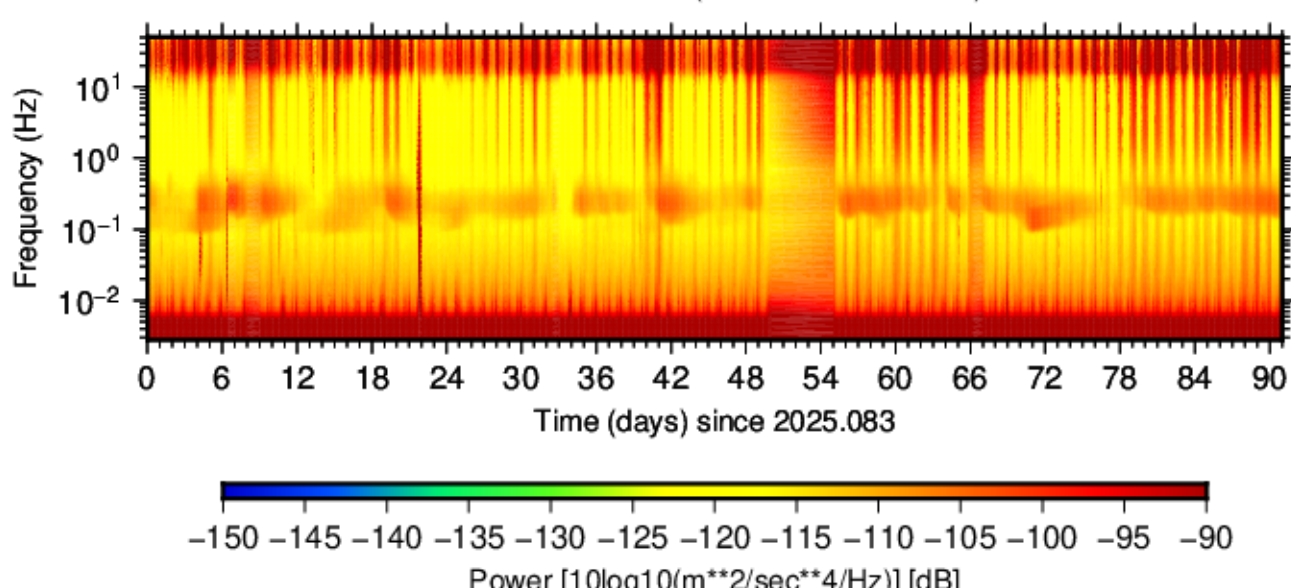
BK.BRAD.HNE.00 (2025.083 - 2025.173)
