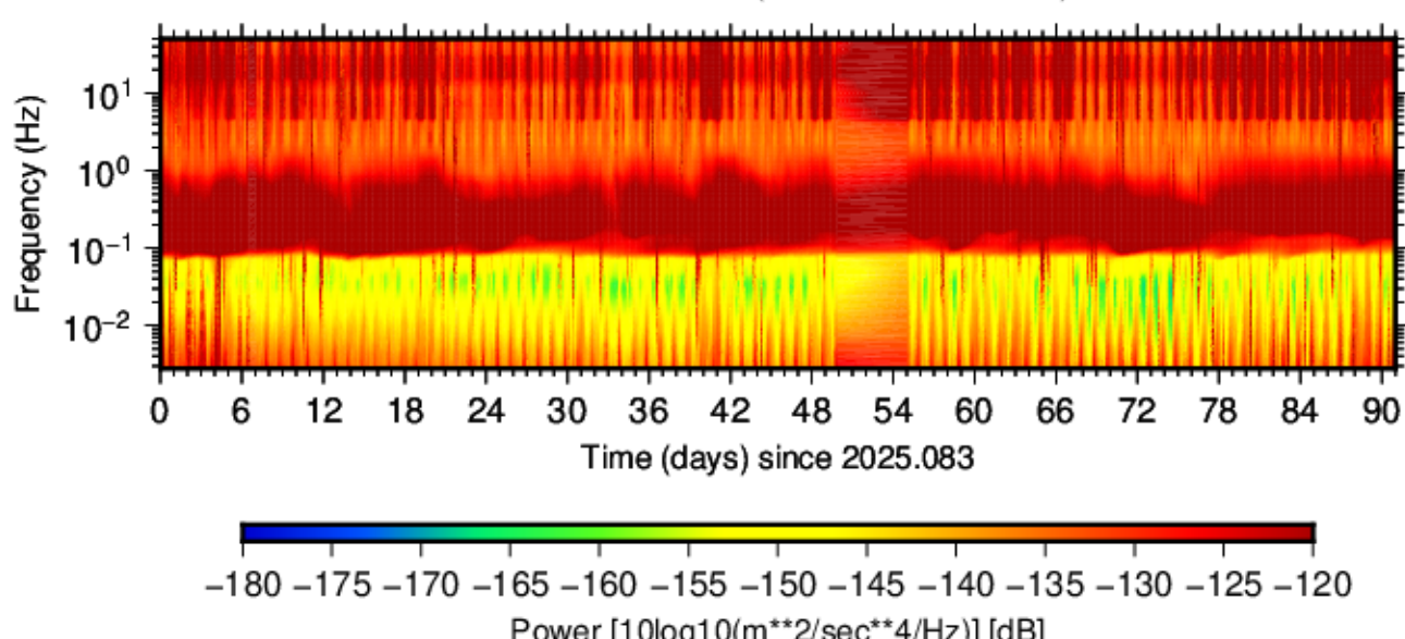
BK.BRAD.HHE.00 (2025.083 - 2025.173)
