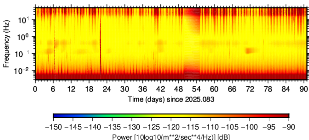
BK.BRAD.HNZ.00 (2025.083 - 2025.173)
