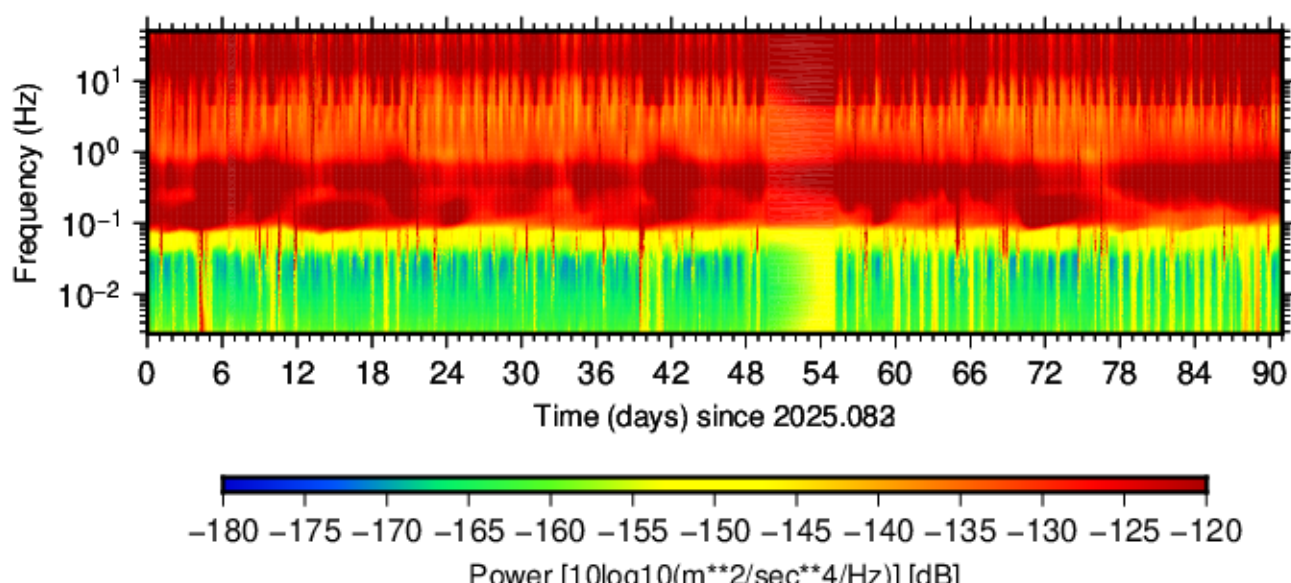
BK.BRAD.HHZ.00 (2025.083 - 2025.173)
