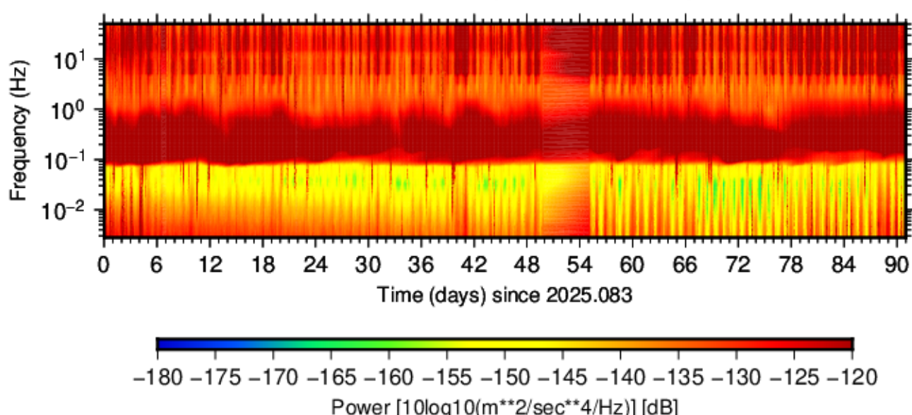
BK.BRAD.HHN.00 (2025.083 - 2025.173)
