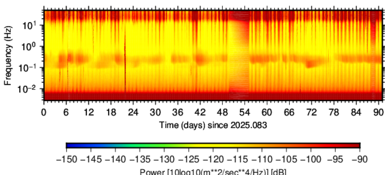
BK.BRAD.HNN.00 (2025.083 - 2025.173)
