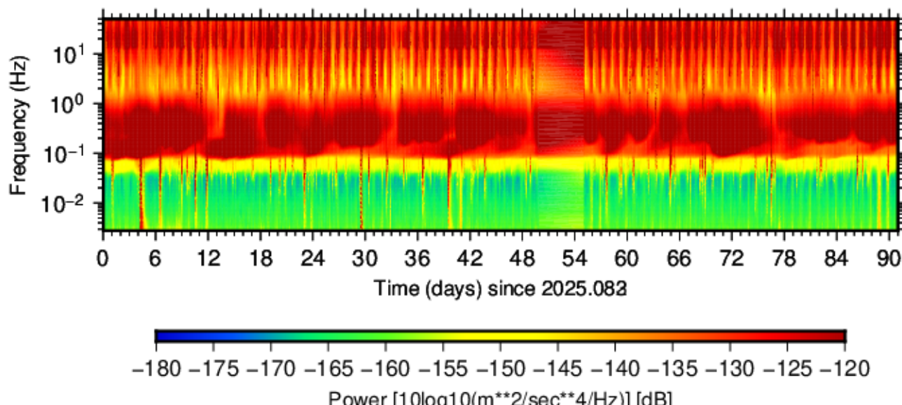
BK.BONV.HHZ.00 (2025.083 - 2025.173)
