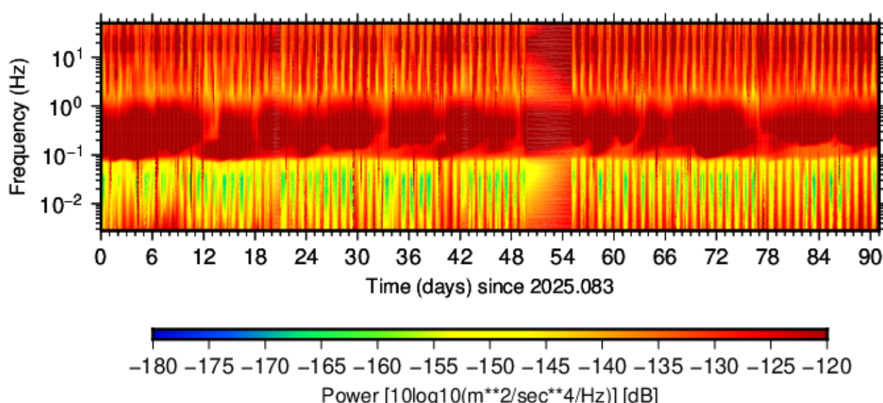
BK.BONV.HHN.00 (2025.083 - 2025.173)
