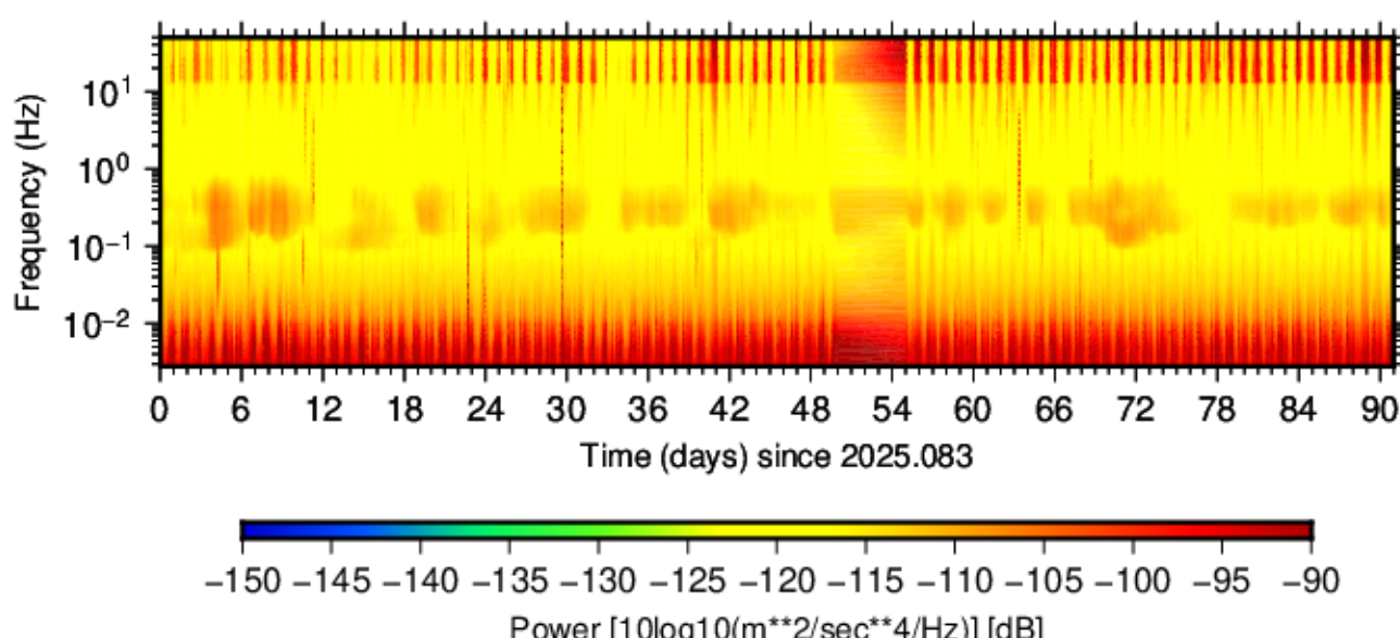
BK.BONV.HNN.00 (2025.083 - 2025.173)
