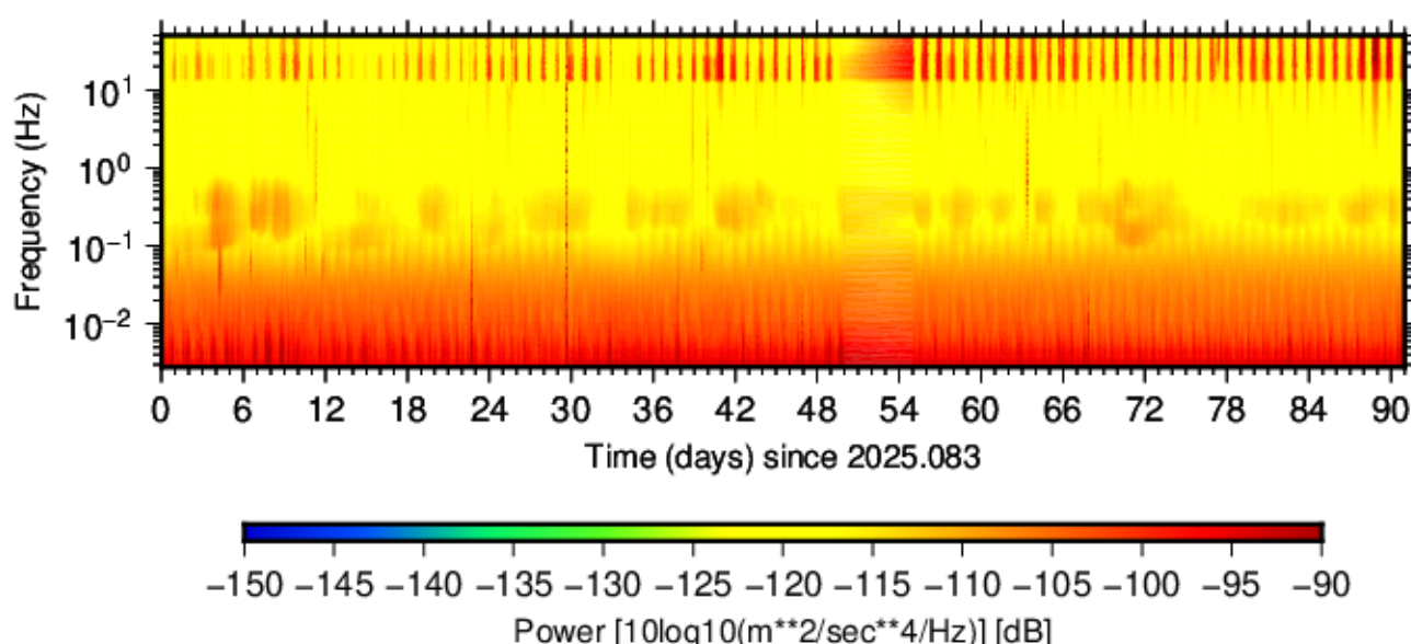
BK.BONV.HNZ.00 (2025.083 - 2025.173)
