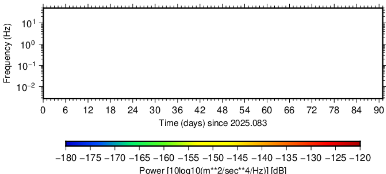
BK.BLUE.HHE.00 (2025.083 - 2025.173)
