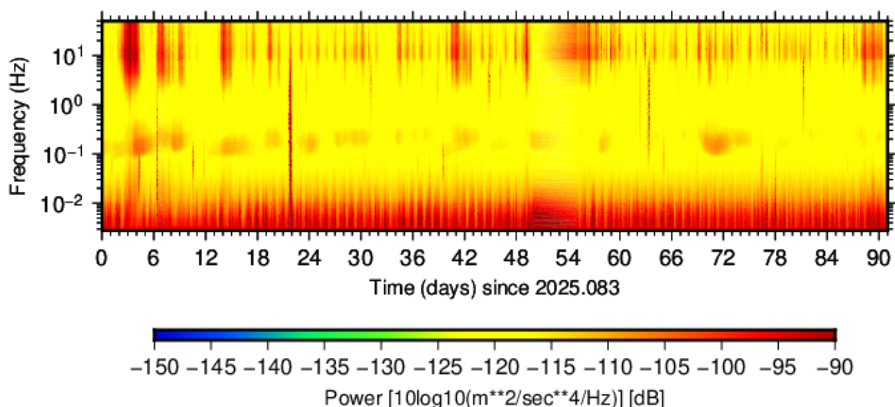
BK.BLAS.HNN.00 (2025.083 - 2025.173)
