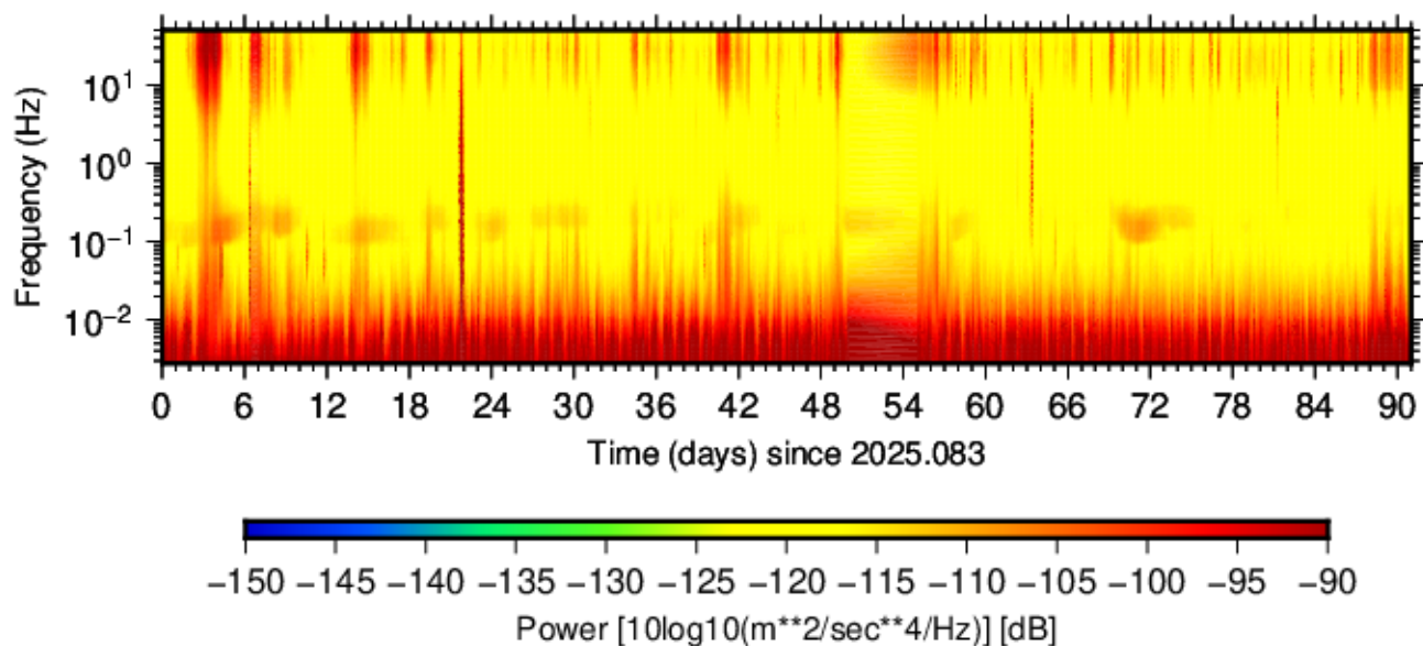
BK.BLAS.HNZ.00 (2025.083 - 2025.173)
