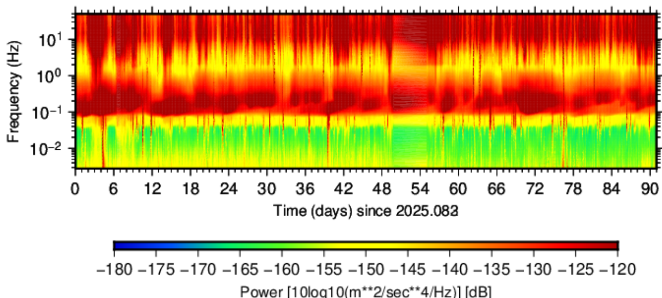
BK.BLAS.HHZ.00 (2025.083 - 2025.173)
