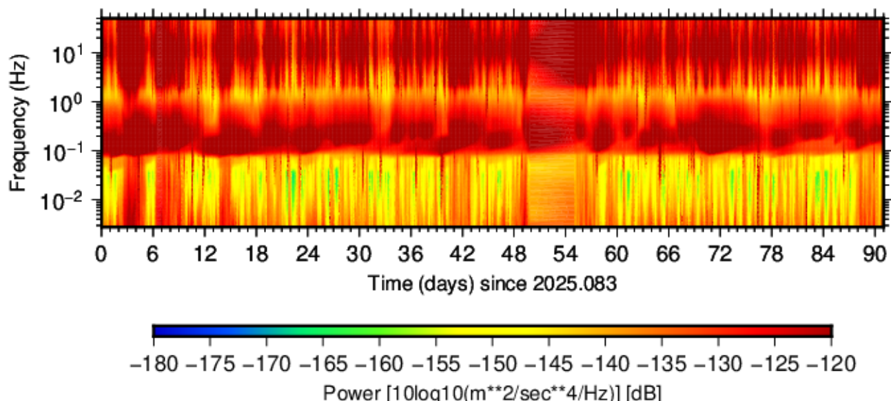
BK.BLAS.HHE.00 (2025.083 - 2025.173)
