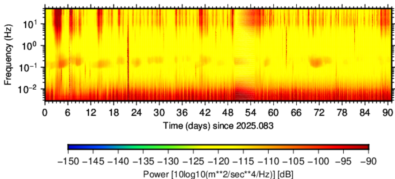
BK.BLAS.HNE.00 (2025.083 - 2025.173)
