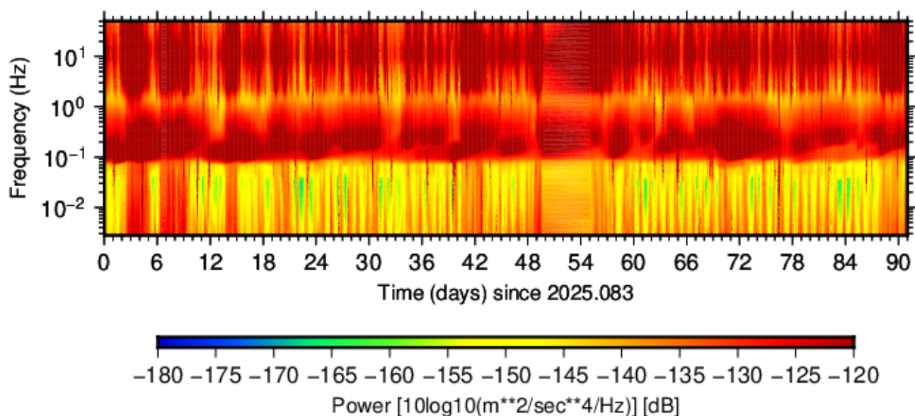
BK.BLAS.HHN.00 (2025.083 - 2025.173)
