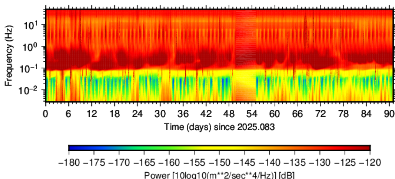
BK.BKS.HHE.00 (2025.083 - 2025.173)
