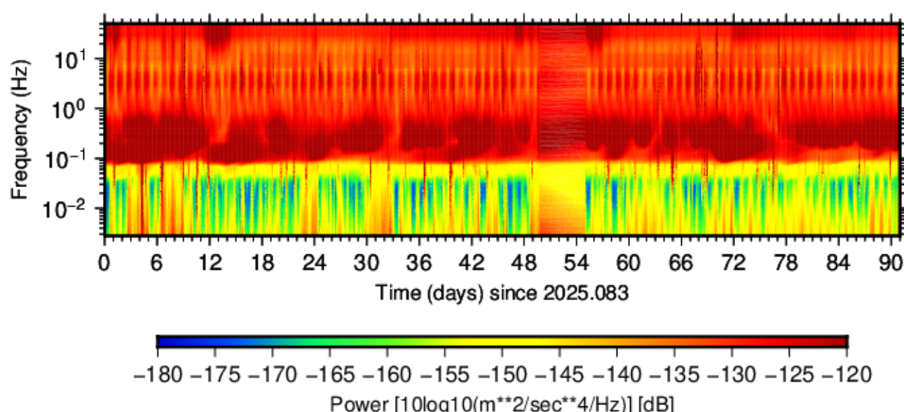
BK.BKS.HHN.00 (2025.083 - 2025.173)
