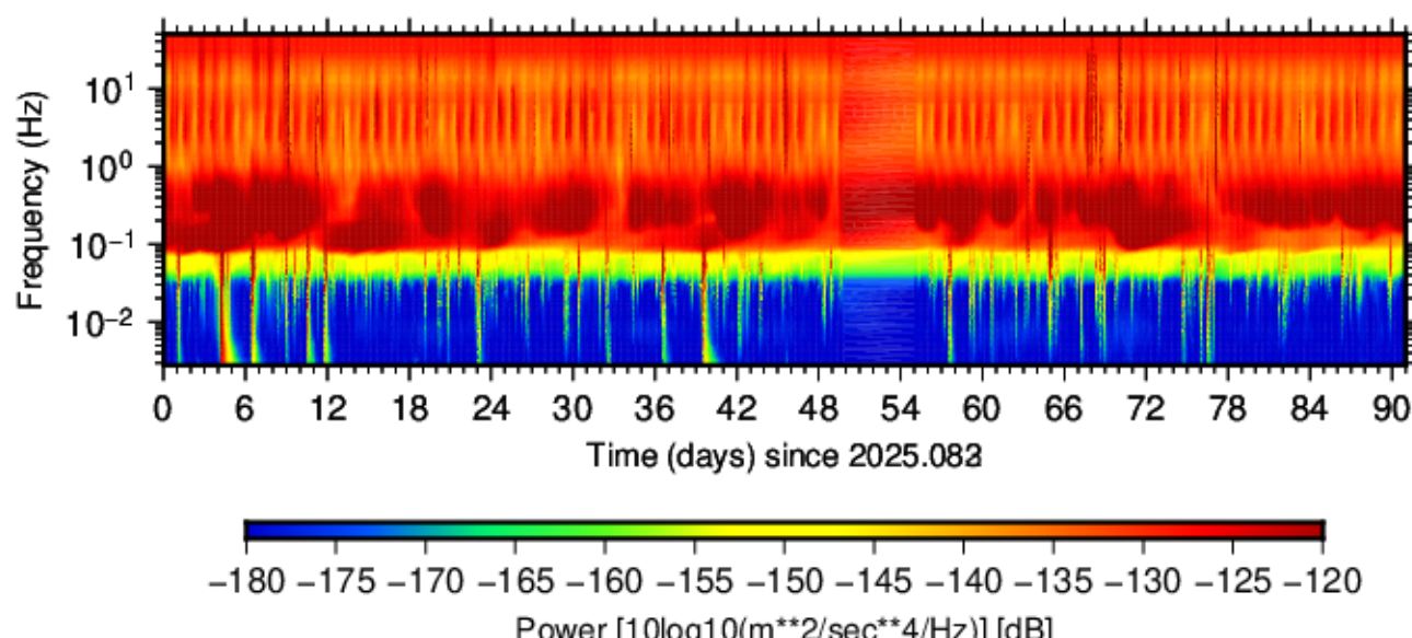
BK.BKS.HHZ.00 (2025.083 - 2025.173)
