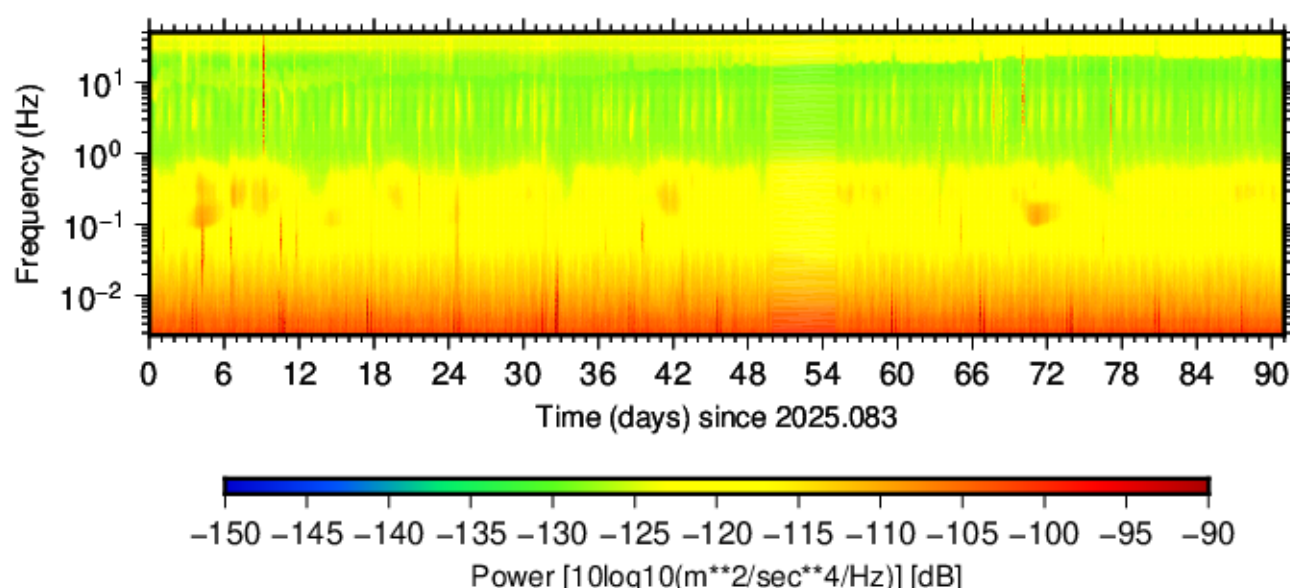
BK.BKS.HNZ.00 (2025.083 - 2025.173)
