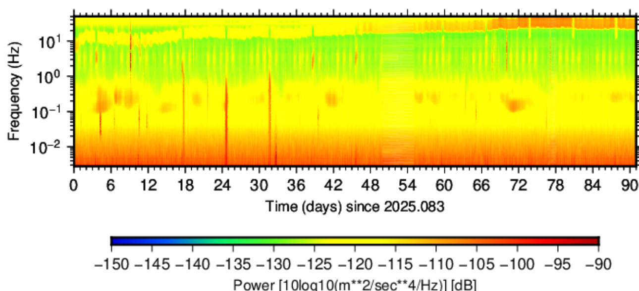
BK.BKS.HNE.00 (2025.083 - 2025.173)
