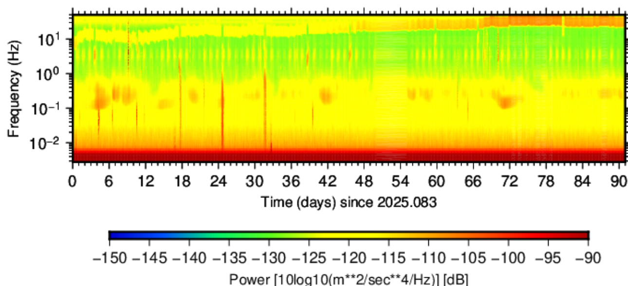
BK.BKS.HNN.00 (2025.083 - 2025.173)
