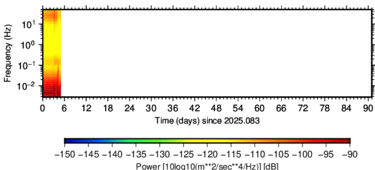
BK.BIGM.HNE.00 (2025.083 - 2025.173)
