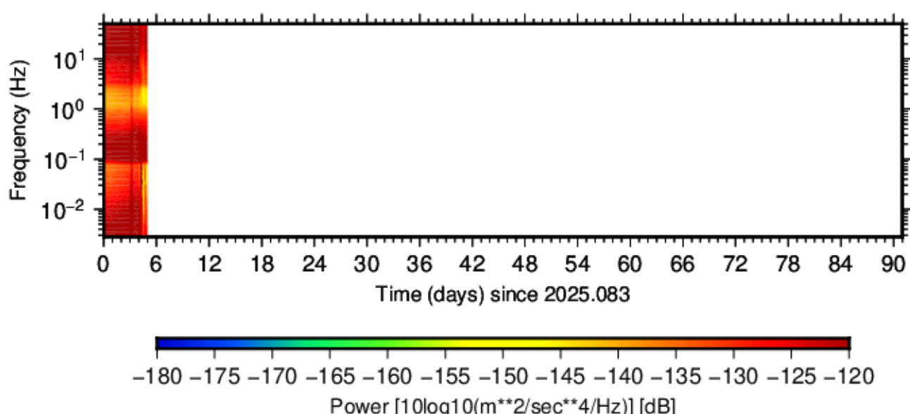
BK.BIGM.HHN.00 (2025.083 - 2025.173)
