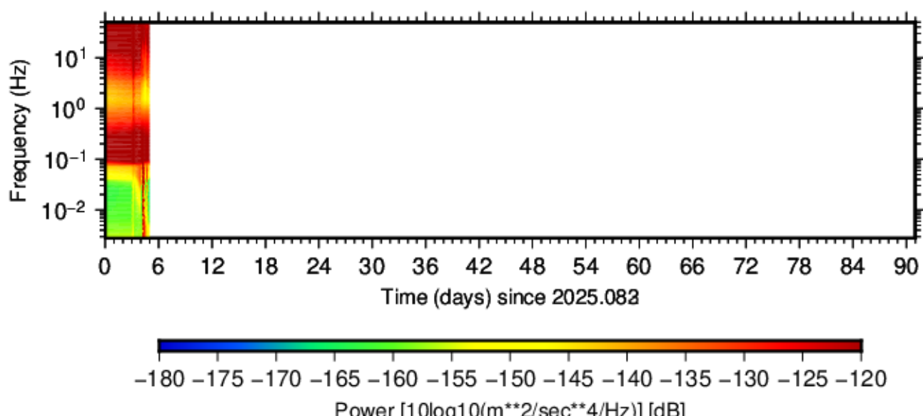
BK.BIGM.HHZ.00 (2025.083 - 2025.173)
