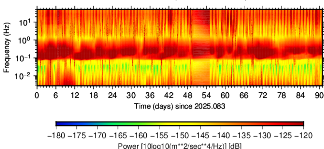
BK.BEVN.HHN.00 (2025.083 - 2025.173)
