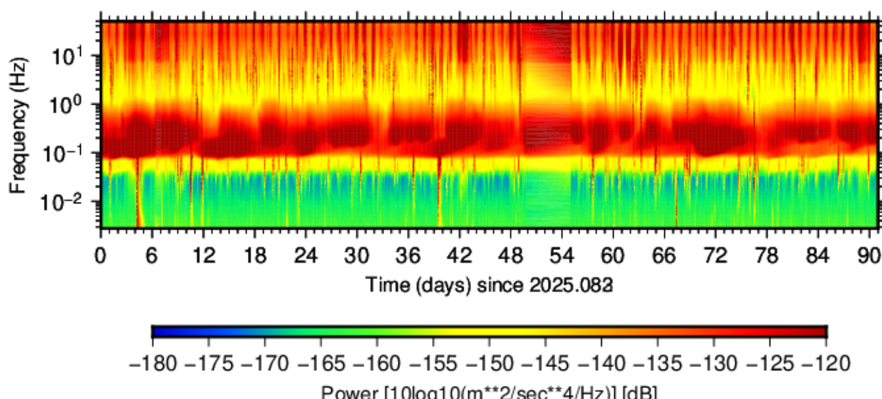
BK.BEVN.HHZ.00 (2025.083 - 2025.173)
