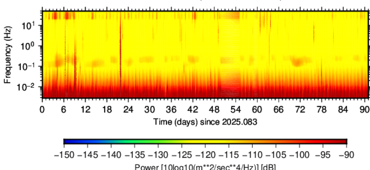
BK.BEVN.HNN.00 (2025.083 - 2025.173)
