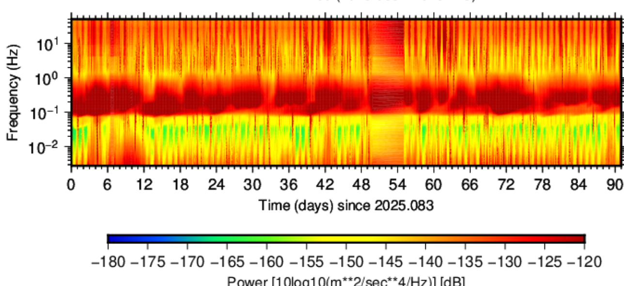
BK.BEVN.HHE.00 (2025.083 - 2025.173)
