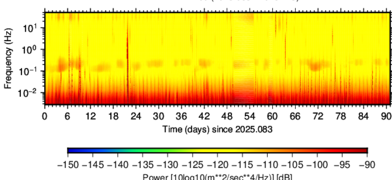
BK.BEVN.HNE.00 (2025.083 - 2025.173)
