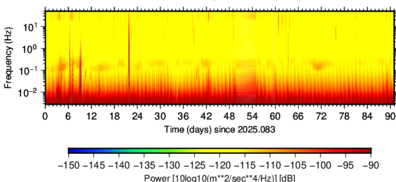
BK.BEVN.HNZ.00 (2025.083 - 2025.173)
