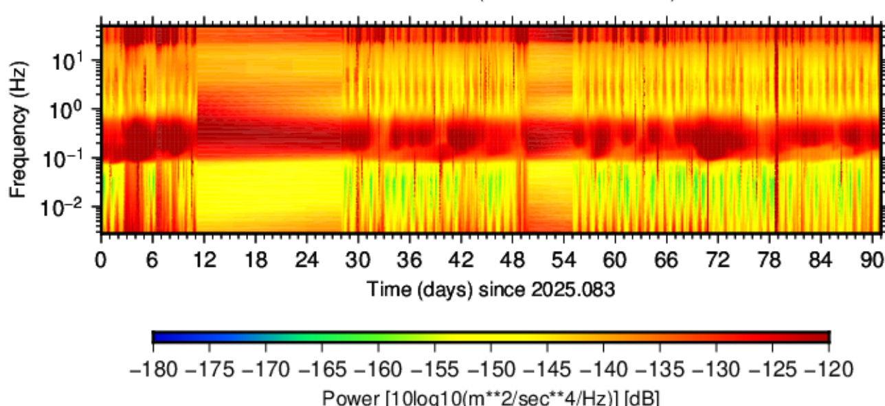
BK.BCCR.HHN.00 (2025.083 - 2025.173)
