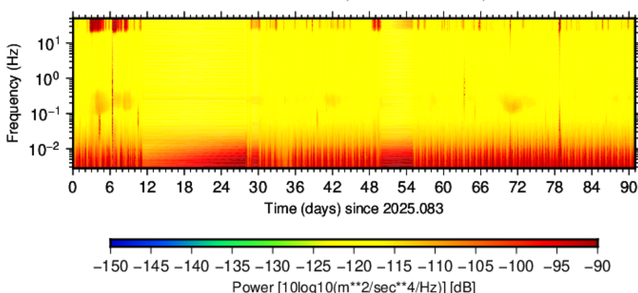
BK.BCCR.HNE.00 (2025.083 - 2025.173)
