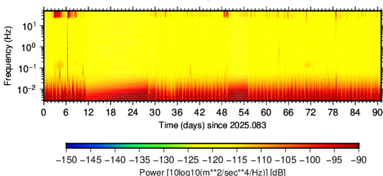
BK.BCCR.HNZ.00 (2025.083 - 2025.173)
