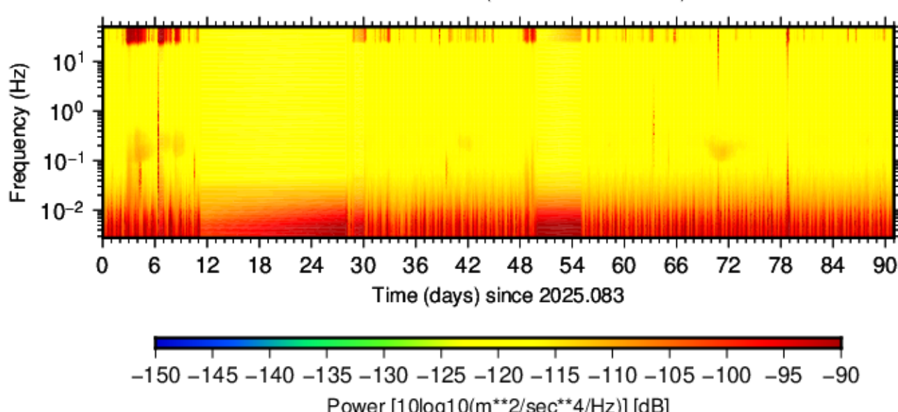
BK.BCCR.HNN.00 (2025.083 - 2025.173)
