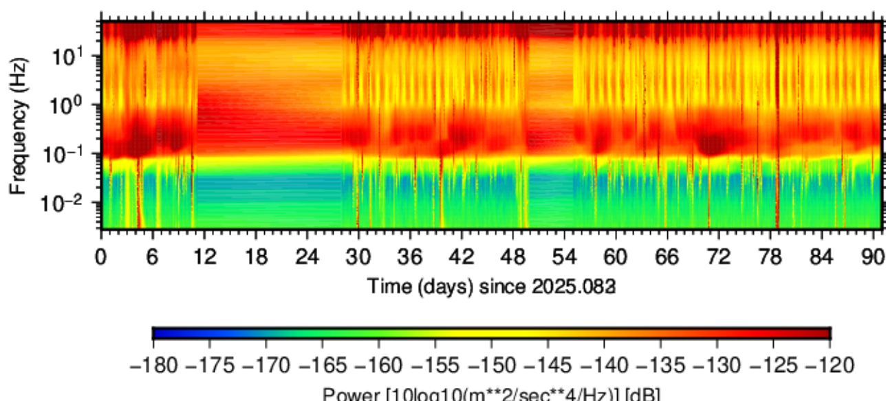
BK.BCCR.HHZ.00 (2025.083 - 2025.173)
