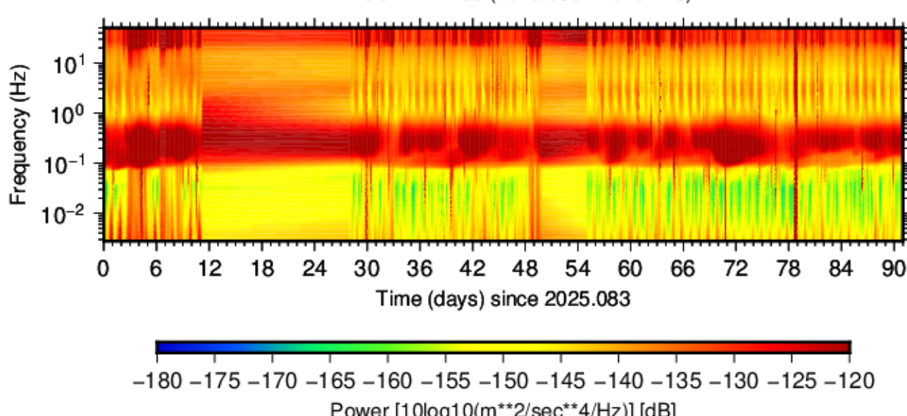
BK.BCCR.HHE.00 (2025.083 - 2025.173)
