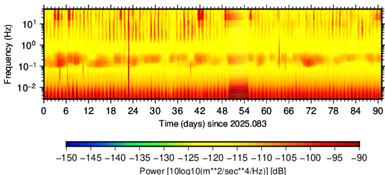
BK.BAYL.HNN.00 (2025.083 - 2025.173)
