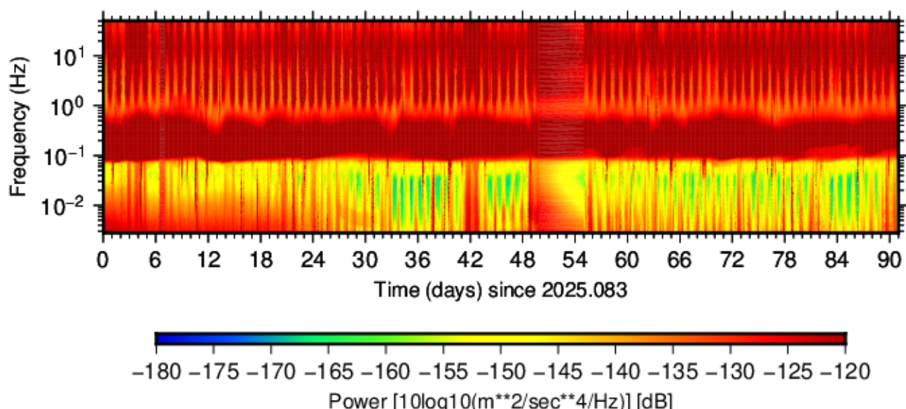
BK.BAYL.HHN.00 (2025.083 - 2025.173)
