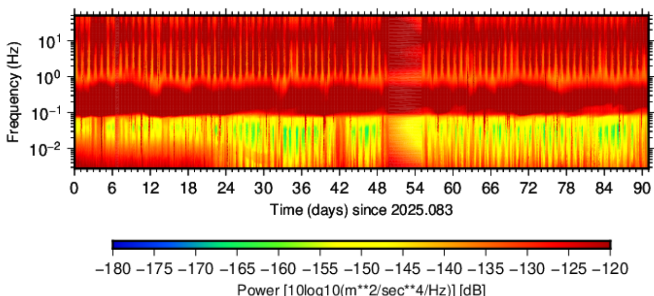
BK.BAYL.HHE.00 (2025.083 - 2025.173)
