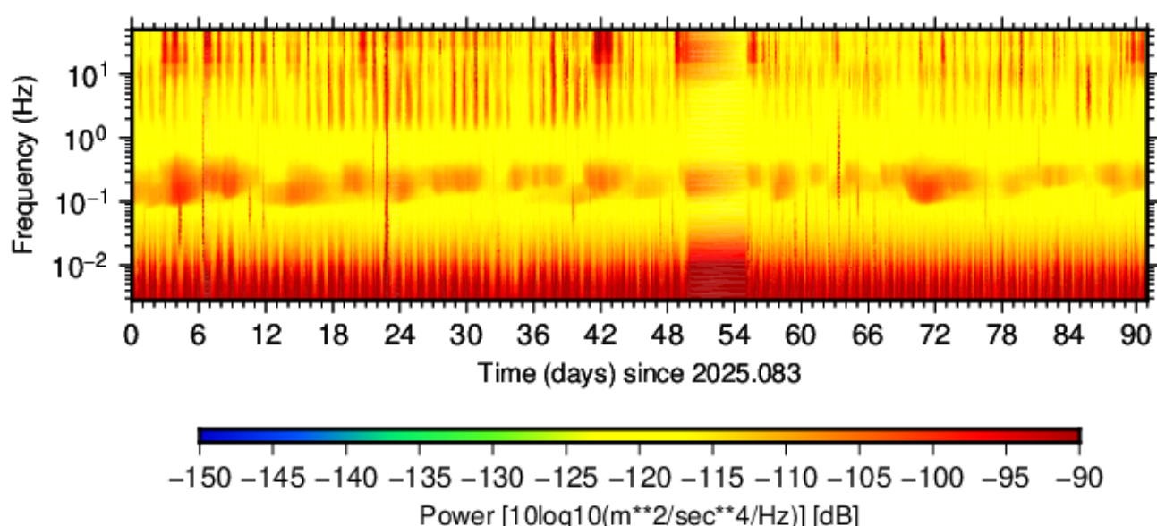
BK.BAYL.HNE.00 (2025.083 - 2025.173)
