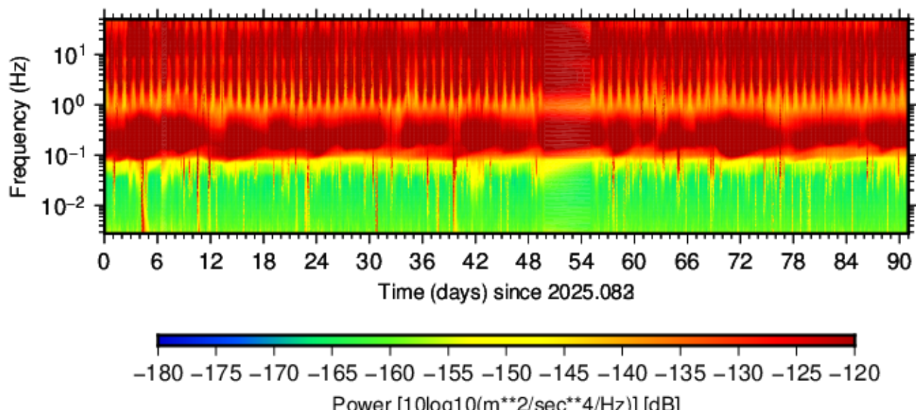
BK.BAYL.HHZ.00 (2025.083 - 2025.173)
