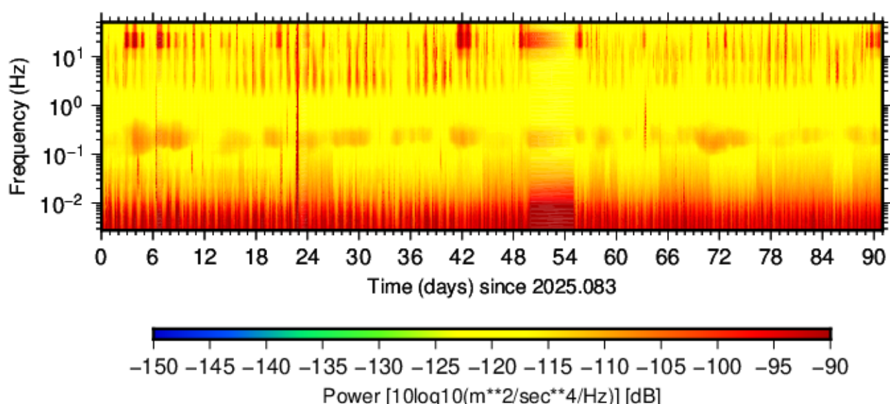
BK.BAYL.HNZ.00 (2025.083 - 2025.173)
