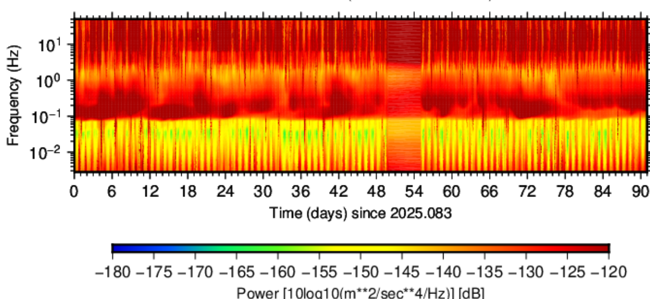
BK.BABI.HHN.00 (2025.083 - 2025.173)
