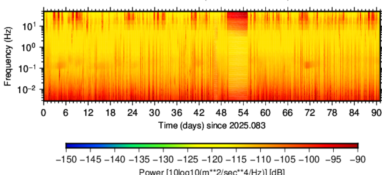
BK.BABI.HNN.00 (2025.083 - 2025.173)
