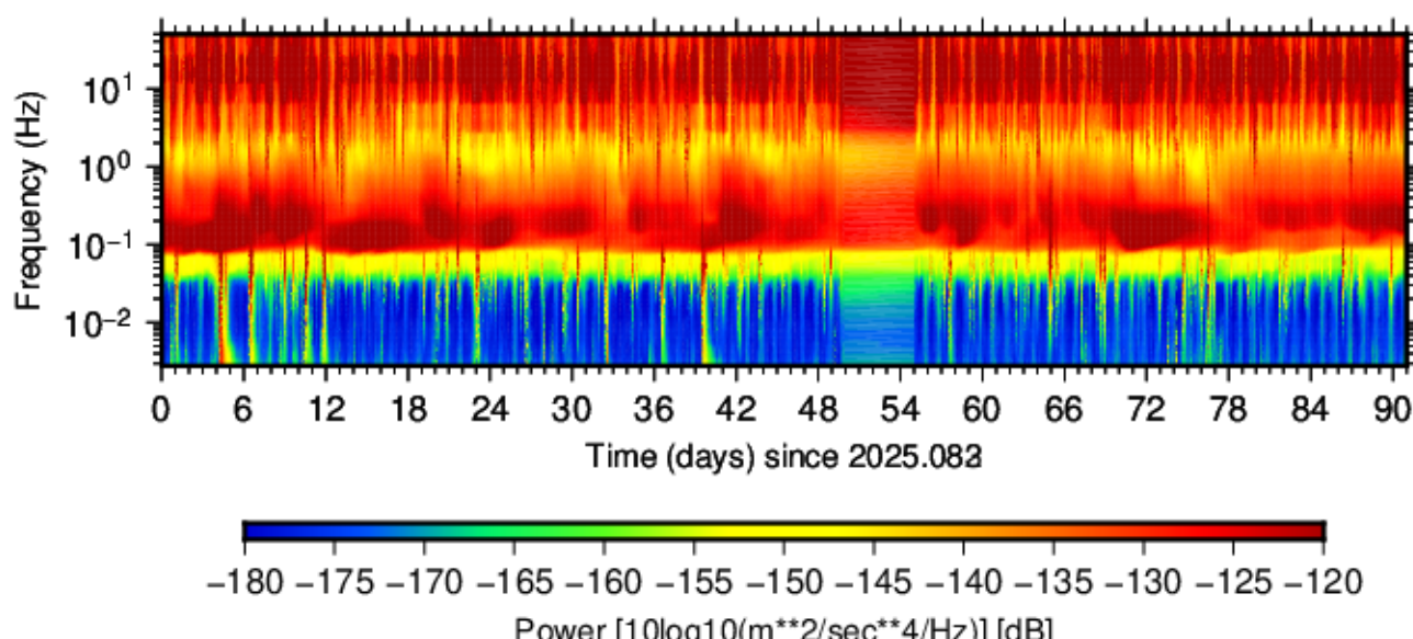
BK.BABI.HHZ.00 (2025.083 - 2025.173)
