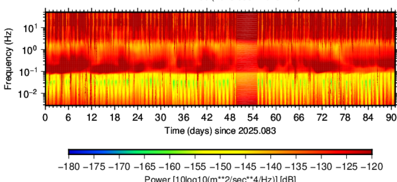
BK.BABI.HHE.00 (2025.083 - 2025.173)
