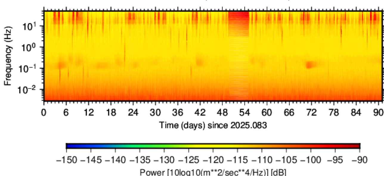
BK.BABI.HNE.00 (2025.083 - 2025.173)
