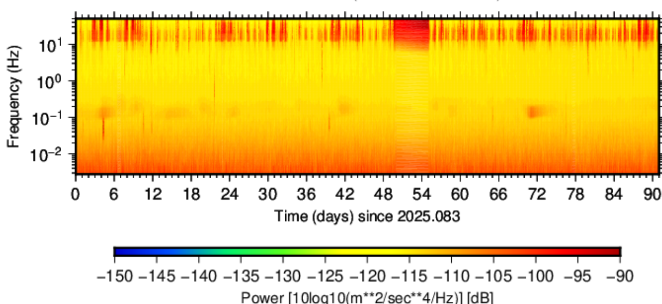
BK.BABI.HNZ.00 (2025.083 - 2025.173)
