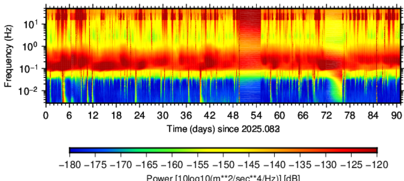
BK.AZUL.HHZ.00 (2025.083 - 2025.173)
