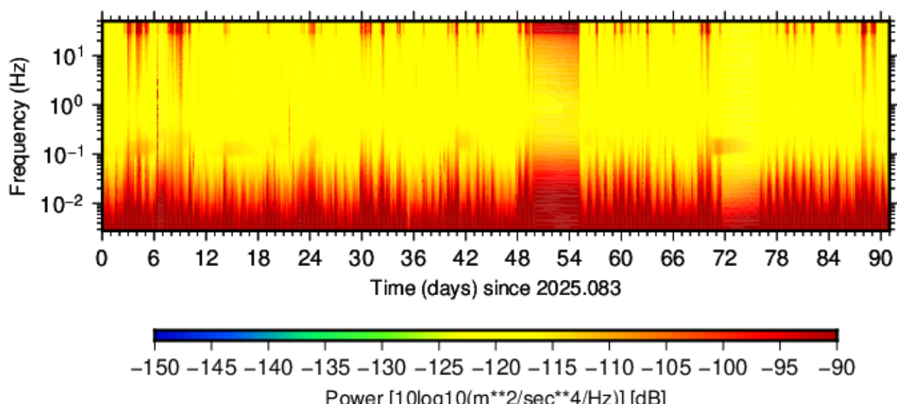
BK.AZUL.HNN.00 (2025.083 - 2025.173)
