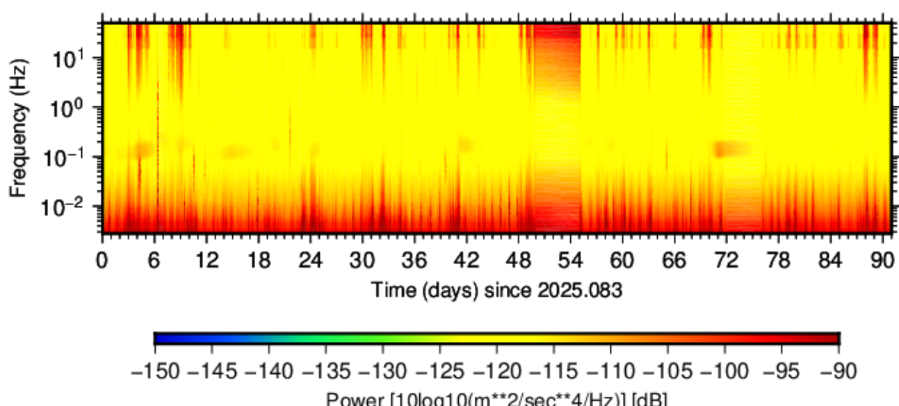
BK.AZUL.HNE.00 (2025.083 - 2025.173)
