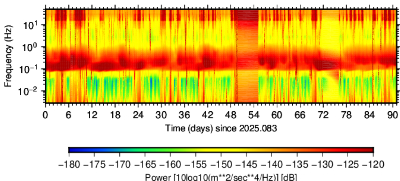
BK.AZUL.HHN.00 (2025.083 - 2025.173)
