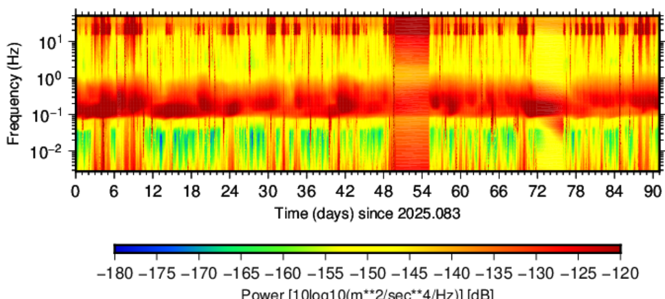
BK.AZUL.HHE.00 (2025.083 - 2025.173)
