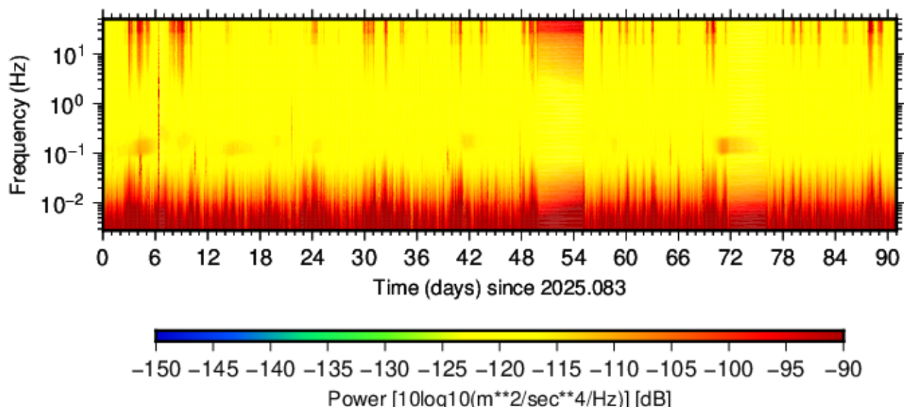
BK.AZUL.HNZ.00 (2025.083 - 2025.173)
