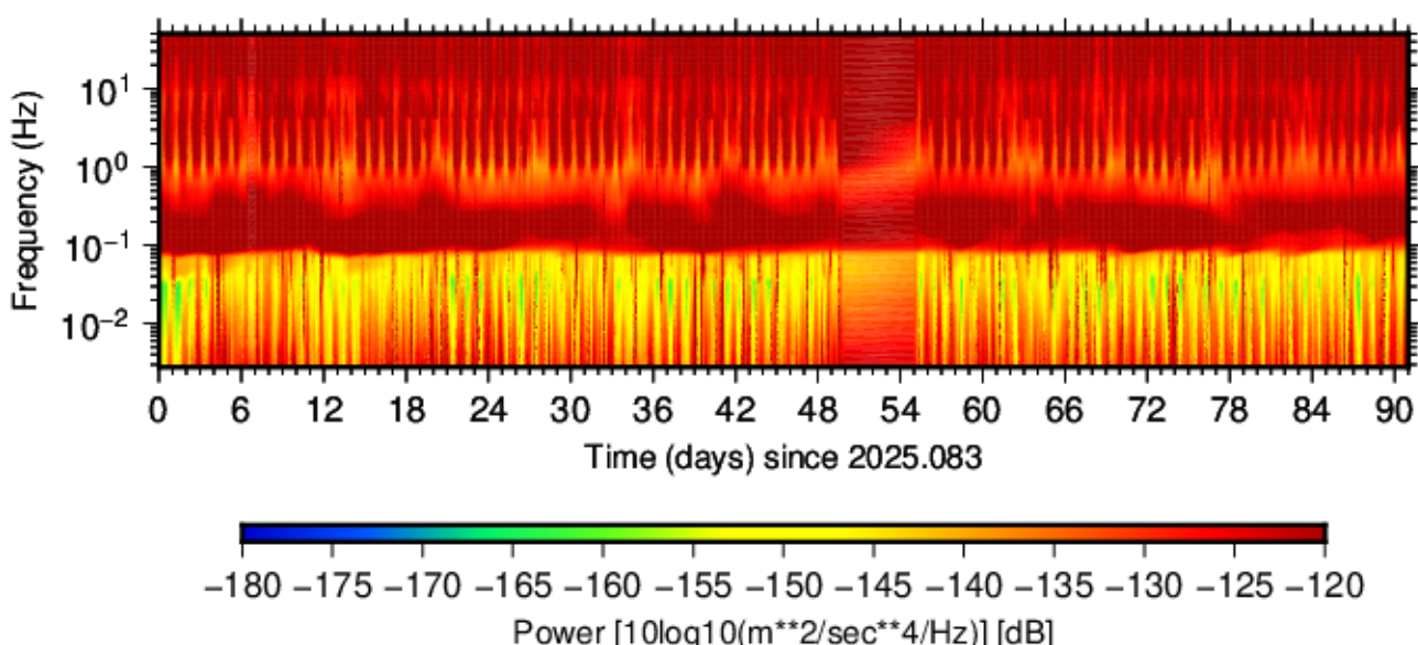
BK.AVSP.HHE.00 (2025.083 - 2025.173)
