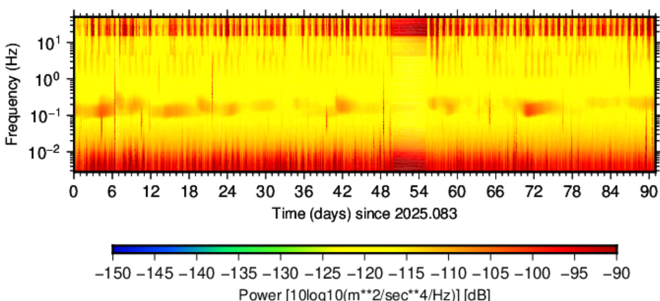
BK.AVSP.HNE.00 (2025.083 - 2025.173)
