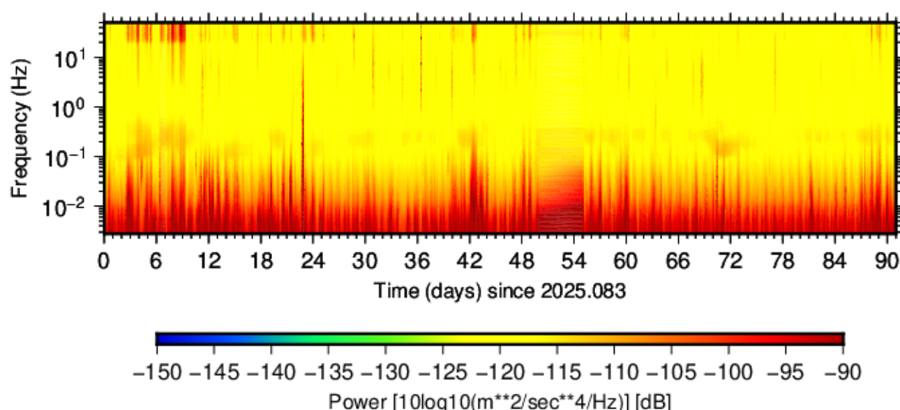
BK.ATP.HNZ.00 (2025.083 - 2025.173)
