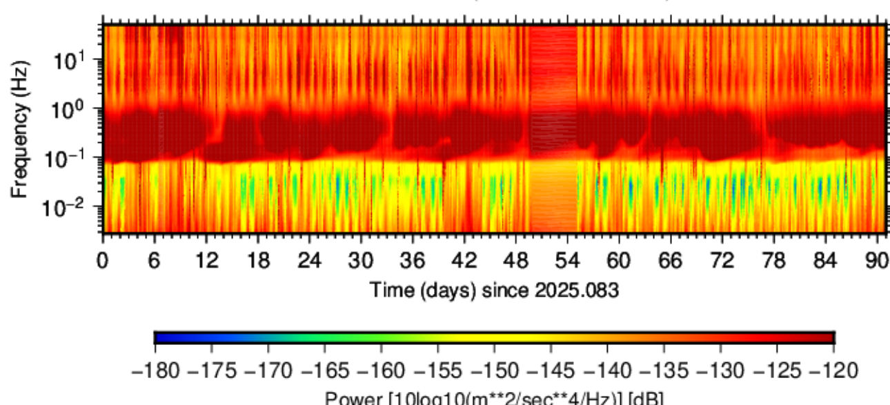
BK.ATP.HHE.00 (2025.083 - 2025.173)
