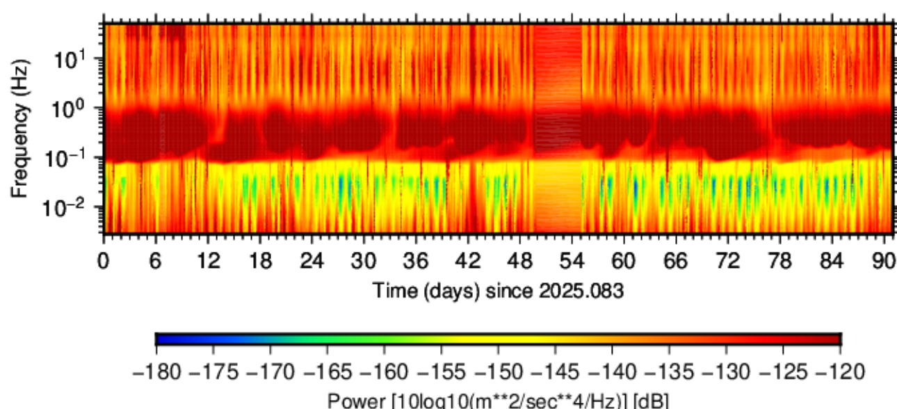
BK.ATP.HHN.00 (2025.083 - 2025.173)
