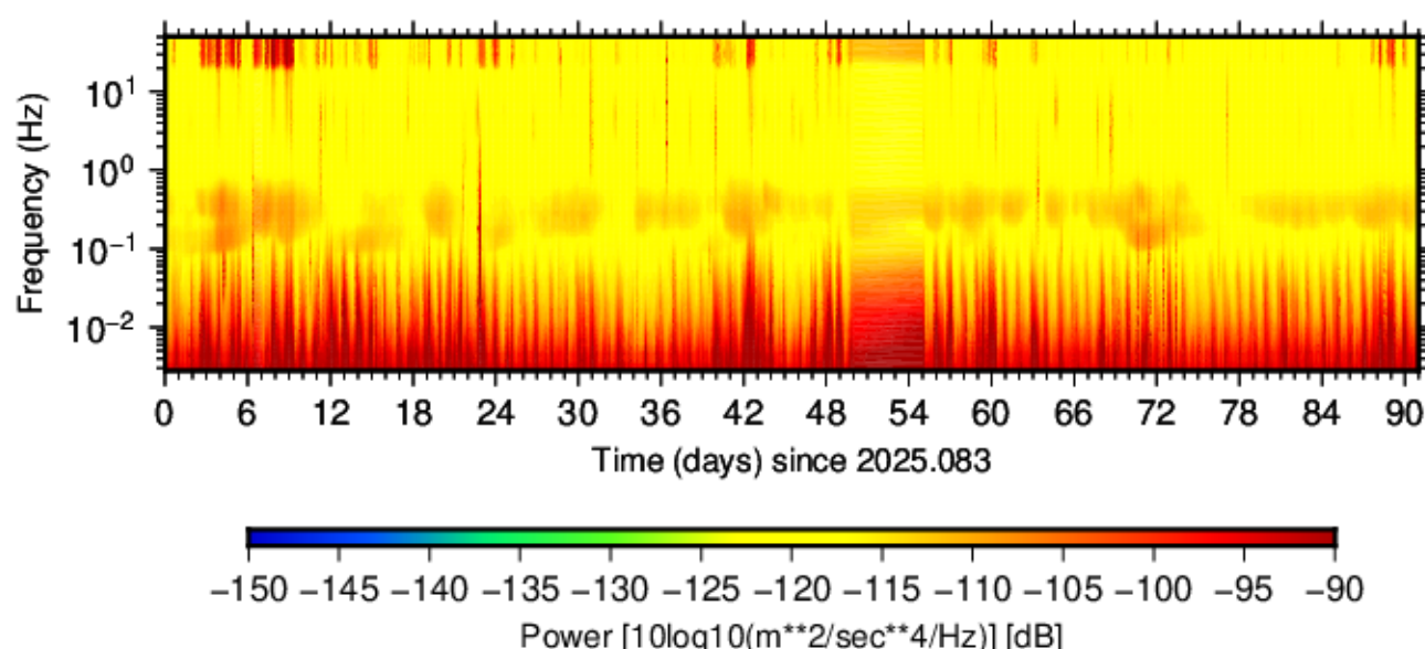
BK.ATP.HNE.00 (2025.083 - 2025.173)
