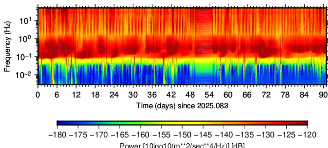
BK.ATP.HHZ.00 (2025.083 - 2025.173)
