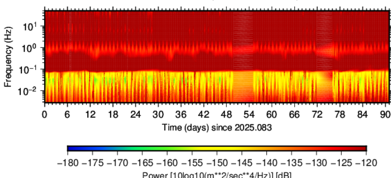
BK.AL VW.HHE.00 (2025.083 - 2025.173)
