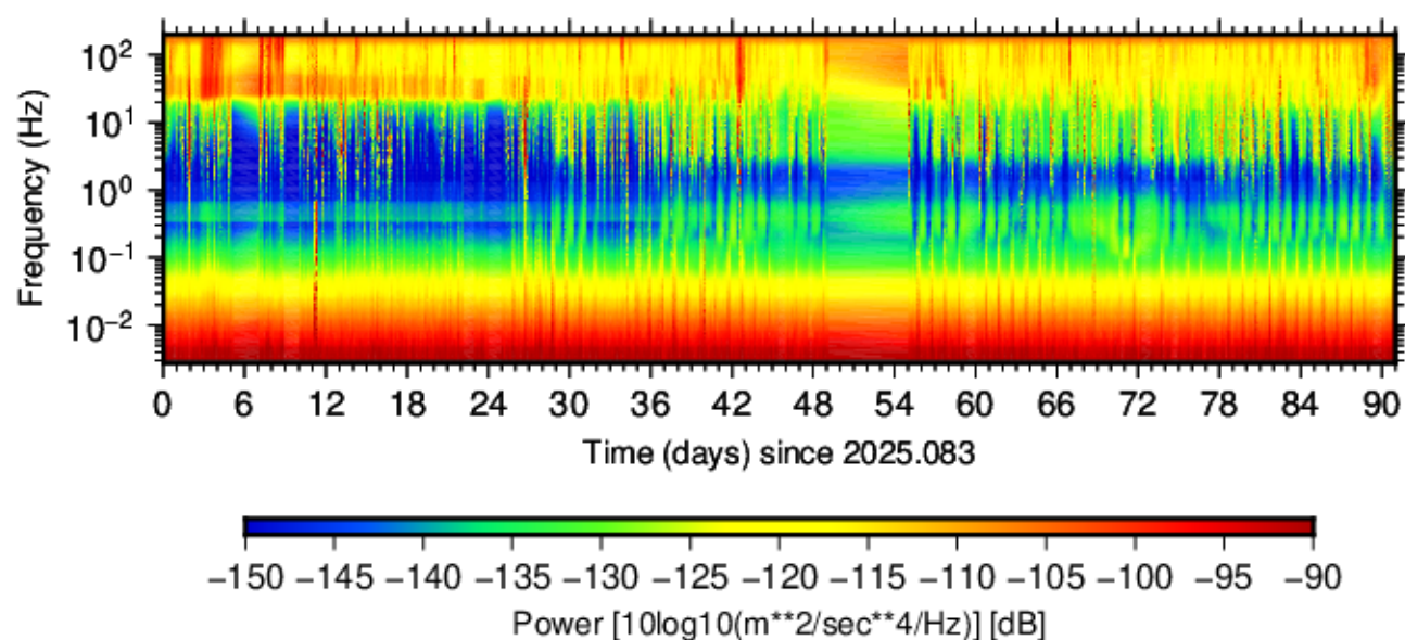
BG.AL6.DPN. (2025.083 - 2025.173)
