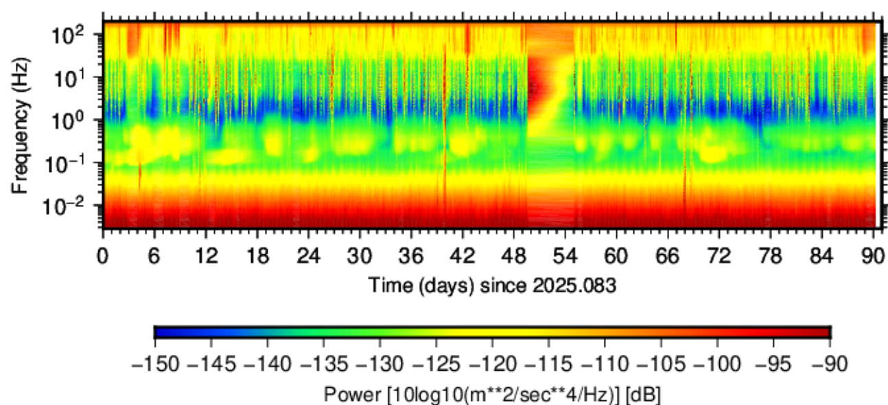
BG.AL6.DPE. (2025.083 - 2025.173)
