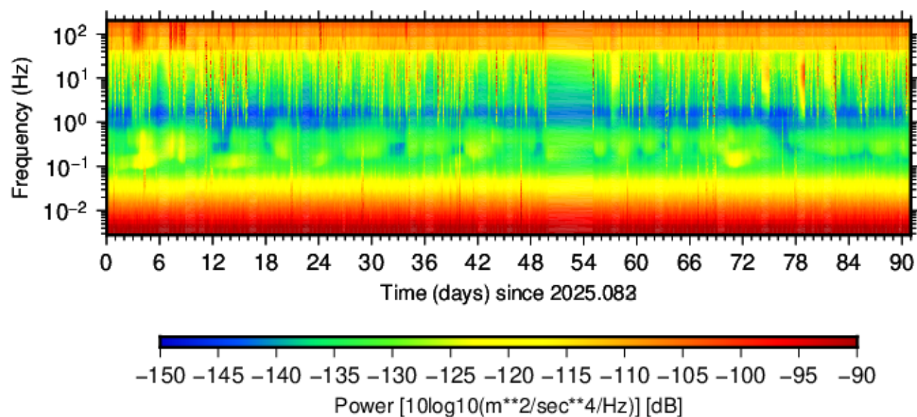
BG.AL6.DPZ. (2025.083 - 2025.173)
